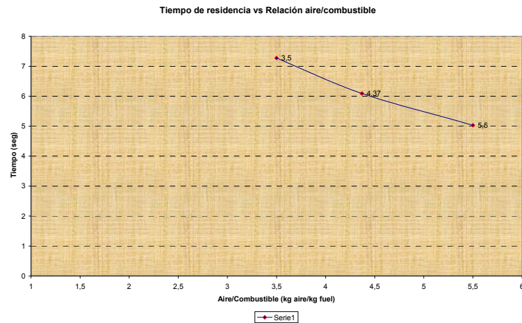
FIGURA 5.2 GRÁFICA TIEMPO DE RESIDENCIA VS RELACIÓN AIRE/COMBUSTIBLE.
