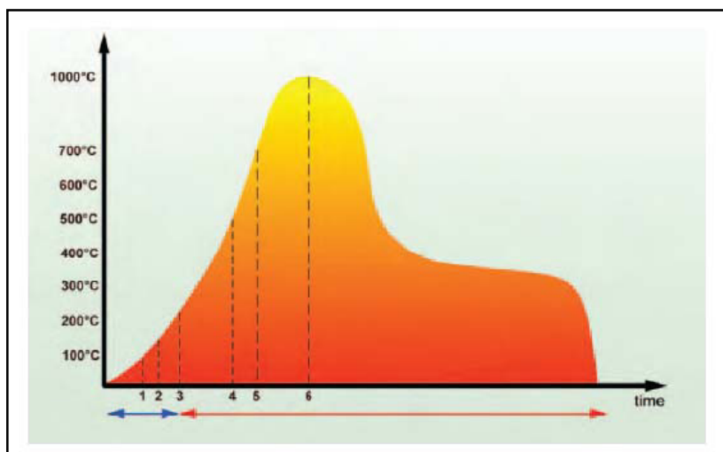
FIGURA 2.11 TEMPERATURA VS TIEMPO DE QUEMA DE LA MADERA.
