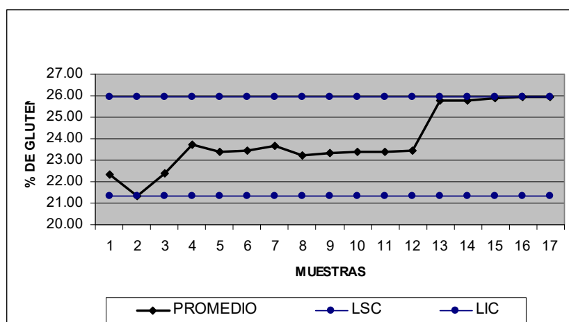
FIGURA 3.4. GRÁFICO DE CONTROL DEL PORCENTAJE DE GLUTEN
