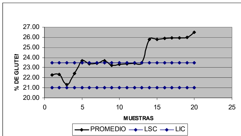
FIGURA 3.2. GRÁFICO COMPARATIVO DEL PORCENTAJE DE GLUTEN
