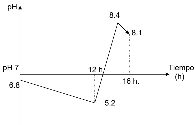
FIGURA 2.1. CURVA DE FERMENTACIÓN DE MASAS CRACKERS.
