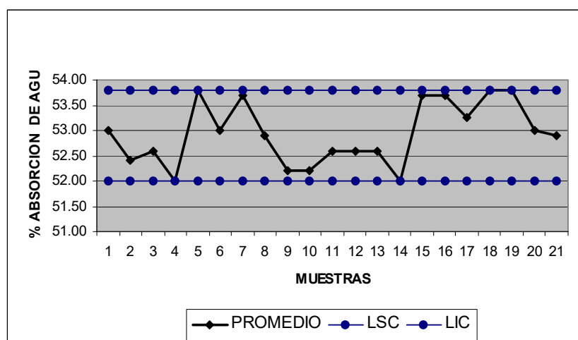
FIGURA 3.5. GRÁFICO DE CONTROL DEL PORCENTAJE DE ABSORCIÓN DE AGUA
