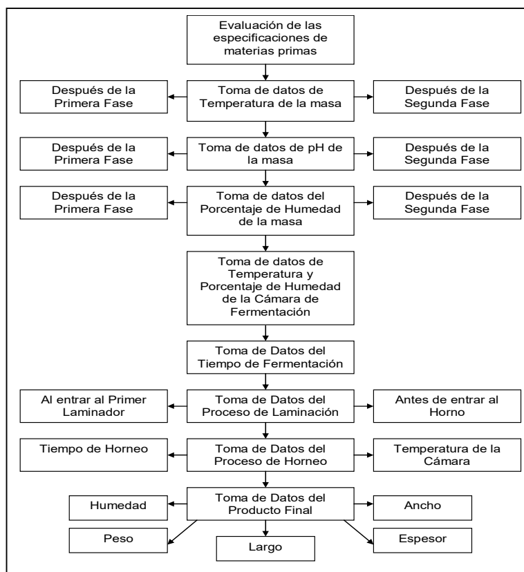
FIGURA 2.2 DIAGRAMA DE FLUJO DE TOMA DE DATOS
