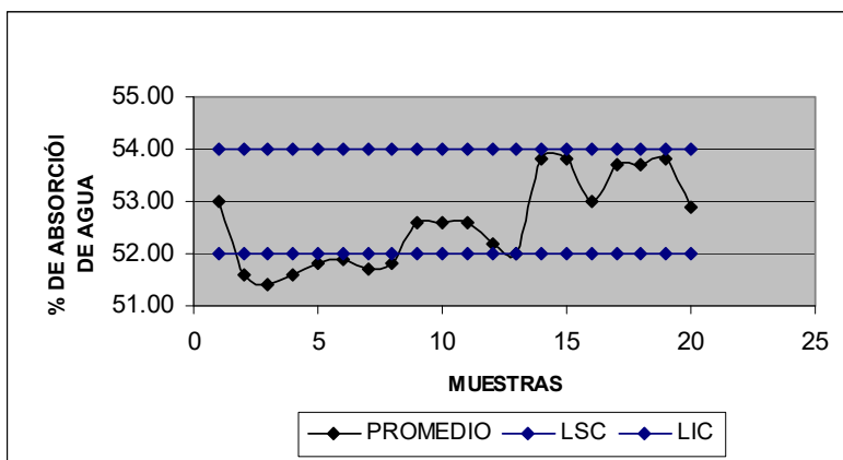
FIGURA 3.3. GRÁFICO COMPARATIVO DEL PORCENTAJE DE ABSORCIÓN DE AGUA
