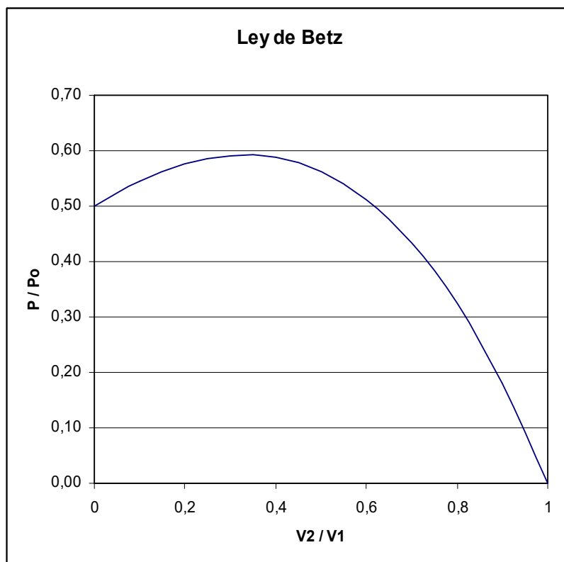
FIGURA 1.2. FRENADO IDEAL DEL VIENTO (LEY DE BETZ)
