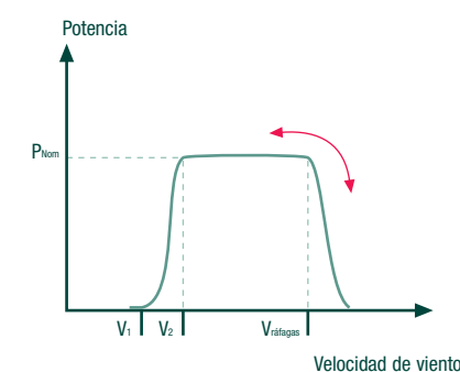
Curva de potencia de un aerogenerador ENERCON con sistema de control de ráfagas – El aerogenerador reduce la potencia sin llegar a desconectarse cuando alcanza una velocidad determinada
