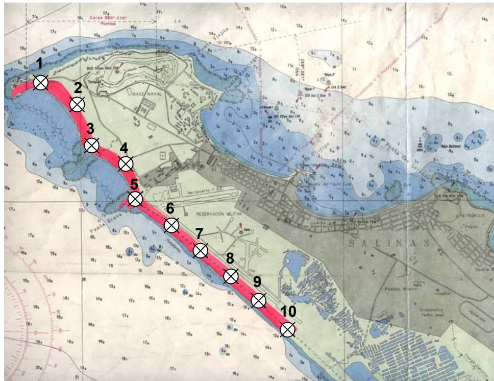
FIGURA 3.8. ARREGLO DEL PARQUE EÓLICO
