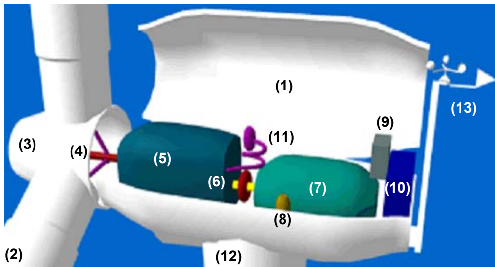
FIGURA 1.3. PARTES DE UNA TURBINA EÓLICA
