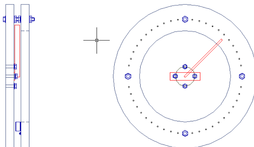
FIGURA 3.8. TAMBOR ROTATORIO.
