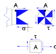
FIGURA 3.17. ANÁLISIS DE ESFUERZOS EN EXTREMO DE ÁRBOL
