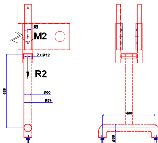
FIGURA 4.4. DIAGRAMA DE SOPORTE DE ESTRUCTURA.
