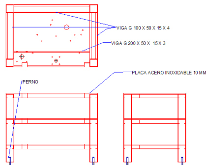
FIGURA 3.48. ESTRUCTURA SOPORTE DE MESA.
