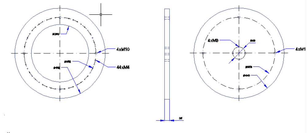
FIGURA 3.13. DATOS SOBRE DISCOS DE TAMBOR.
