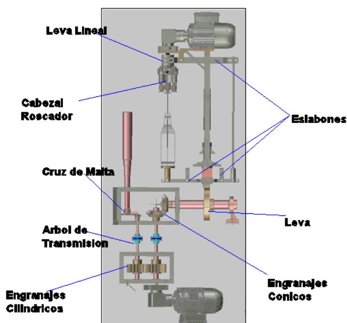
FIGURA 3.41. PARTES PRINCIPALES DEL SISTEMA CENTRAL DE LA MAQUINA.
