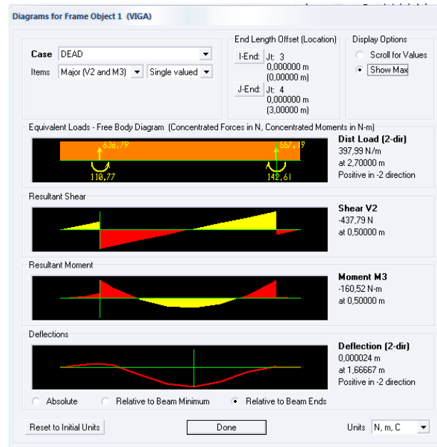
FIGURA 4.3. DIAGRAMAS DE FUERZA CORTANTE, MOMENTO FLECTOR Y DESPLAZAMIENTO DE VIGA PRINCIPAL.
