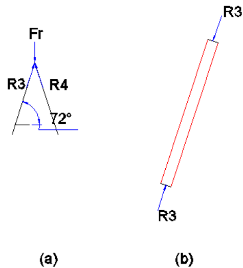
FIGURA 3.20. DIAGRAMA DE FUERZAS SOBRE COLUMNA.
