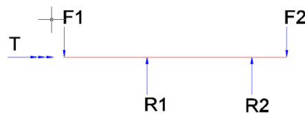
FIGURA 3.15. FUERZAS EN ÁRBOL DE TRANSMISIÓN
