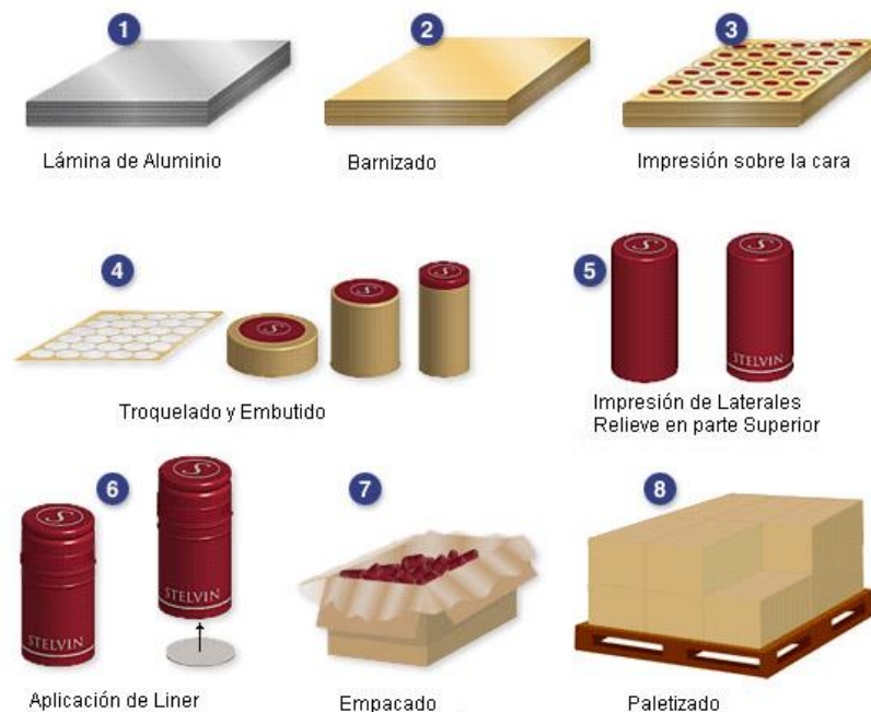
FIGURA 1.2. PASOS DE PRODUCCIÓN DE TAPAS INVIOLABLES.
