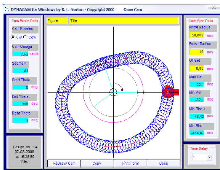
FIGURA 3.38. DISEÑO DE LEVA CON SEGUIDOR DE RODILLO.
