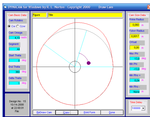
FIGURA 3.39. DISEÑO DE LEVA SECUNDARIA PARA ACCIONAMIENTO DE VÁLVULA NEUMATICA DE RODILLO.
