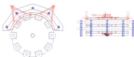
FIGURA 3.6. DIAGRAMA DE FORMA DE JUEGO DE ESTRELLAS.
