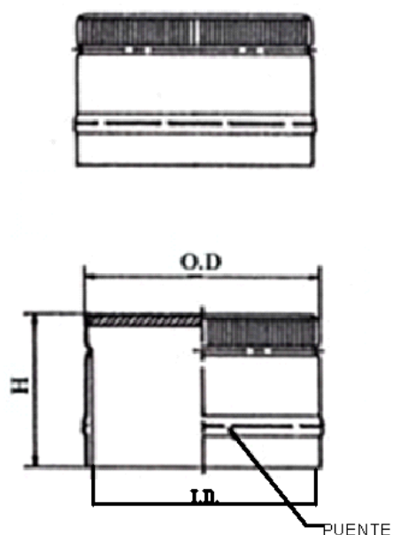
FIGURA 1.5. ESQUEMA DE TAPA INVIOABLES.
