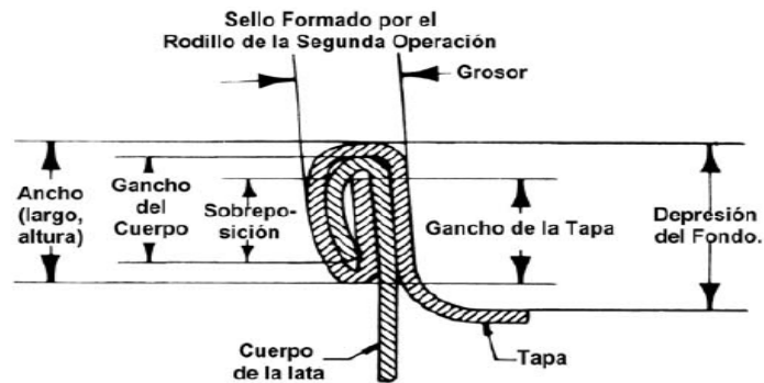
FIGURA 1.3: Segunda operación de formado del doble cierre
