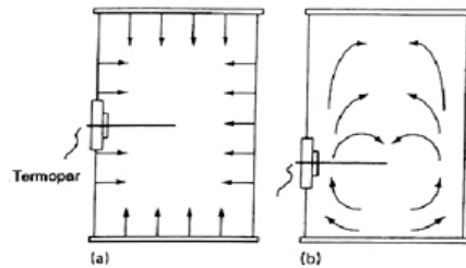
FIGURA1.1 a) Calentamiento por conducción b) Calentamiento por convección
