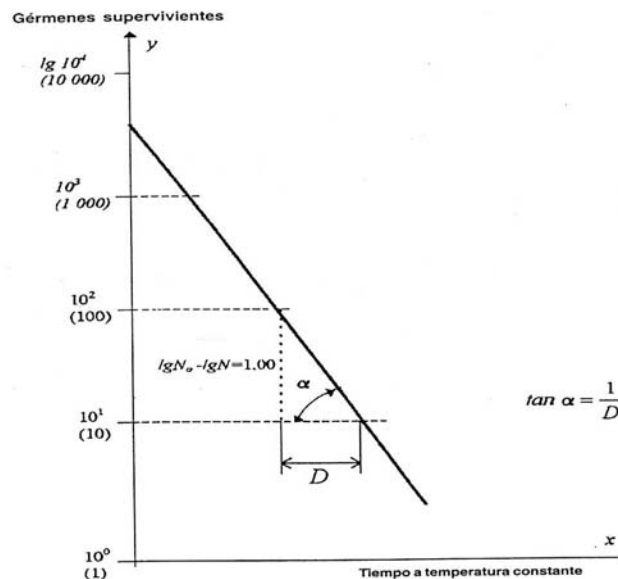
FIGURA 1.4: Curva logarítmica de supervivencia de los gérmenes
