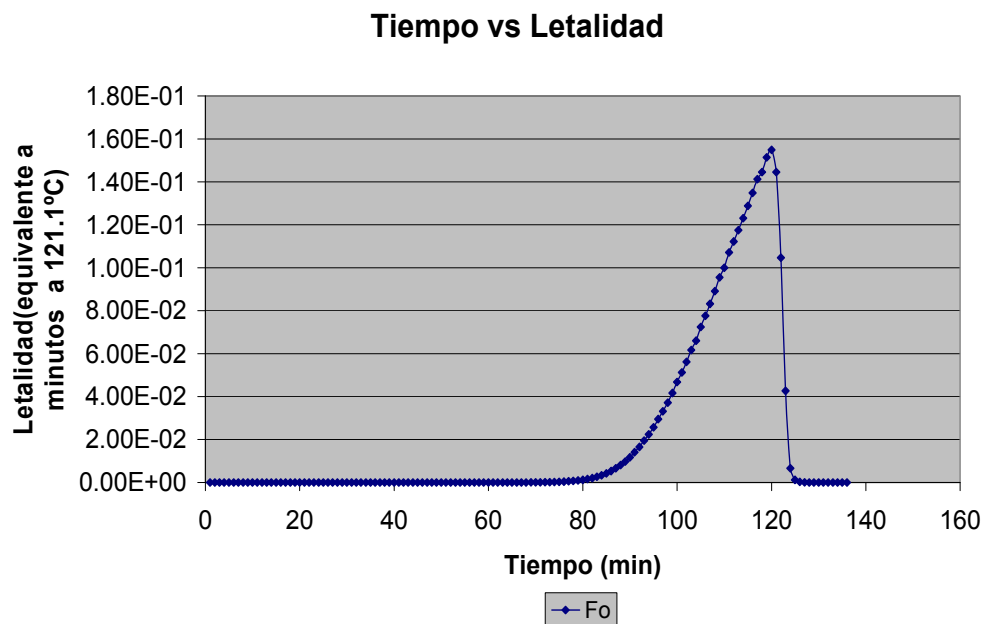
FIGURA 2.4: Letalidad vs tiempo (primer estudio de penetración de calor)
