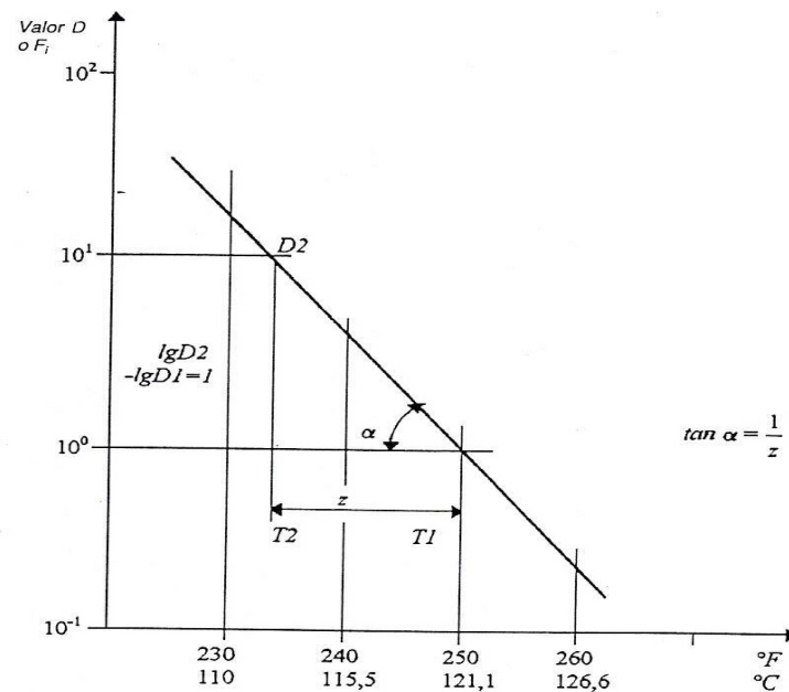
FIGURA 1.5: Curva de los tiempos de destrucción de gérmenes durante 1 minuto a 121.1° c
