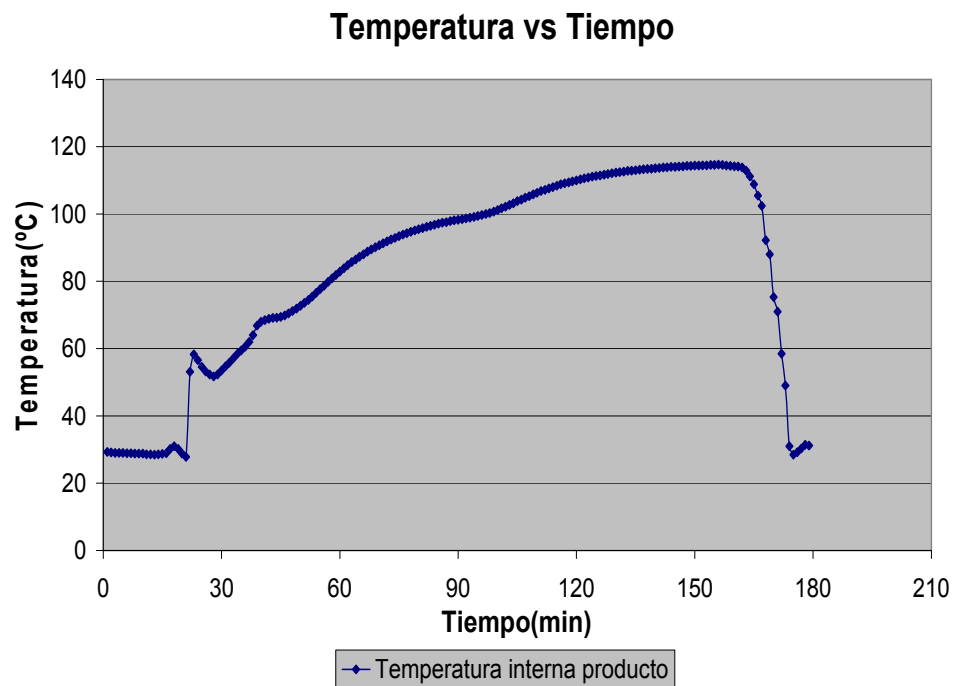
FIGURA 3.17: Temperatura vs. Tiempo, sensor M3P17494
