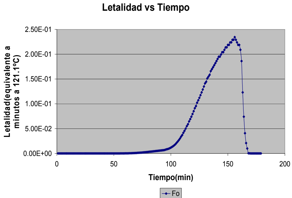
FIGURA 3.20: Letalidad vs. Tiempo, sensor M3P18271
