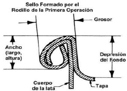
FIGURA 1.2: Primera operación de formado del doble cierre
