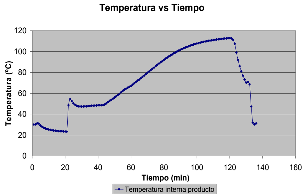
FIGURA2.3 Temperatura vs tiempo (primer estudio de penetración de calor)
