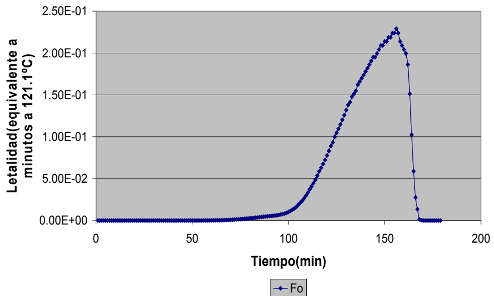
FIGURA 3.18: Letalidad vs. Tiempo, sensor M3P17494
