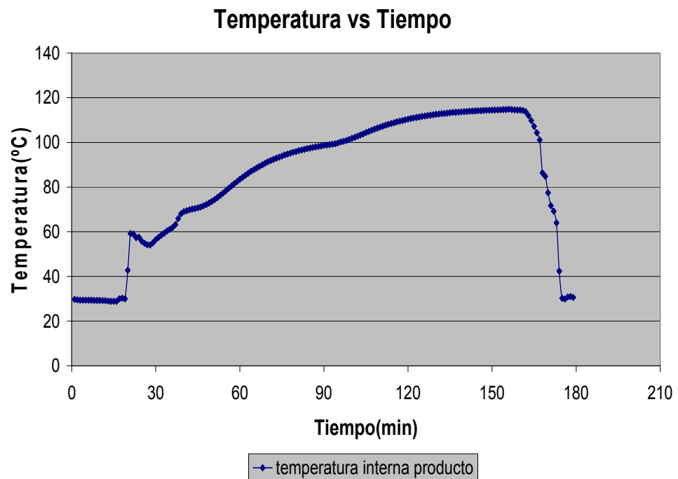
FIGURA 3.19: Temperatura vs. Tiempo, sensor M3P18271
