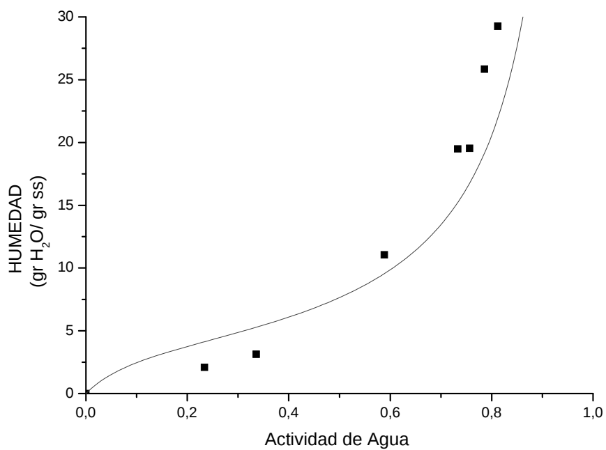
FIGURA 2.2. ISOTERMA DE DESORCIÓN DE CARNE DE CORVINA FRESCA - MÉTODO GRAVIMÉTRICO
