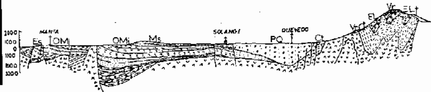
CORTE GEOLOGICO DE LA COSTA ECUATORIANA TOMADO DE LA PUBLICACION DE FUCHER y SAVOYAT, 1972
