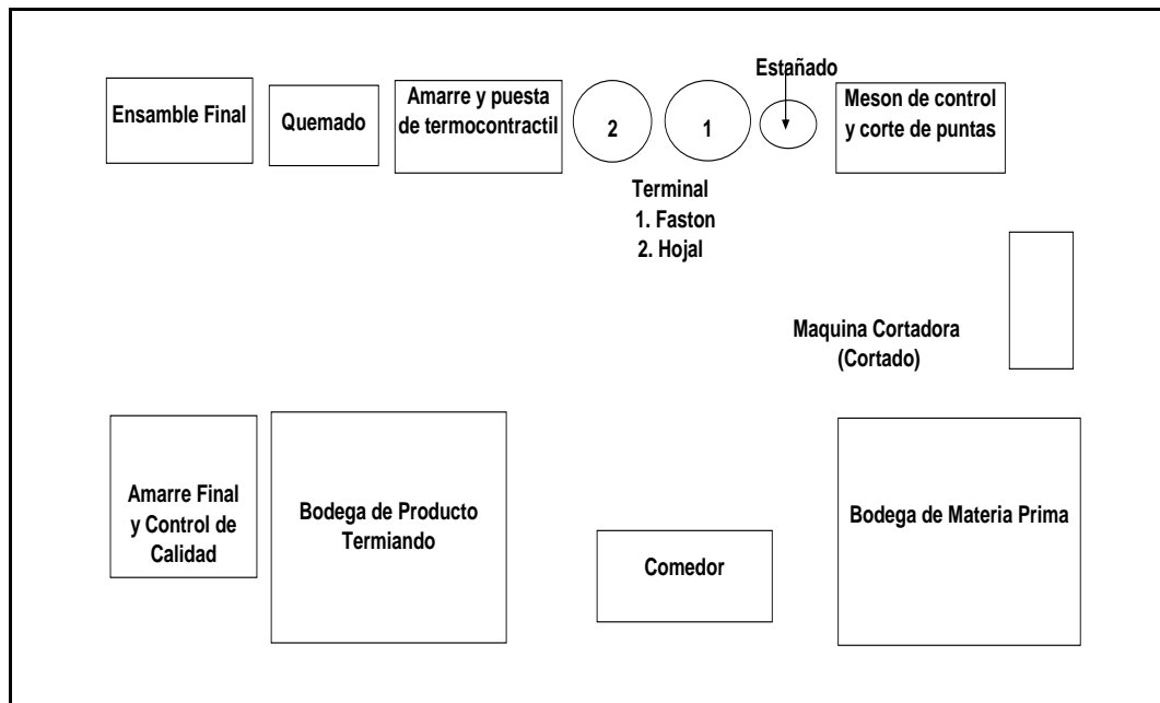
FIGURA 2.1 DISTRIBUCIÓN DE LA PLANTA DE ARNESES ELÉCTRICOS
