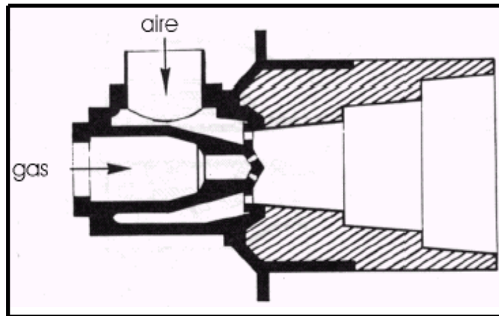
Quemador con abertura lateral escalonada
