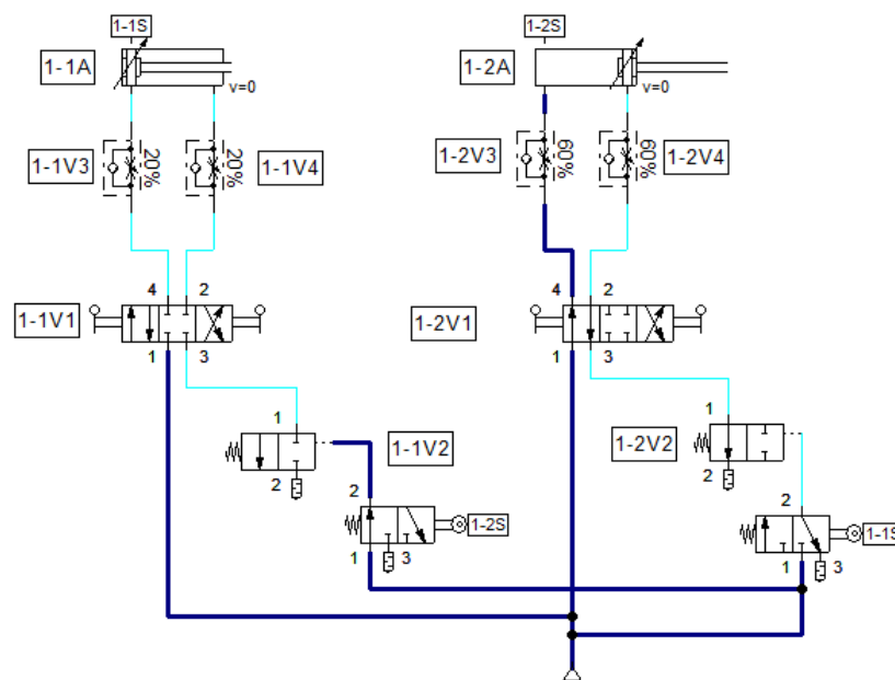
Figura 2.29: Cabezal descendido, marmitta en posición de trabajo
