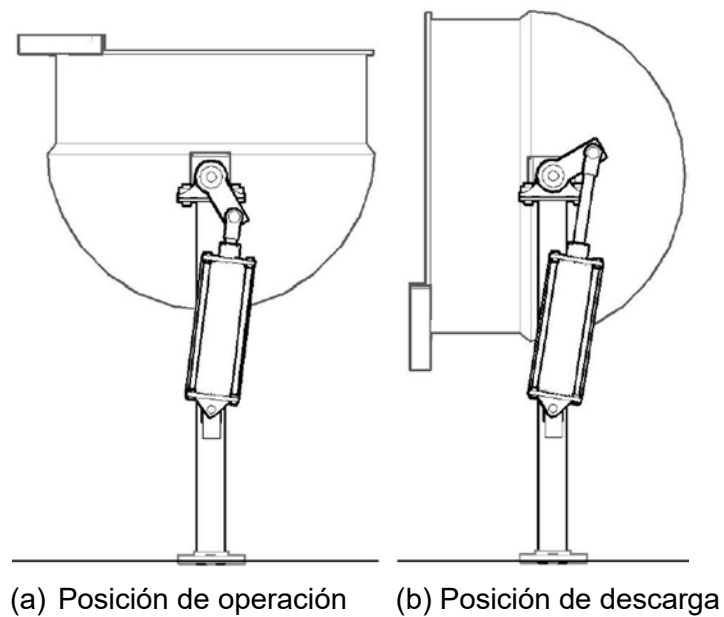
Figura 2.1. Esquema de operación del actuador 1-1A
