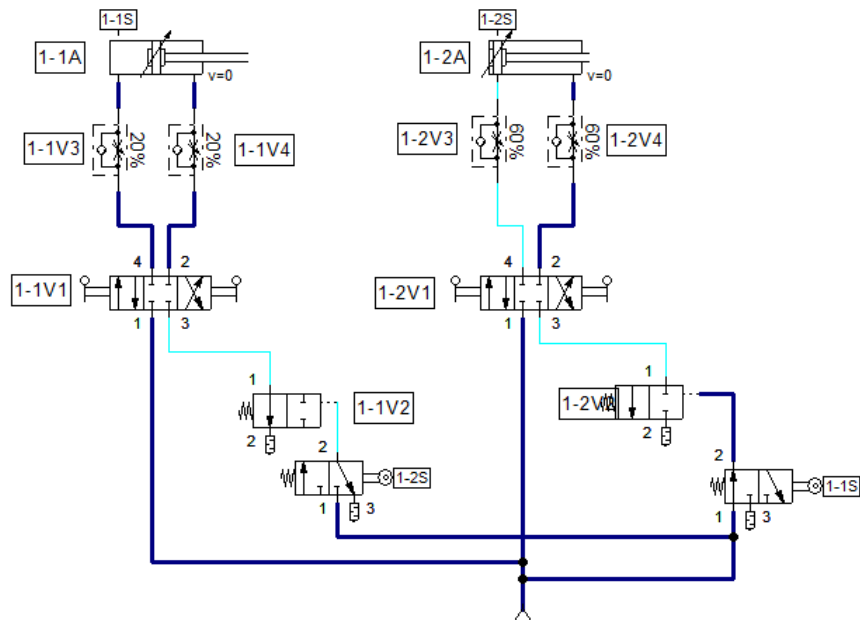
Figura 2.35: Marmita en posición intermedia, cabezal de agitador elevado
