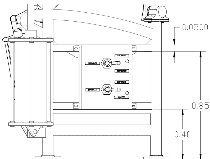
Figura 3.10: Ubicación de platinas de fijación del gabinete
