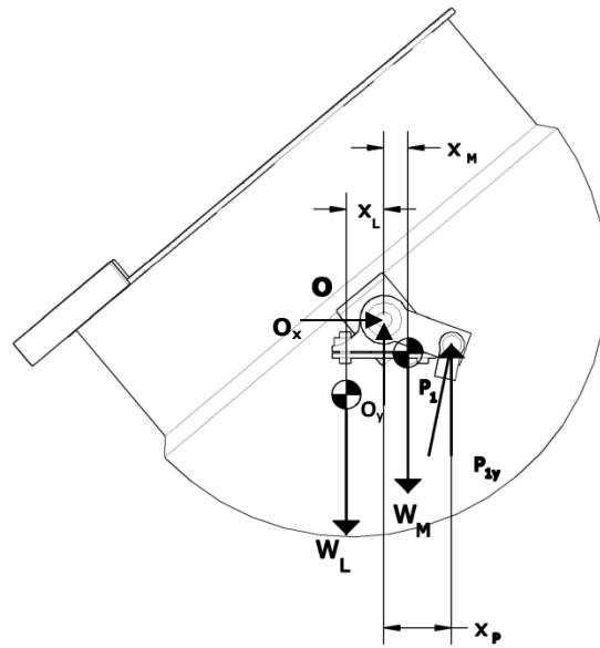
Figura 2.3: Diagrama de cuerpo libre de la marmita y fluido
