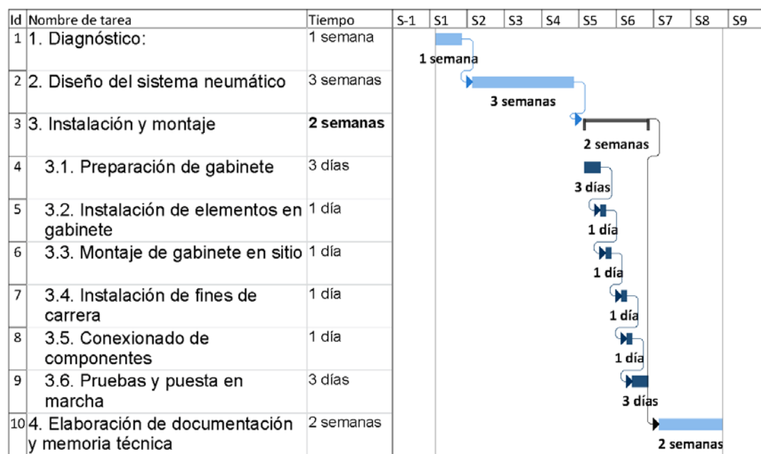
Figura 3.2: Cronograma de repotenciación del sistema neumático de volteo de la marmita y elevación del cabezal agitador
