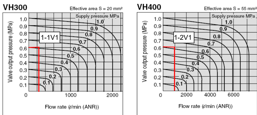
Figura 2.14: Curvas de caudal Serie VH [14]
