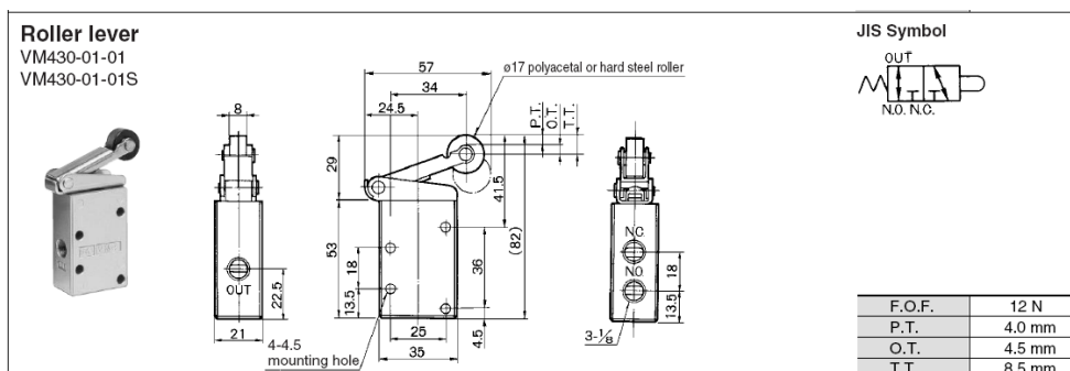
Figura 2.19: Finales de carrera VM430-01-01S [14]
