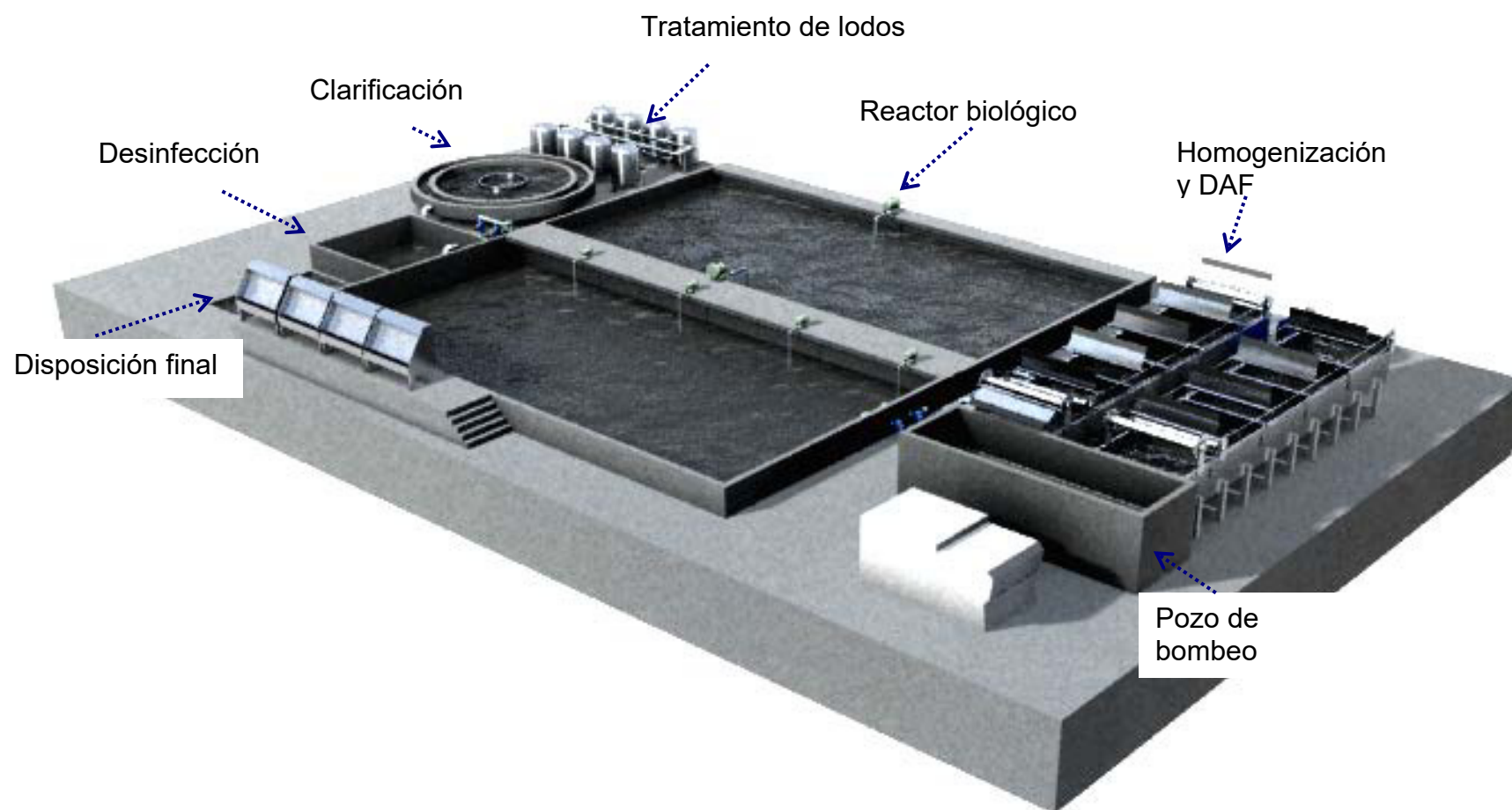
Figura # 3.7.- Esquema de la planta de tratamiento de aguas residuales
