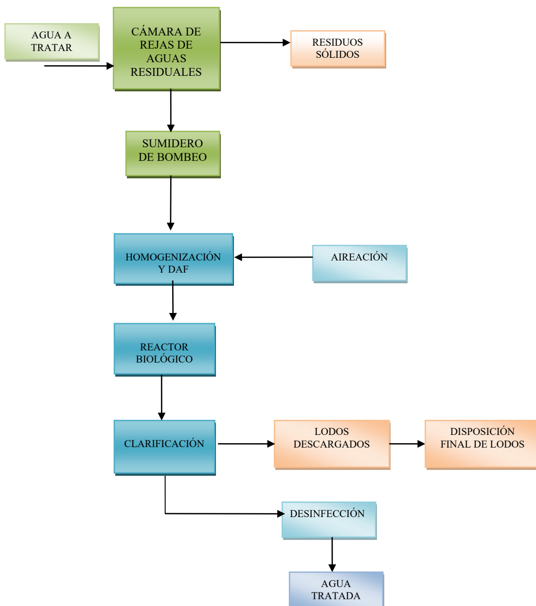
Figura # 3.6.- Diagrama de flujo del tratamiento de aguas residuales
