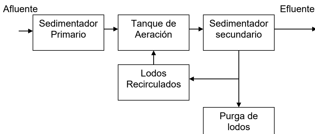
Figura # 3.5.- Esquema del tratamiento biológico
