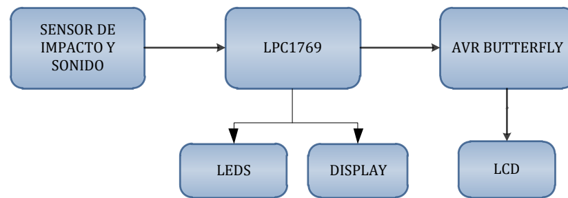
Figura3. 10 Diagrama de Bloques Proyecto
