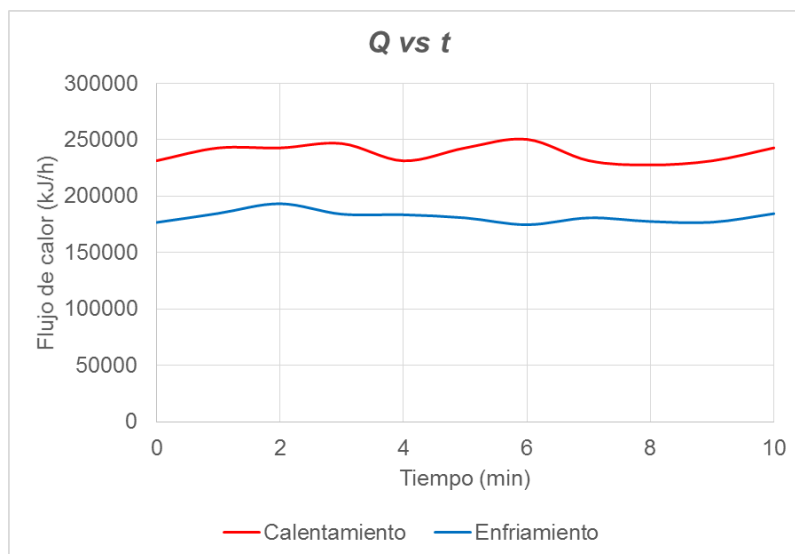
Gráfico 26. PRUEBA 3: Transferencia de calor.
