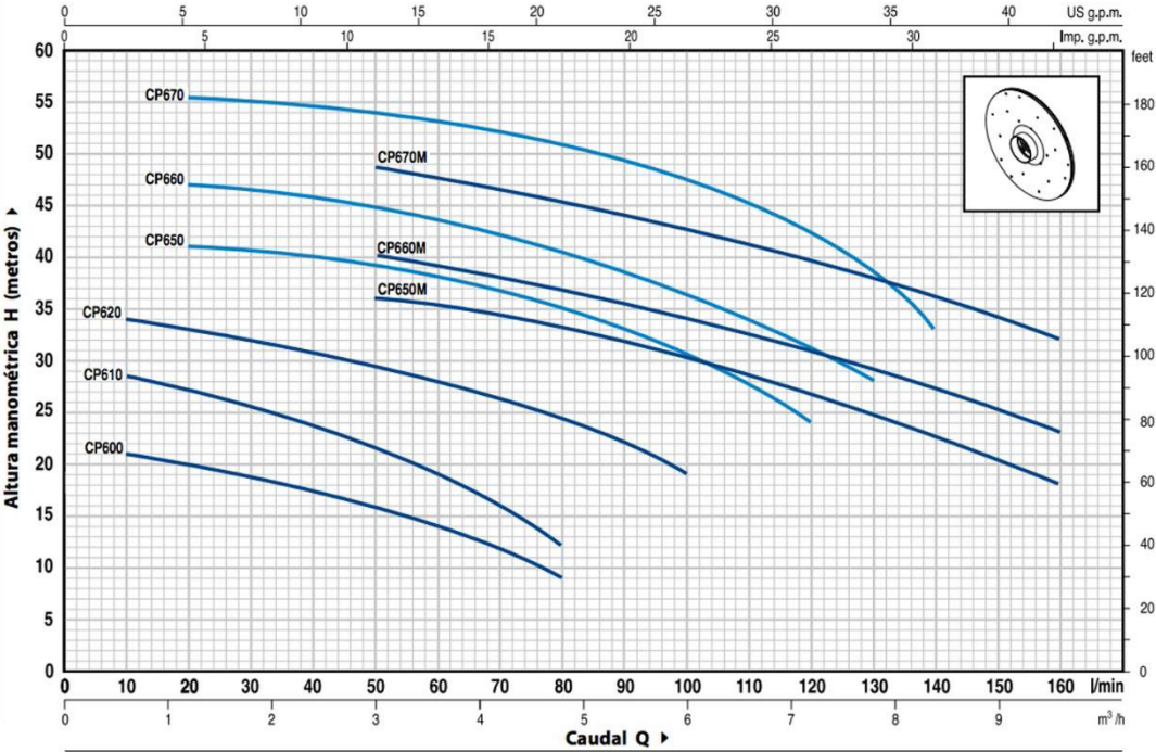
CURVAS Y DATOS DE PRESTACIONES 60 Hz n= 3450 1/min HS= 0 m
