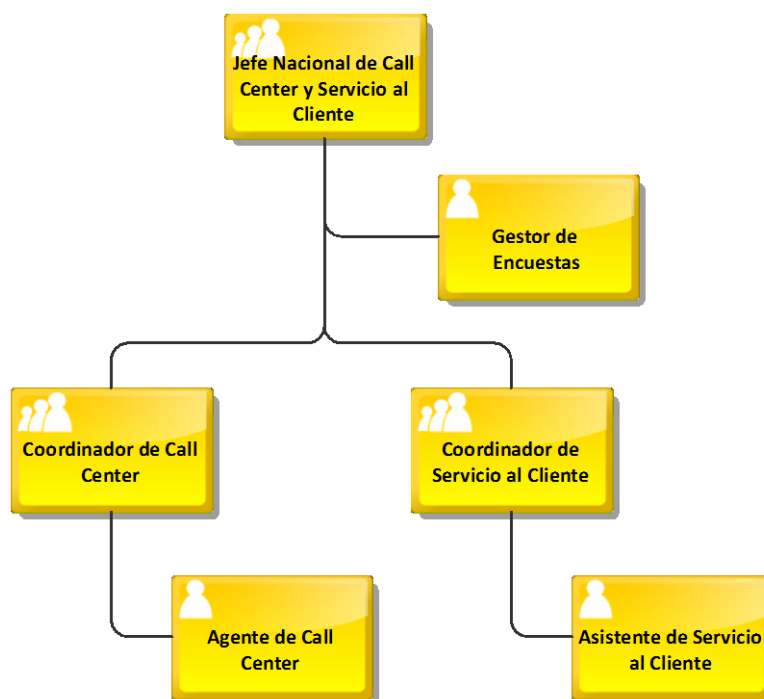
FIGURA N° 10: ORGANIGRAMA DEPARTAMENTAL
