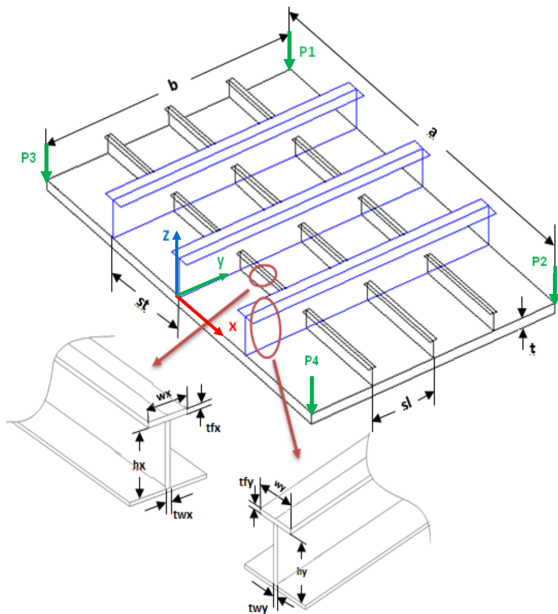
Figura 6: Representación de las variables utilizadas para definir las características geométricas de una plancha reforzada.
