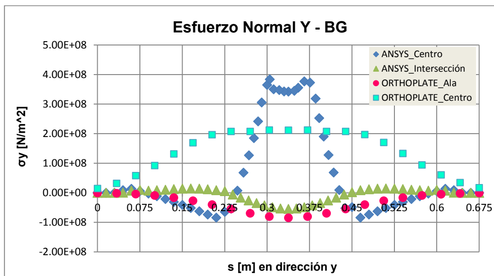
Figura 42: Distribución de \sigma_y a lo largo de distintas posiciones del panel.
