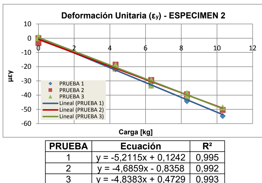
Figura I 5: Microdeformación unitaria \epsilon_y por acción de peso de: 4.32, 6.32, 8.32, 10.32, 8.32, 6.32, 4.32 kg.
