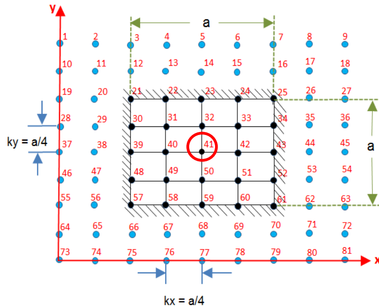
Figura A 1: Discretización del dominio realizada por ORTHO_PLATE .
