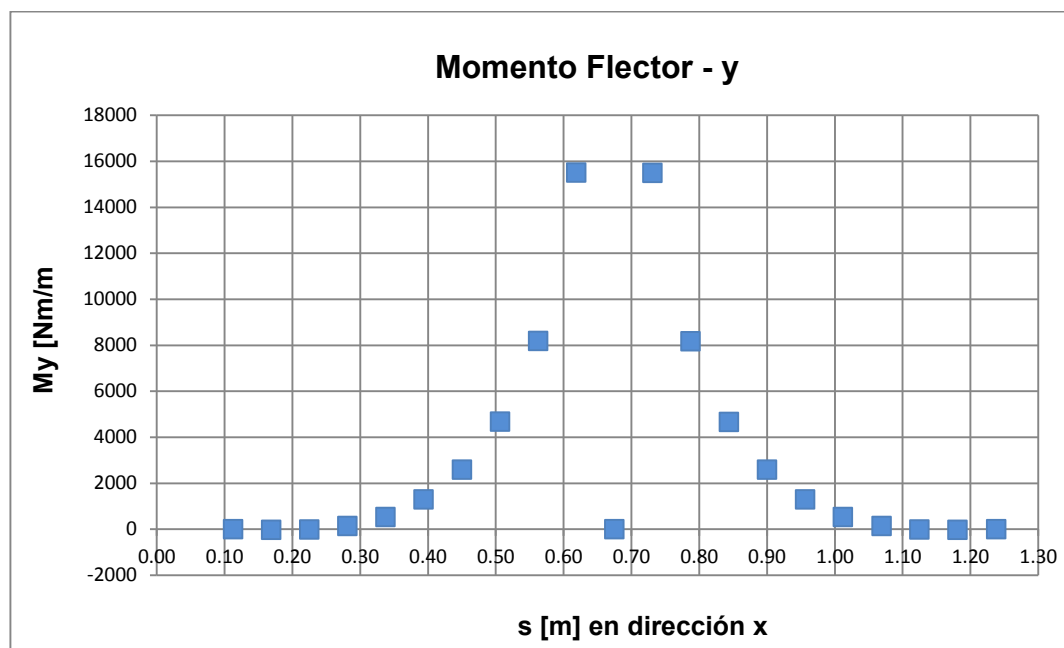
Figura 13: Distribución de momento flector-y del panel a lo largo del nodo central.
