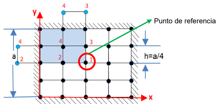
Figura A 2: Discretización del dominio realizada por Ugural, [5].
