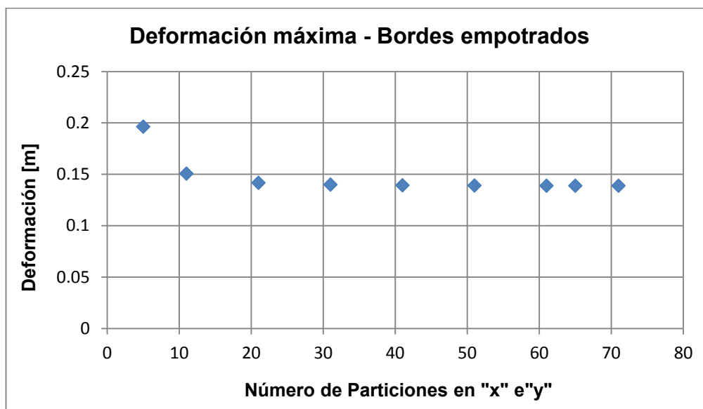
Figura B 1: Convergencia de la solución con ORTHO_PLATE. Ejemplo 1.
