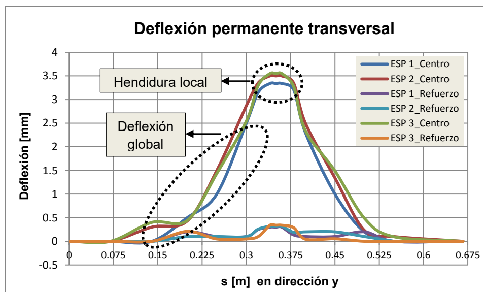
Figura 57: Deflexión residual en el eje y de los 3 especímenes.
