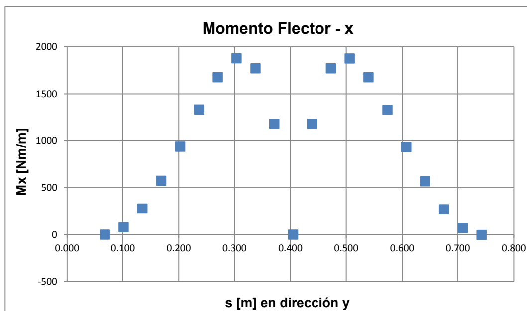
Figura 12: Distribución de momento flector-x del panel a lo largo del nodo central.
