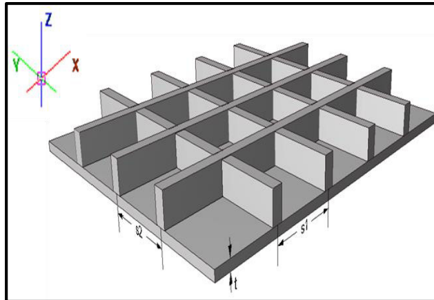
Figura 2: Plancha reforzada en uno de sus lados por refuerzos equidistantes en dos direcciones perpendiculares.
