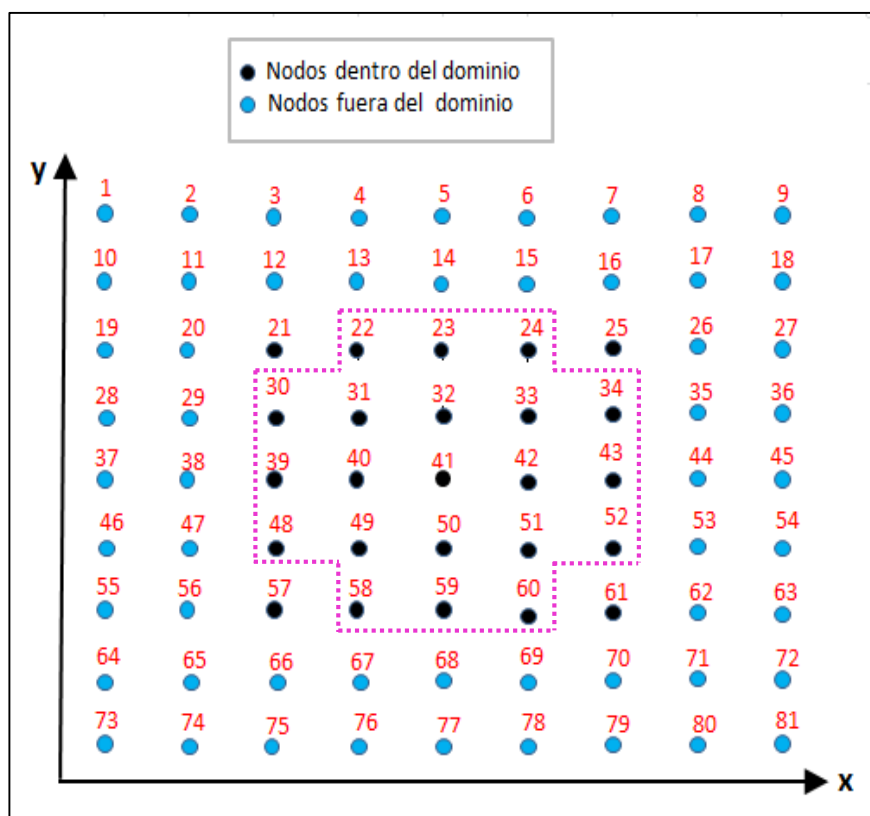
Figura 5: Representación de la discretización del dominio de un panel, (Ejemplo: npx = npy = 5 divisiones en ambas direcciones).
