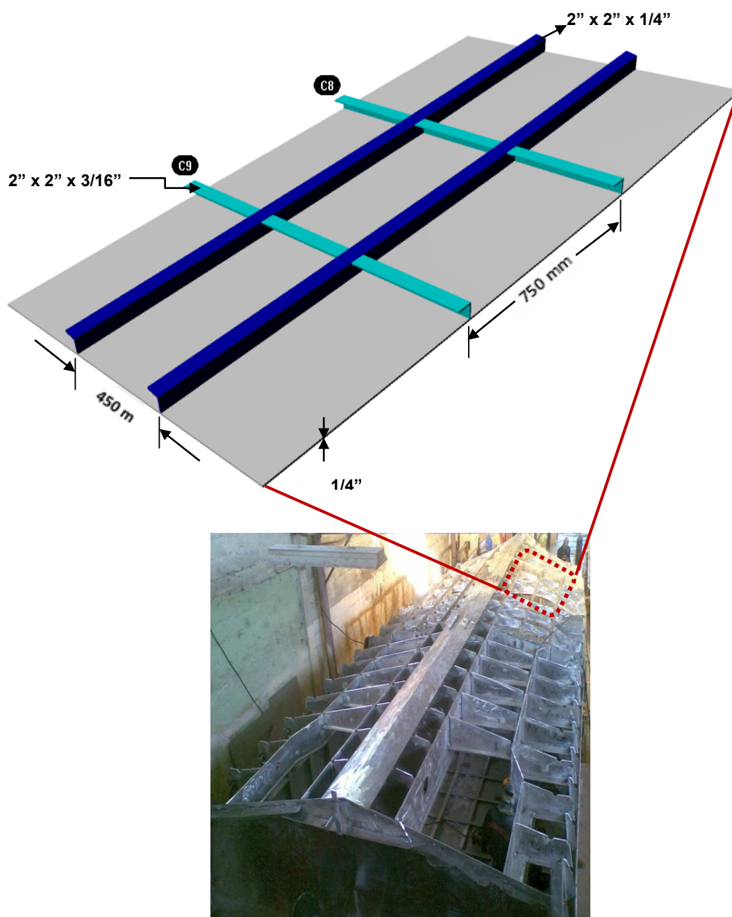
Figura 8: Ubicación del panel seleccionado de la lancha LP-AST-1304, [10].
