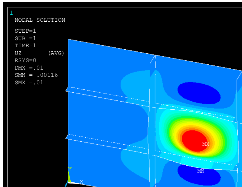
Figura 35: Panel deformado en el sistema de coordenadas global, con asignación de desplazamientos 1 y 2.
