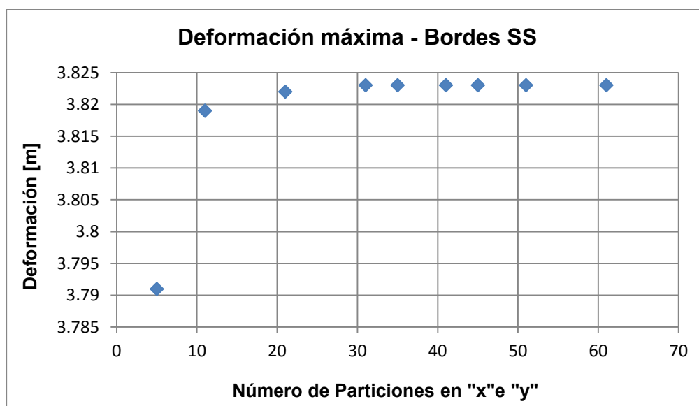
Figura B 2: Convergencia de la solución con ORTHO_PLATE. Ejemplo 2.
