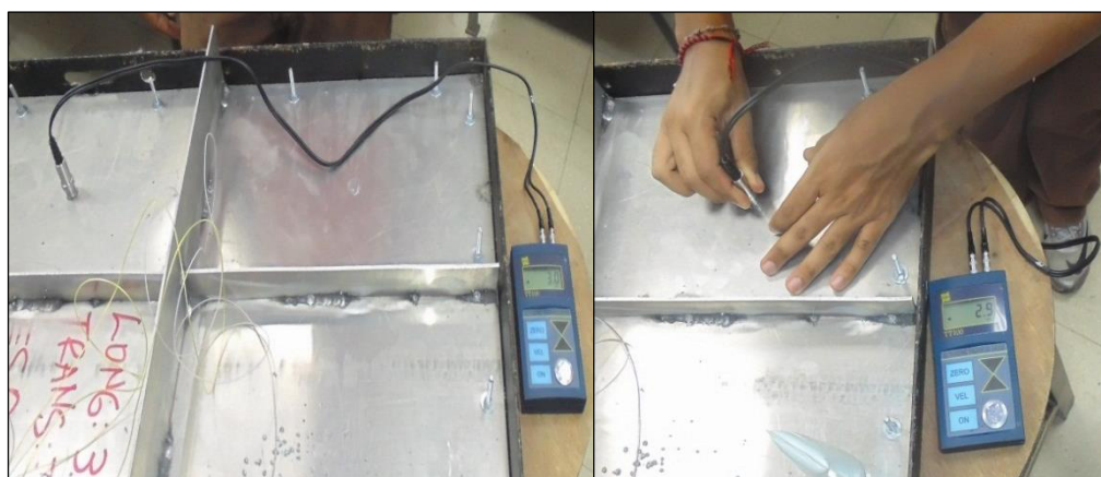
Figura 24: Medición de espesores en cada espécimen.
