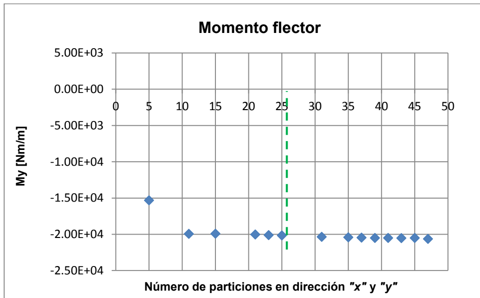
Figura B 3: Análisis de convergencia, a partir del momento flector.
