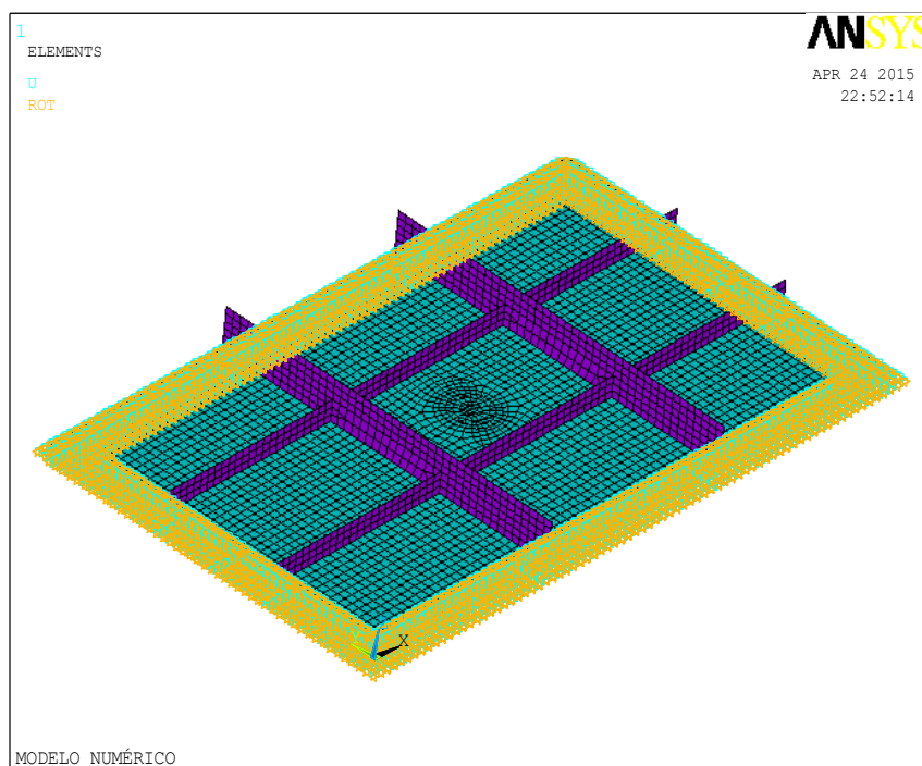
Figura 15: Modelo numérico del panel.
