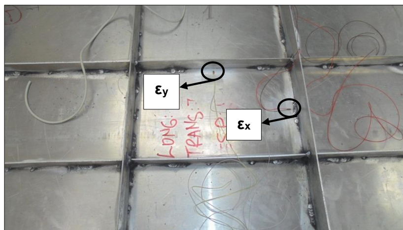
Figura 25: Ubicación y denominación de los extensómetros.
