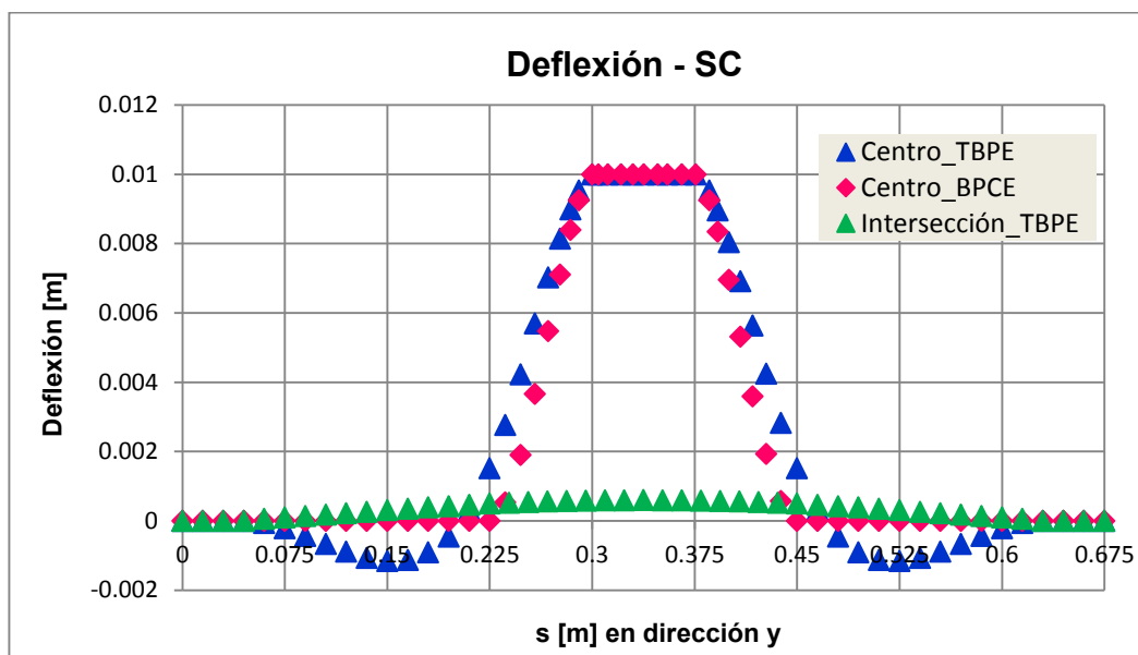
Figura 50: Deflexión en dirección “y”, a lo largo de distintas posiciones del panel. Asignación 2: SC.
