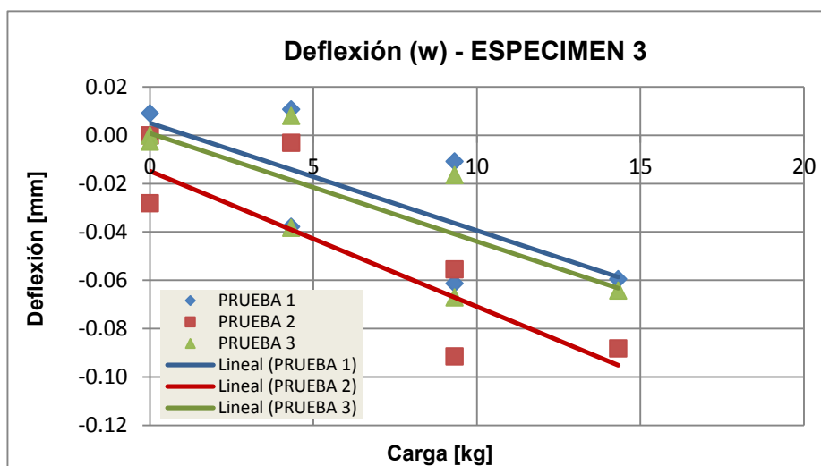
Figura I 8: Microdeformación unitaria \epsilon_y por acción de peso de: 4.32, 9.32, 14.32, 9.32, 4.32 kg.
