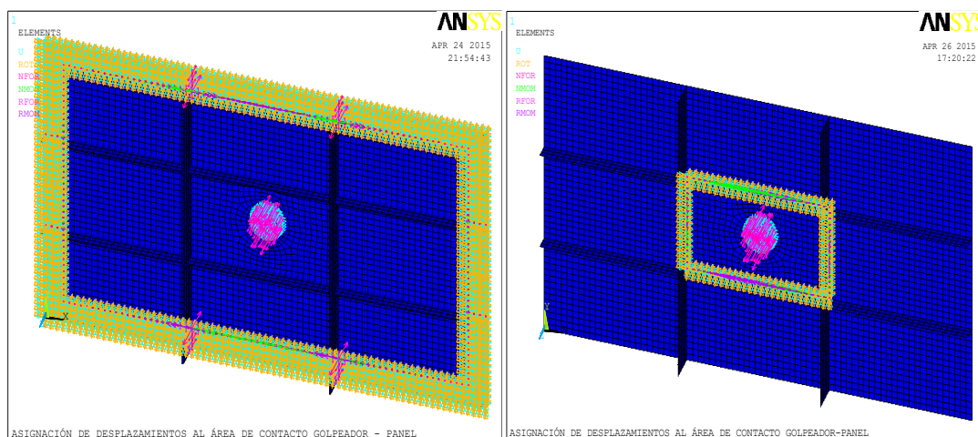
Figura 46: Modelos numéricos, empotrados en sus bordes y en la zona central del panel. Asignación 1 y 2, respectivamente.
