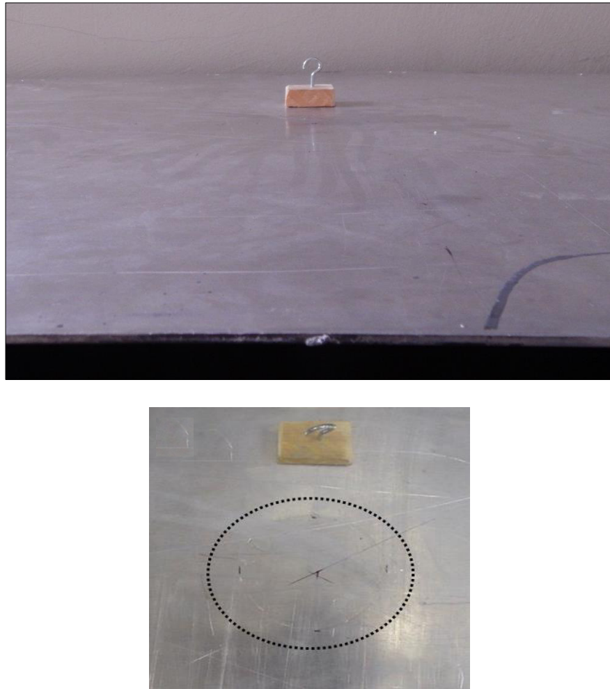
Figura 55: Estado final de los especímenes luego del impacto.
