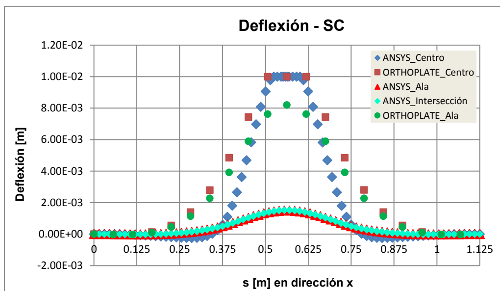
Figura 39: Perfil longitudinal de deflexión, a lo largo de distintas posiciones del panel. Asignación 2: SC
