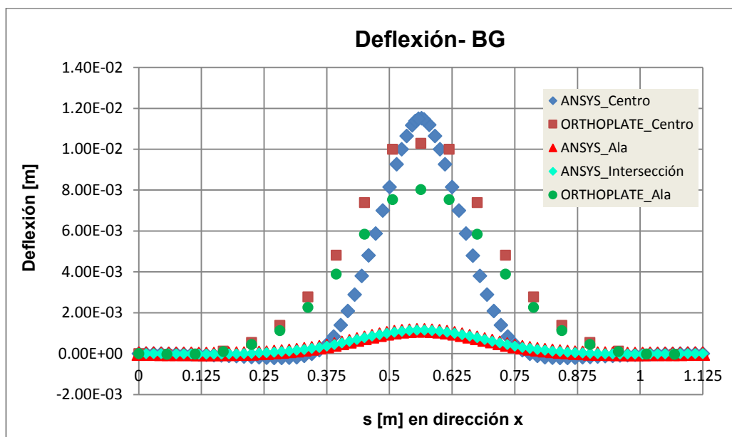
Figura 38: Perfil longitudinal de deflexión, a lo largo de distintas posiciones del panel. Asignación 1: BG.
