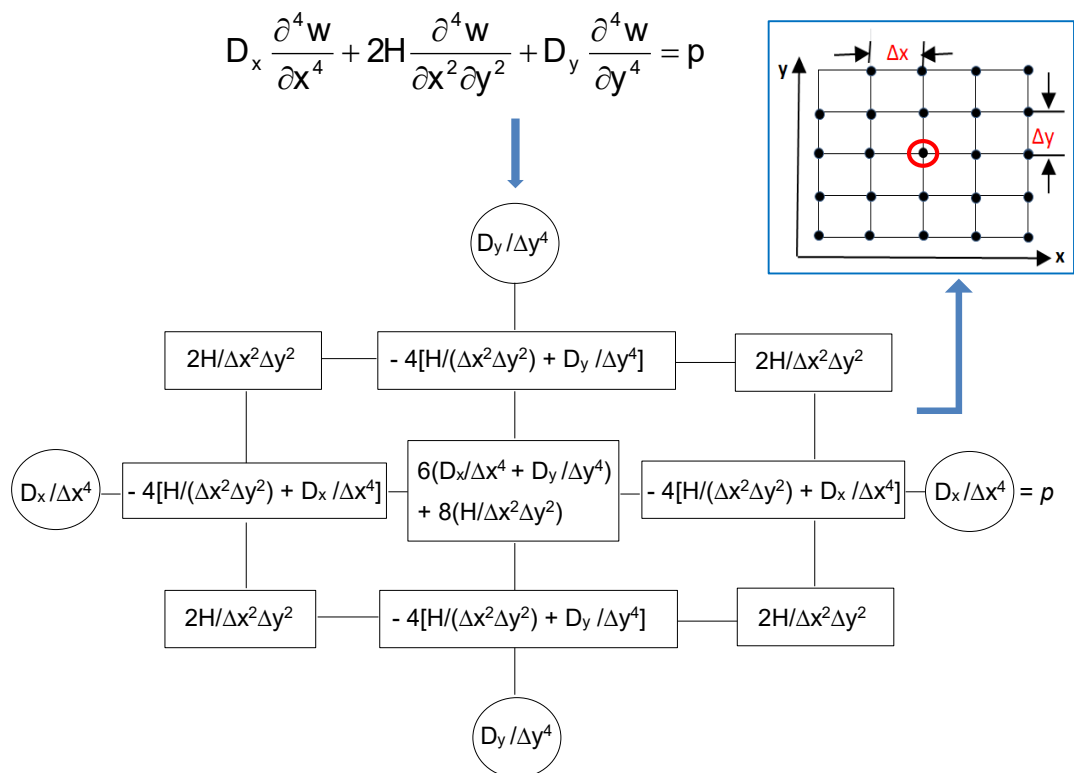
Figura 3: Coeficientes en DF de la ecuación de Planchas Ortotrópicas, [5].
