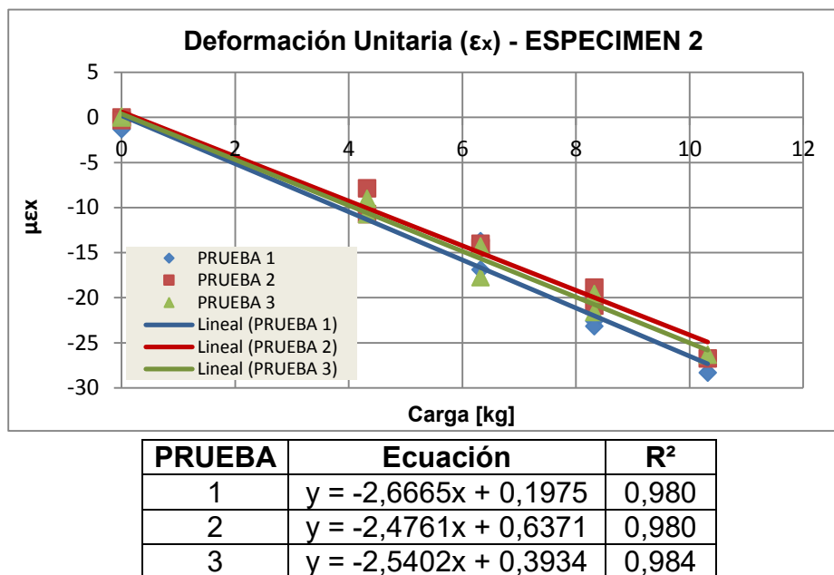
Figura I 4: Microdeformación unitaria \epsilon_x por acción de peso de: 4.32, 6.32, 8.32, 10.32, 8.32, 6.32, 4.32 kg.
