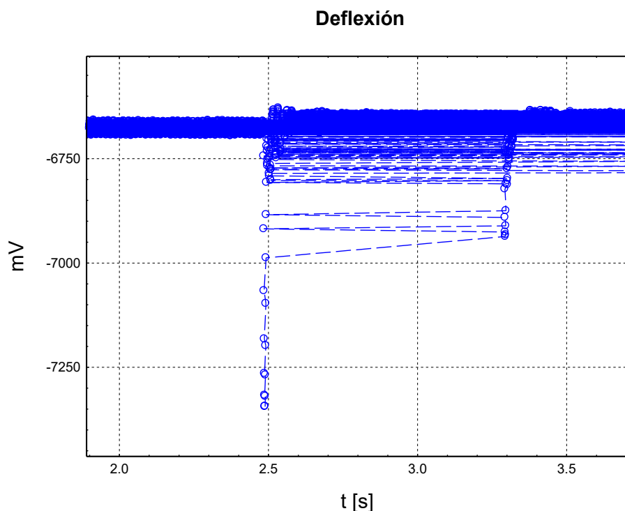
Figura 31: Microdeformaciones unitarias \varepsilon_x , \varepsilon_y , \gamma , deflexión (milivoltios) por impacto de peso de 500 gr desde una altura de 2.00 m.
