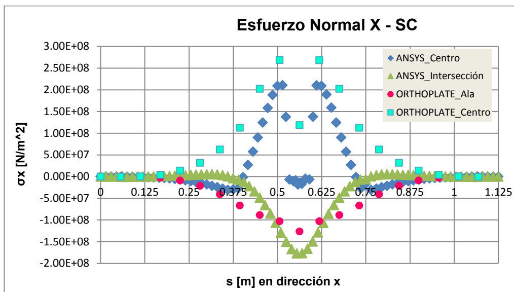
Figura 45: Distribución de \sigma_x a lo largo de distintas posiciones del panel.
