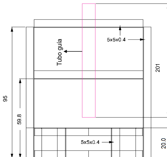
Figura G 1: Plano en centímetros de la base y torre de caída.
