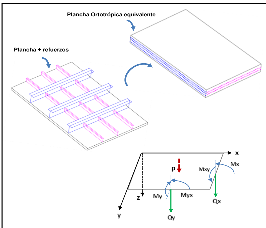
Figura 1: Panel reforzado modelado como Plancha Ortotrópica y convención de signos adoptado para el análisis.
