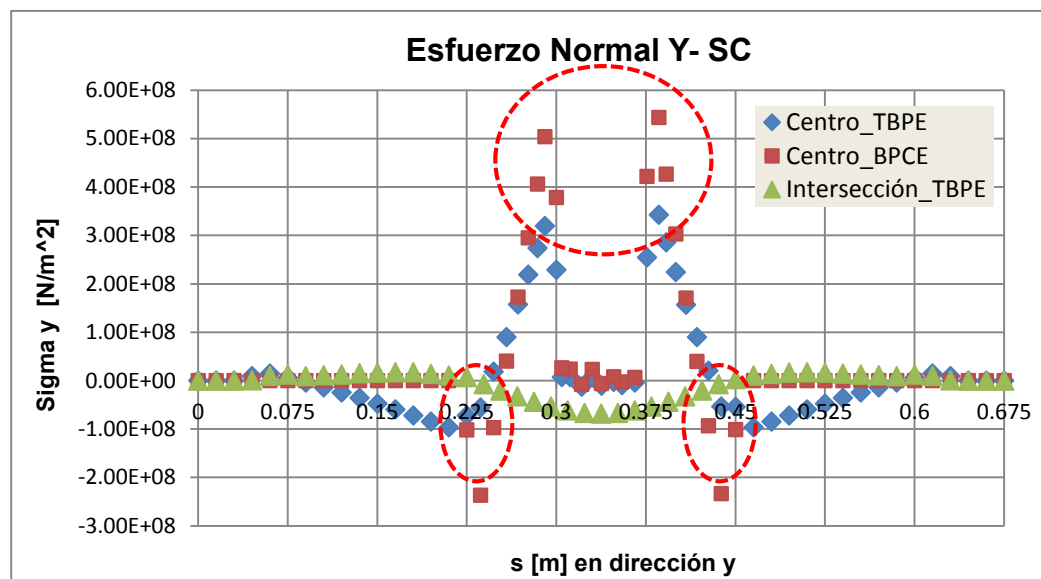
Figura 53: Distribución de \sigma_y a lo largo de distintas posiciones del panel.
