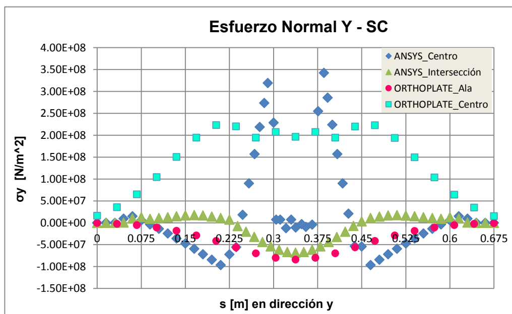
Figura 44: Distribución de \sigma_y a lo largo de distintas posiciones del panel.
