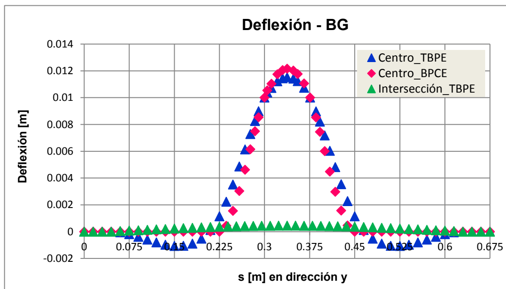
Figura 49: Deflexión en dirección “y”, a lo largo de distintas posiciones del panel. Asignación 1: BG.
