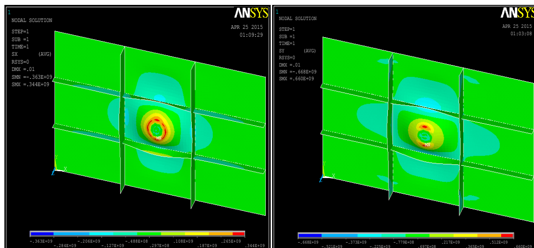
Figura 37: \sigma_x y \sigma_y del panel en el sistema de referencia global. Asignación 2.
