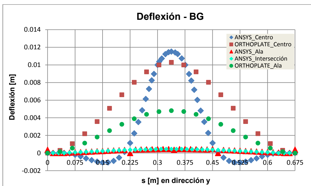
Figura 40: Perfil transversal de deflexión, a lo largo de distintas posiciones del panel. Asignación 1: BG.
