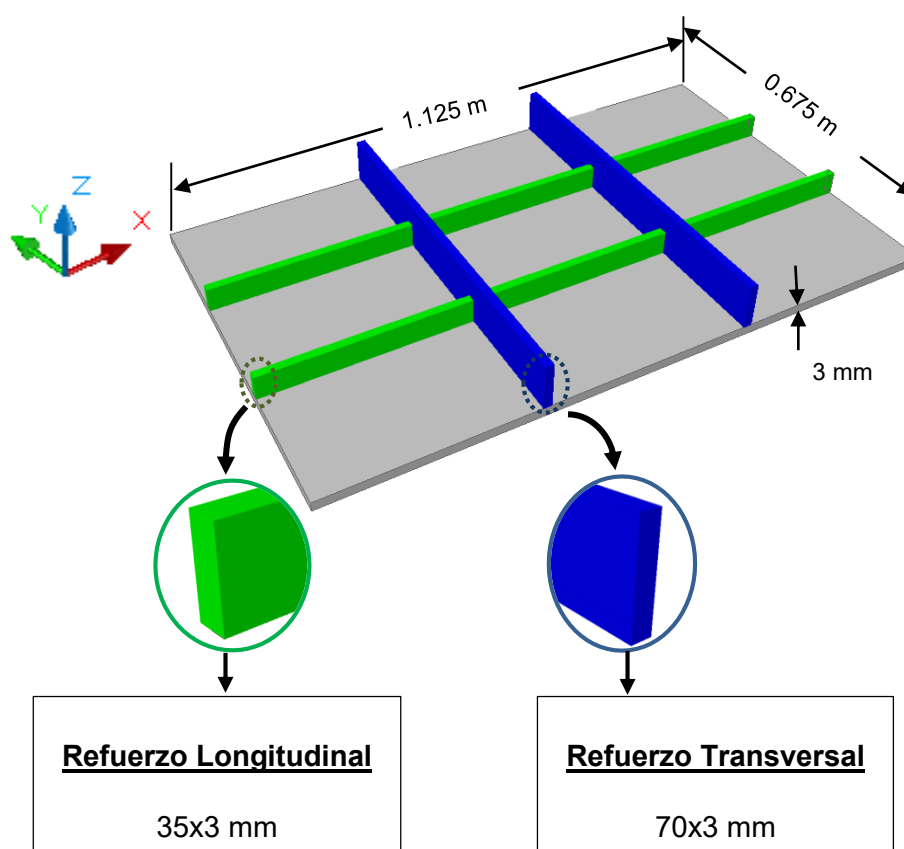
Figura 9: Características geométricas del panel reforzado.
