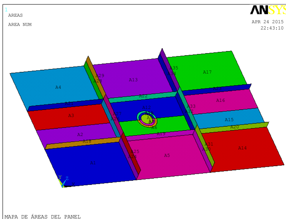
Figura 14: Representación de la geometría del panel en ANSYS.
