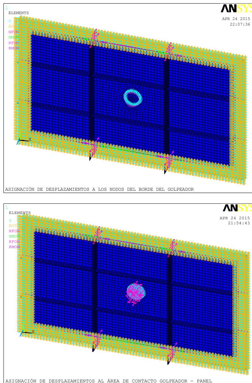
Figura 34: Asignación de desplazamientos específicos con el MEF.
