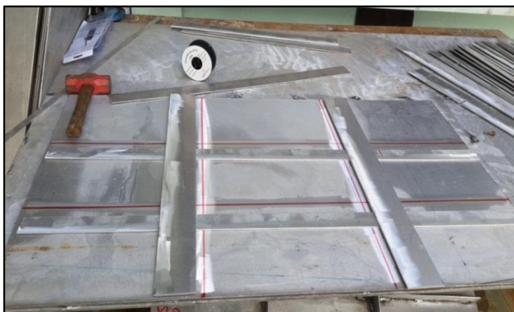
Figura 21: Corte de los segmentos de plancha y refuerzos tipo platina.
