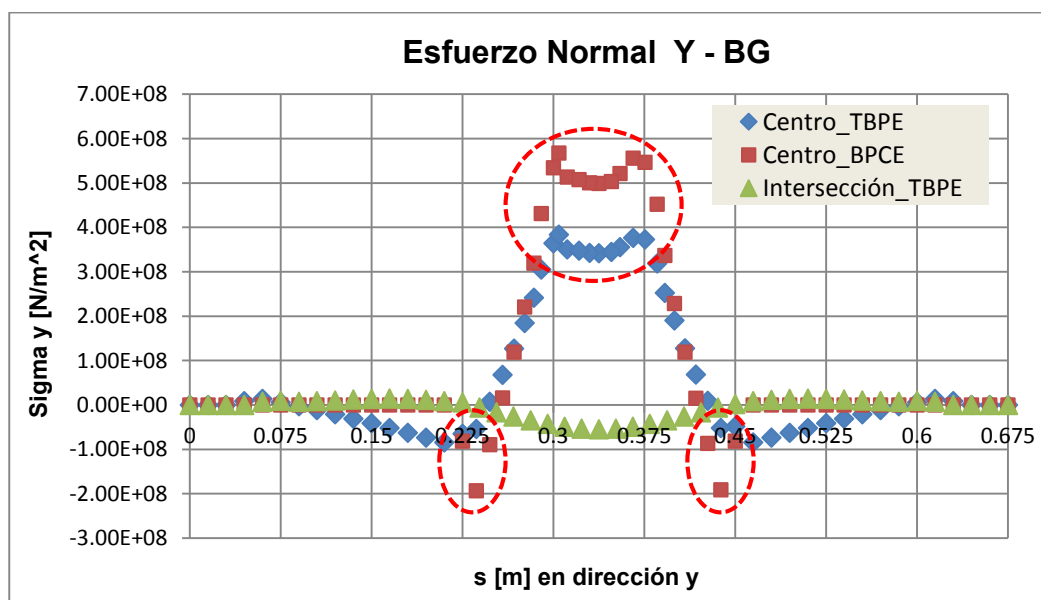
Figura 51: Distribución de \sigma_y a lo largo de distintas posiciones del panel.
