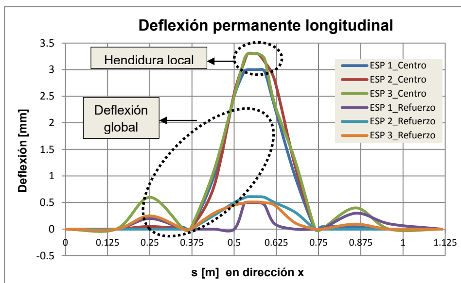
Figura 56: Deflexión residual en el eje x de los 3 especímenes.
