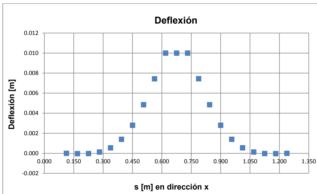
Figura 11: Deflexión vertical (UZ) del panel a lo largo del nodo central.
