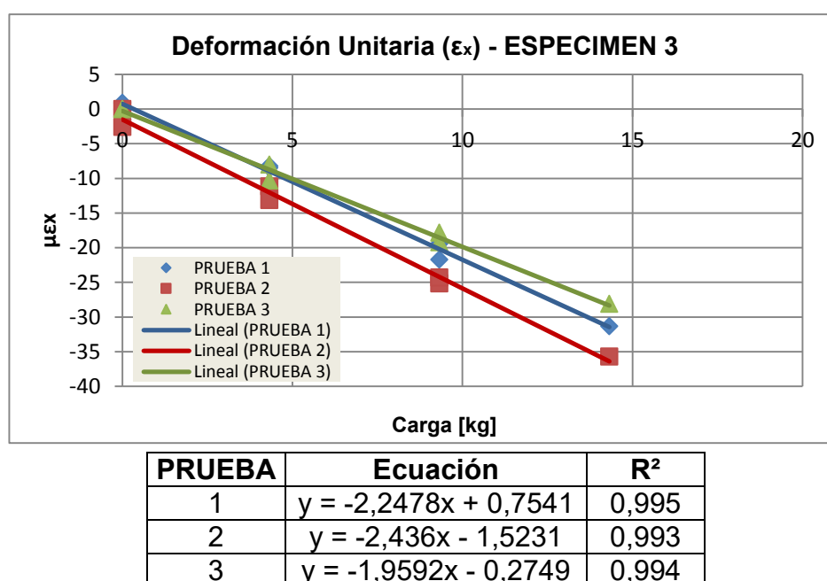
Figura I 7: Microdeformación unitaria \epsilon_x por acción de peso de: 4.32, 9.32, 14.32, 9.32, 4.32 kg.
