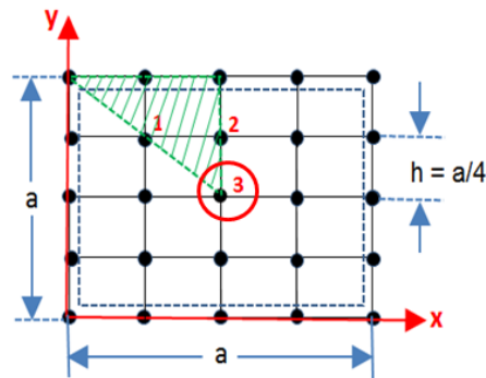
Figura A 3: Discretización del dominio de una placa con todos sus bordes simplemente soportados, [5].
