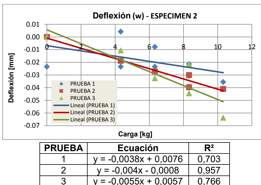
Figura I 6: Deflexión por acción de peso de: 4.32, 6.32, 8.32, 10.32, 8.32, 6.32, 4.32 kg.
