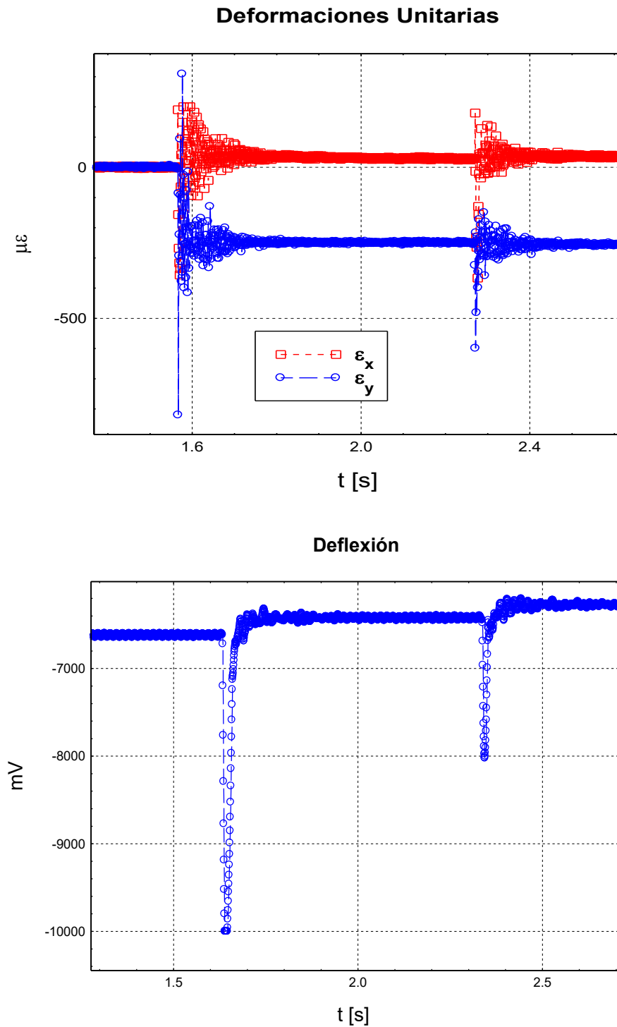
Figura 32: Microdeformaciones unitarias \varepsilon_x , \varepsilon_y , y , deflexión (milivoltios) por impacto del golpeador de 4.32 kg desde una altura de 2.03 m.
