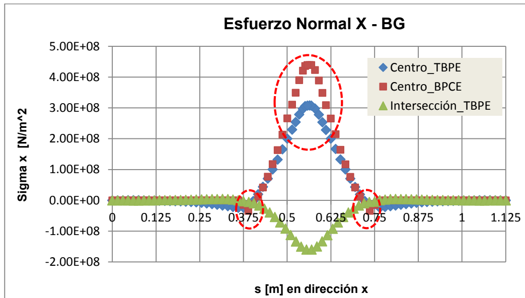
Figura 52: Distribución de \sigma_x a lo largo de distintas posiciones del panel.
