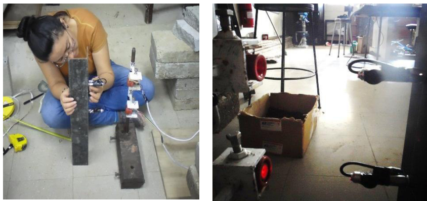
Figura H 2: Disposición final de los sensores y apuntadores láser.
