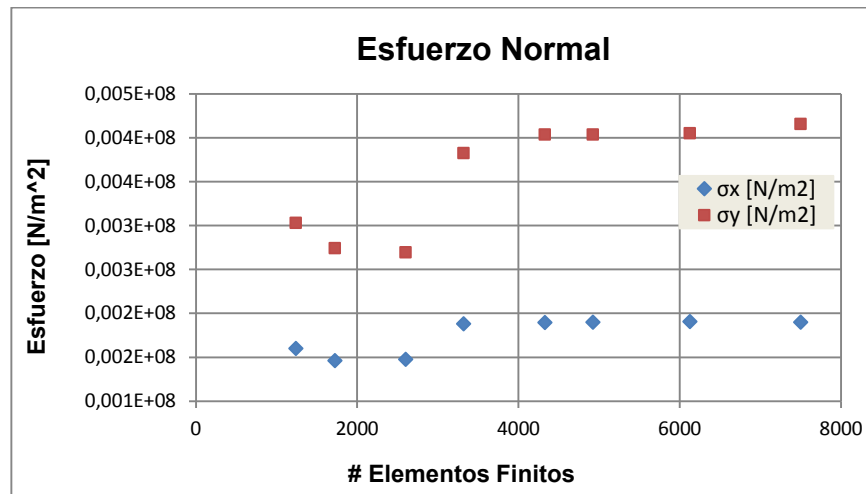
Figura D 1: Esfuerzo normal máximo para diferentes números de elementos de la malla.
