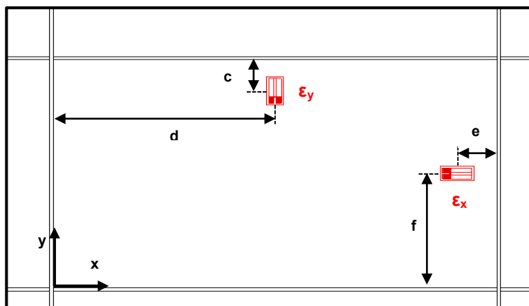
Figura 26: Esquema de la posición de los extensómetros instalados.
