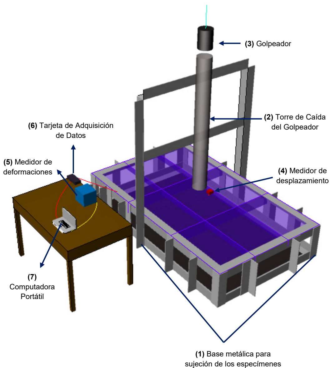
Figura 27: Esquema de los equipos de medición y elementos de ensayo.
