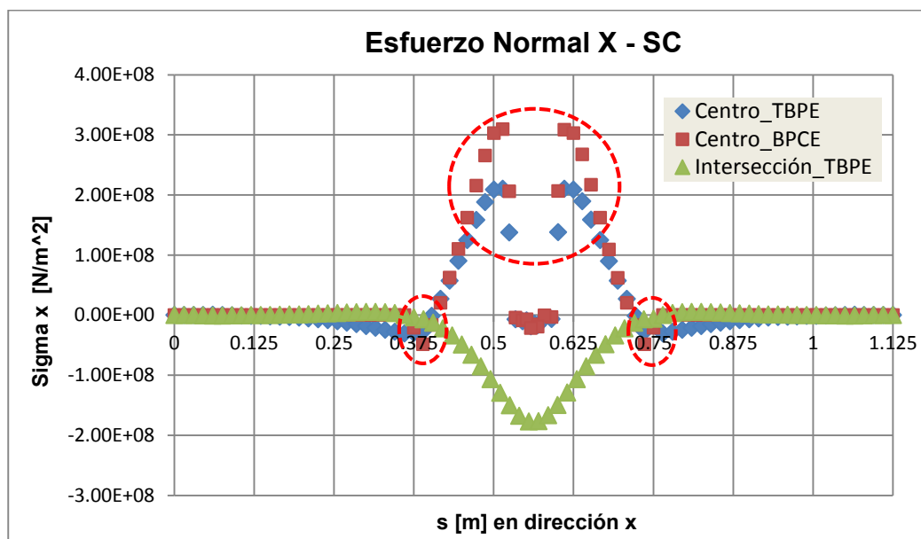
Figura 54: Distribución de \sigma_x a lo largo de distintas posiciones del panel.
