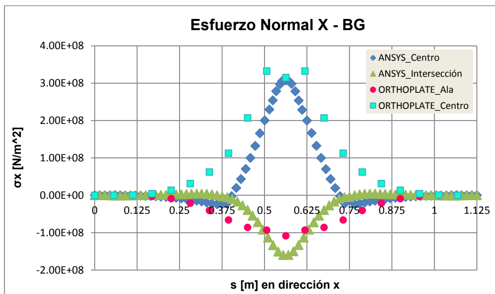
Figura 43: Distribución de \sigma_x a lo largo de distintas posiciones del panel.
