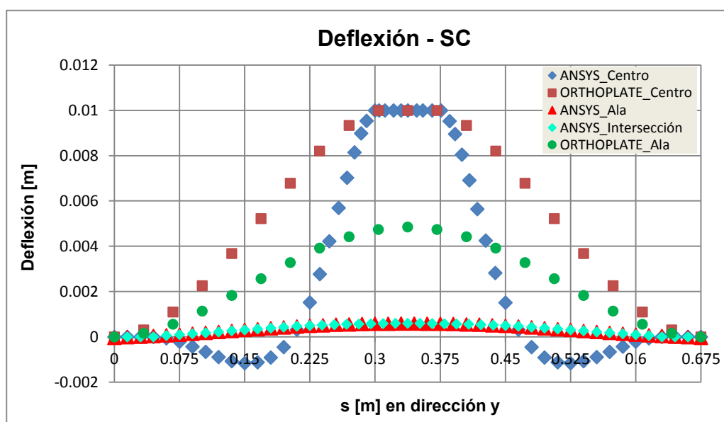
Figura 41: Perfil transversal de deflexión, a lo largo de distintas posiciones del panel. Asignación 2: SC.
