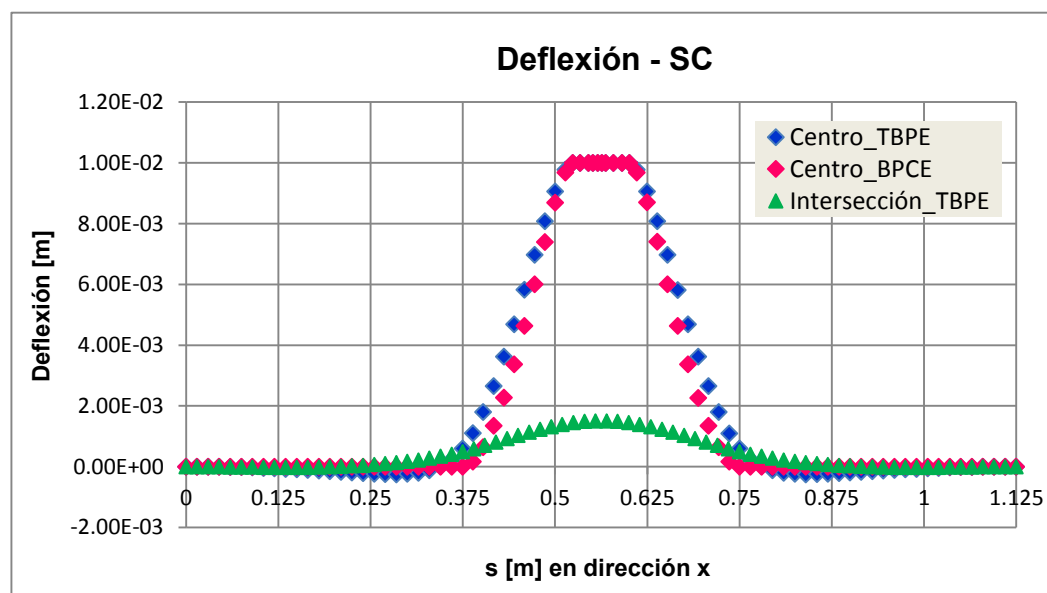
Figura 48: Deflexión en dirección “x”, a lo largo de distintas posiciones del panel. Asignación 2: SC.
