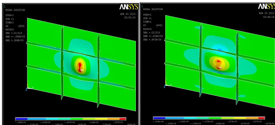
Figura 36: \sigma_x y \sigma_y del panel en el sistema de referencia global. Asignación 1.
