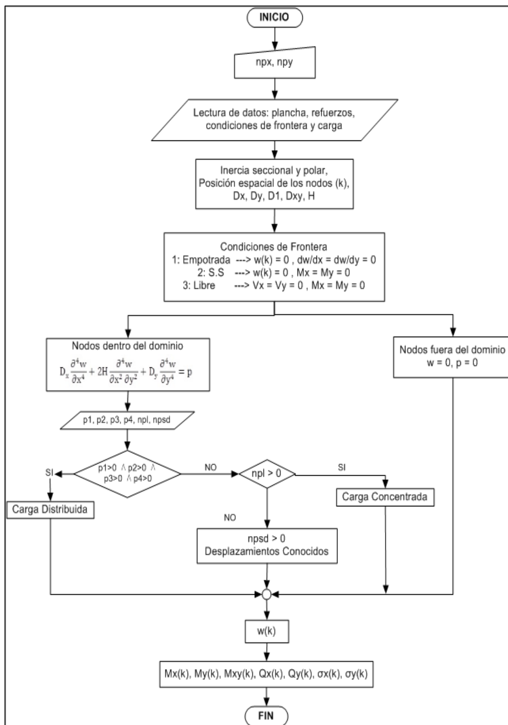
Figura 4: Diagrama de flujo del cálculo de una plancha reforzada por Diferencias Finitas.
