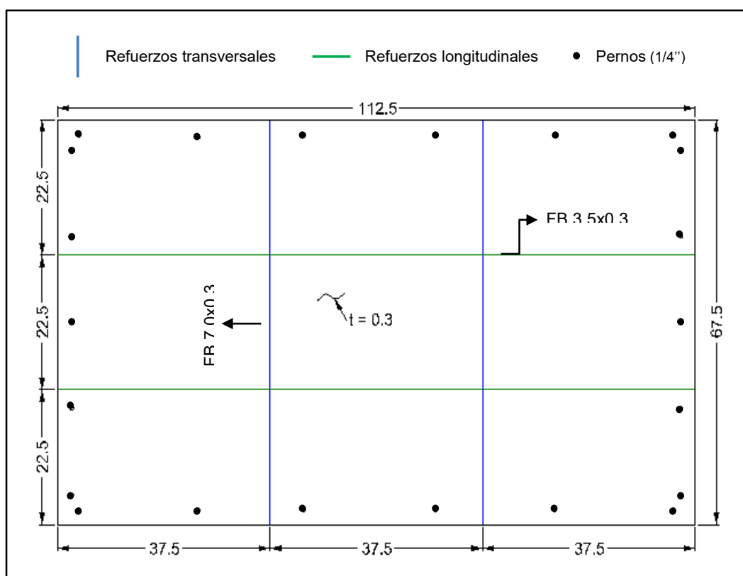
Figura 20: Plano en centímetros del panel reforzado.
