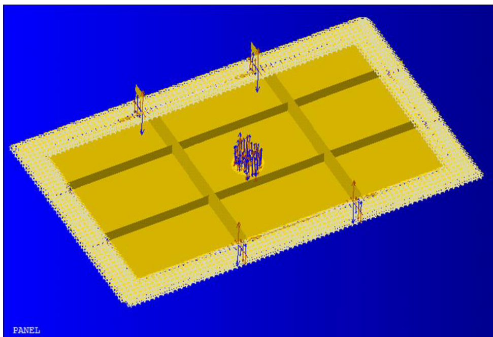
Figura 17: Asignación de desplazamientos conocidos al modelo numérico.
