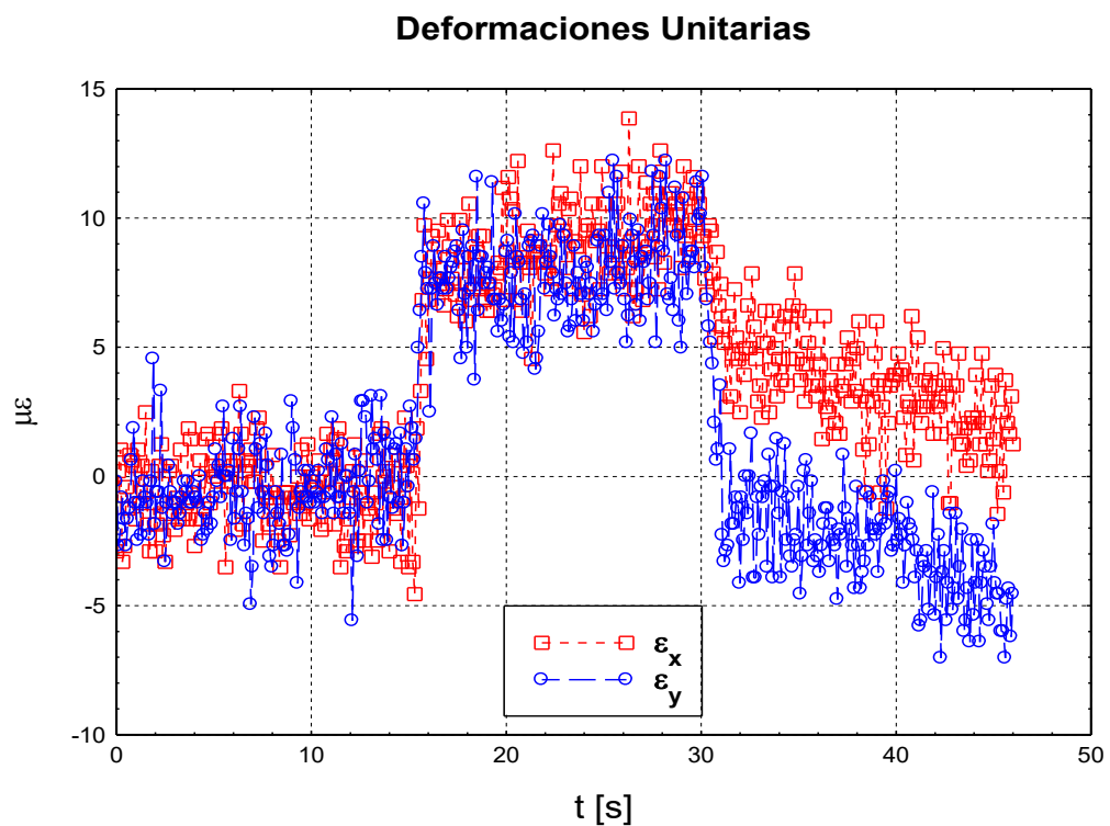
Figura 33: Microdeformaciones unitarias \epsilon_x , \epsilon_y por acción del retiro del golpeador de 4.32 kg.
