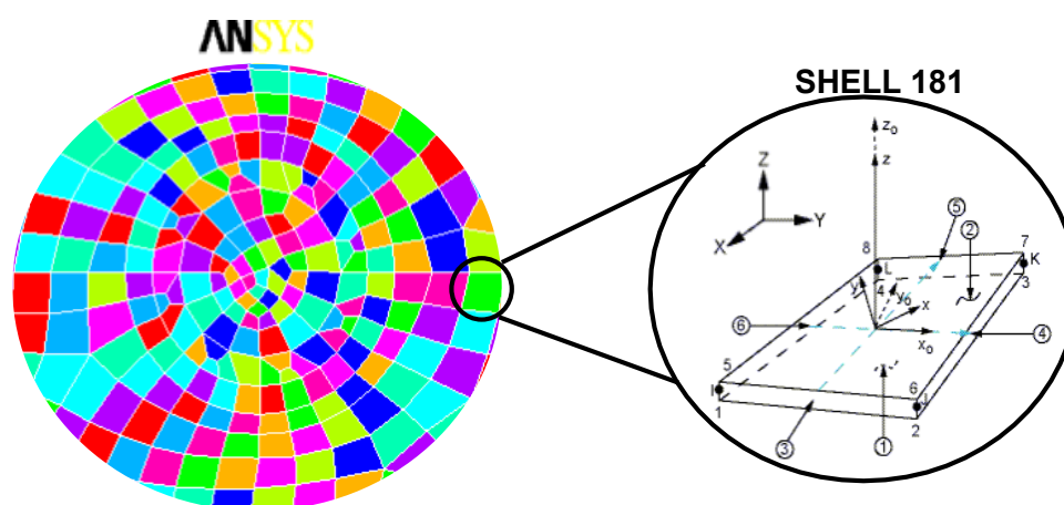
Figura 16: Detalle de la discretización de las áreas circulares del panel.
