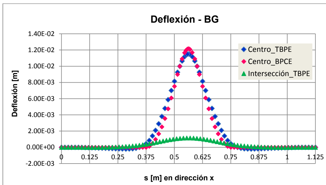
Figura 47: Deflexión en dirección “x”, a lo largo de distintas posiciones del panel. Asignación 1: BG.
