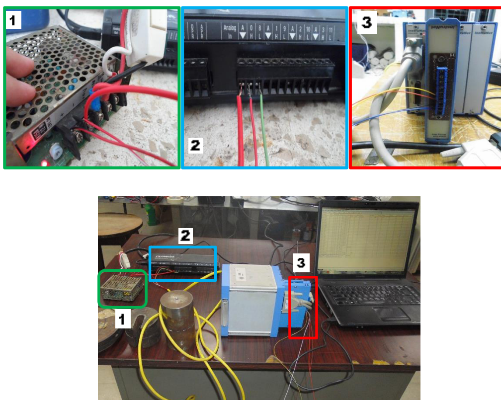
Figura 28: Conexión de los dispositivos de adquisición de datos.
