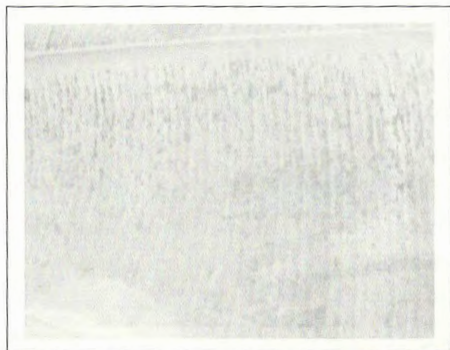
Figura. 2.2.4. Estadio cuatro.
