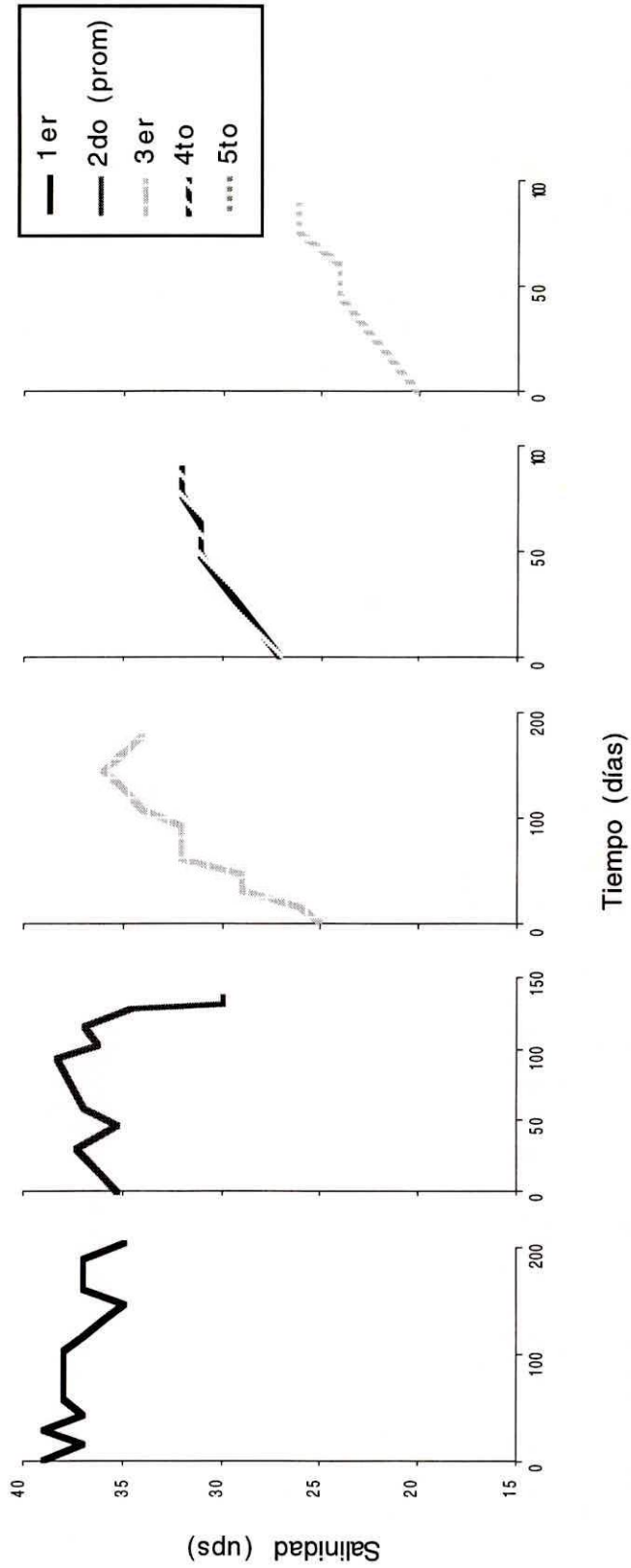
Figura 25 Variación de la salinidad en los cultivos
