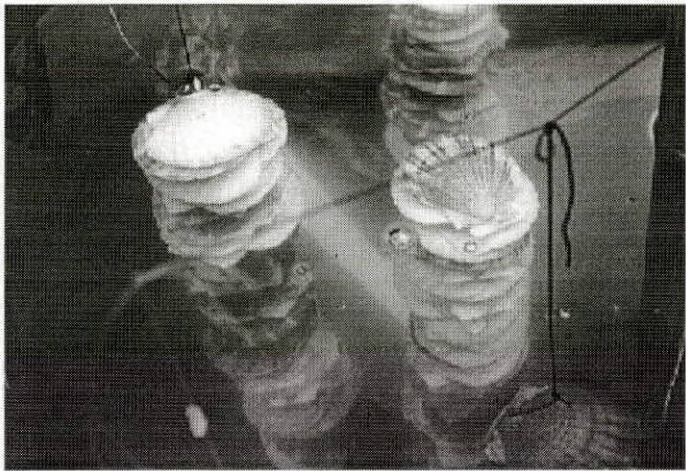
Figura 6. Colectores de semilla de ostra hechos con valvas de pectínidos
