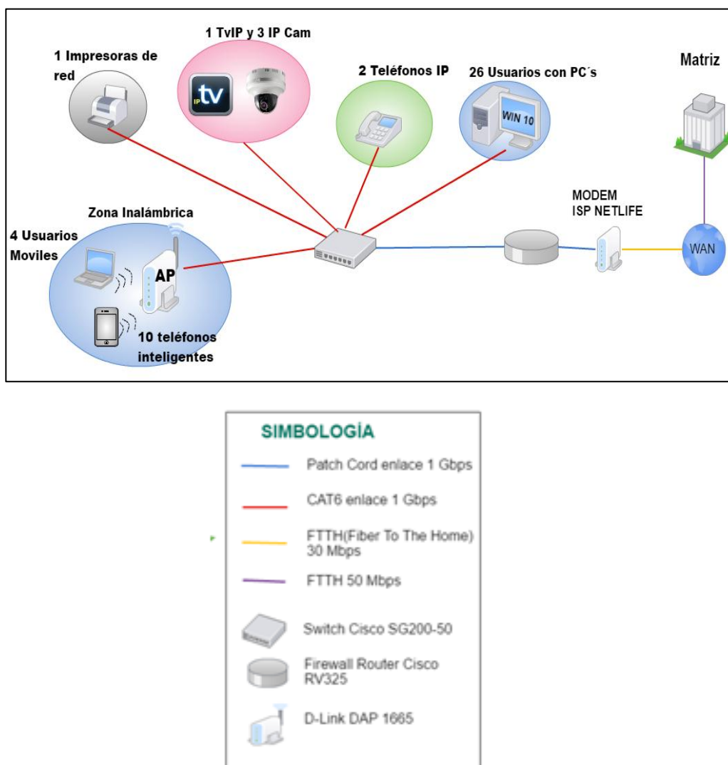
Figura.2.2: Propuesta de diseño de red sucursales.
