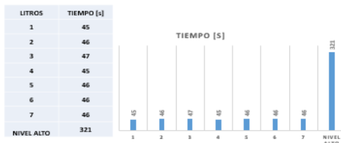
Figura 4.2: Tiempo de Llegada al Nivel Alto (LOGO! 8)
