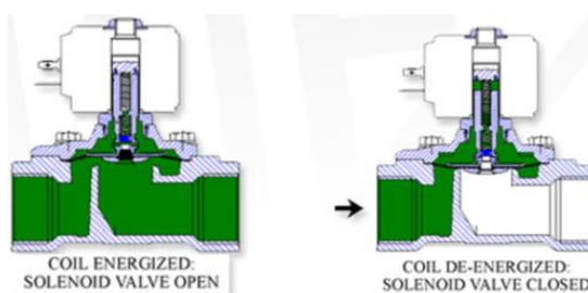
Figura 3.4: Funcionamiento de electroválvula
