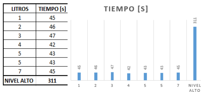
Figura 4.3: Tiempo de Llegada al Nivel Alto (Cronómetro)
