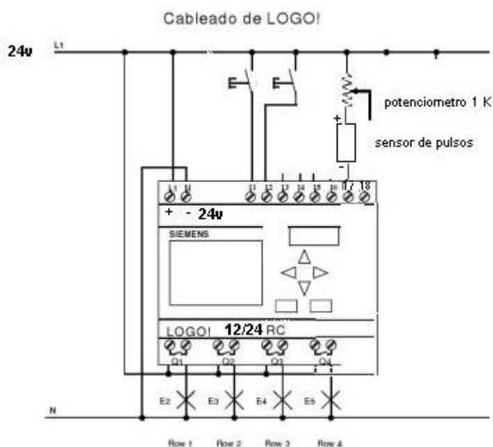
Figura 2.1: Funcionamiento de LOGO!
