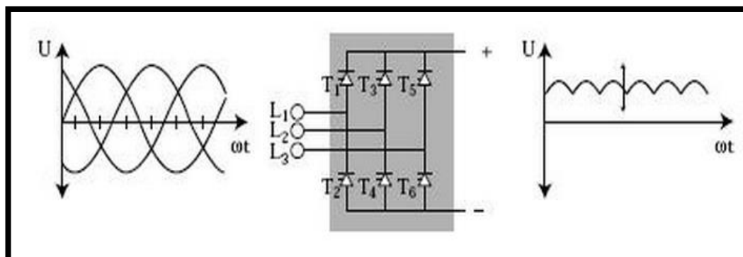
Figura 2.2 Rectificador trifásico controlado [4]
