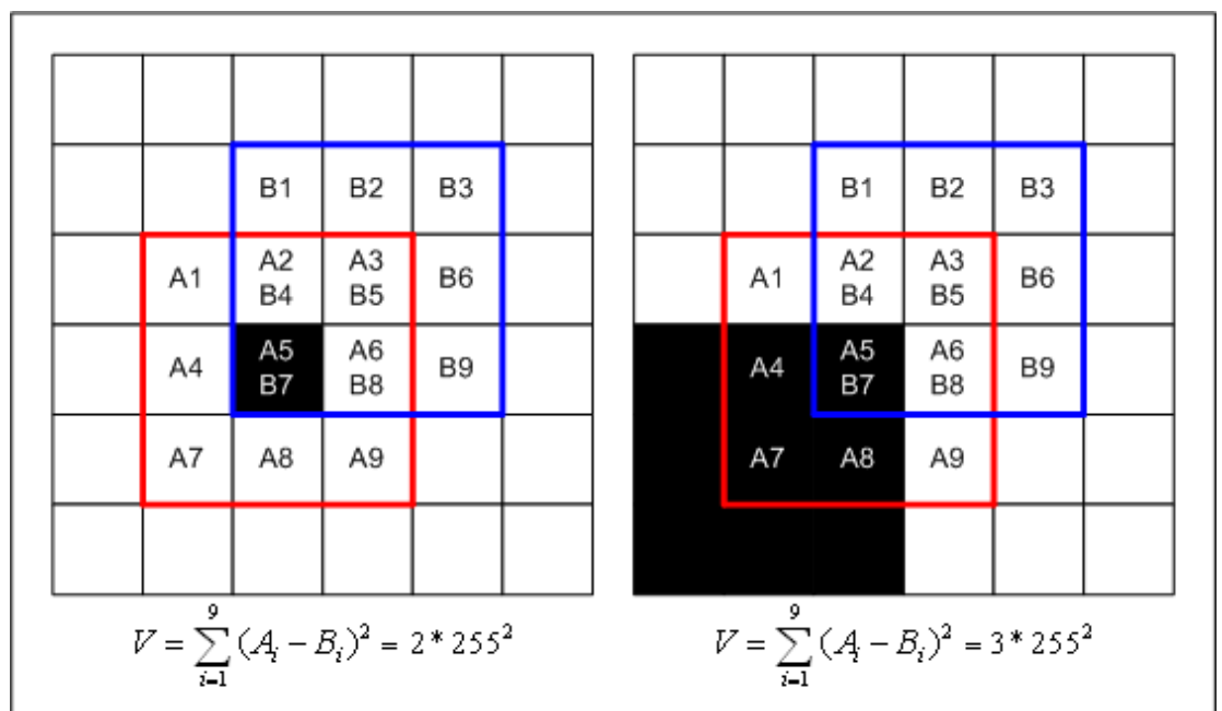
Figura 2.3 - Cálculo operador Moravec
