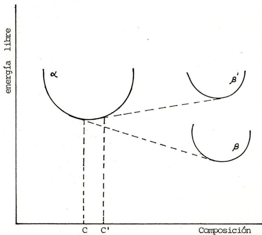
Figura 4-11.- Energías libres de una solución sólida madre \alpha , de un precipitado en equilibrio \beta , y un precipitado coherente \beta' ; C y C' representan los límites de solubilidad respectivos
