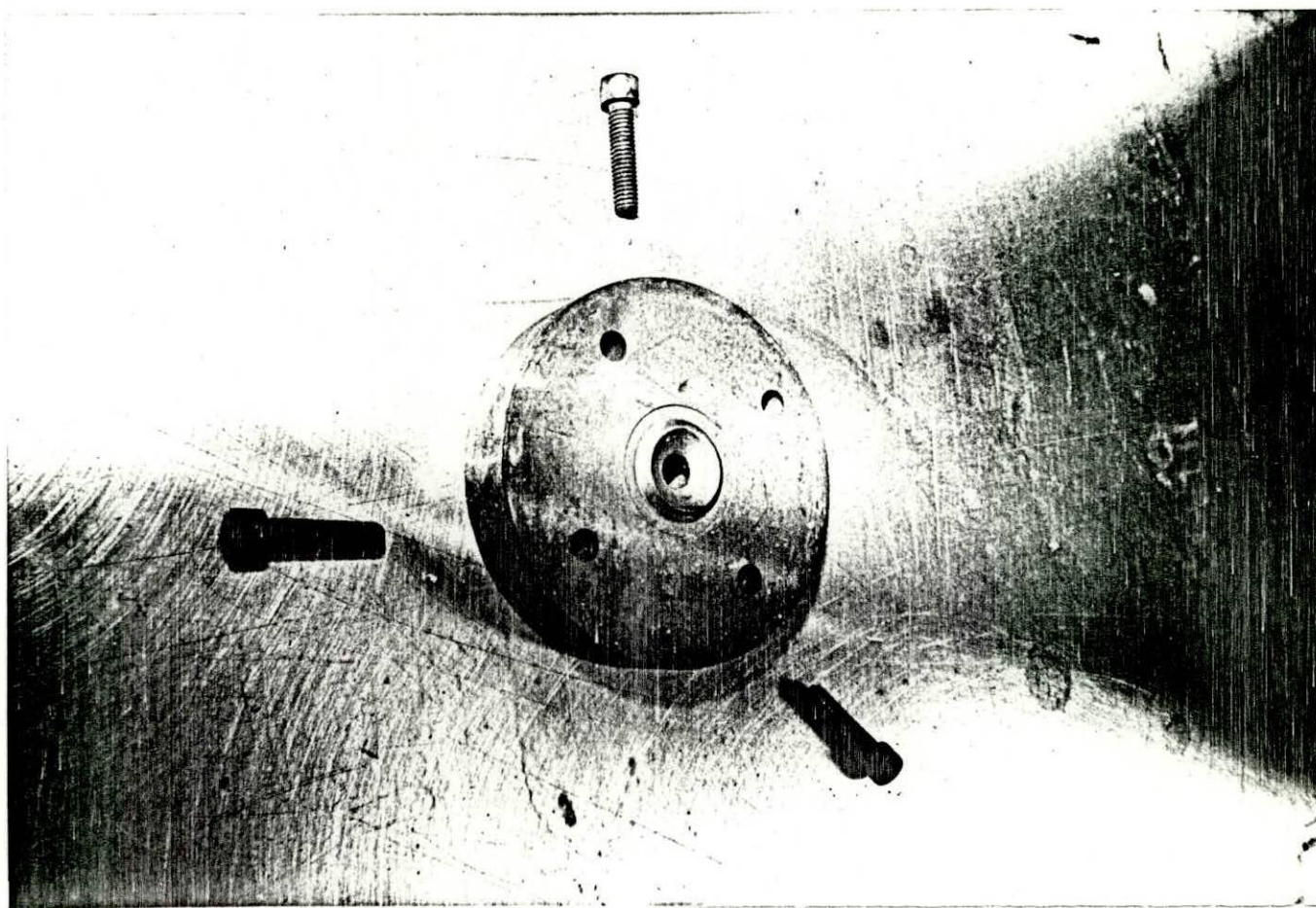
Figura 5-21.- Portamatriz, matriz y los tornillos de ajuste del cuerpo de extrusión
