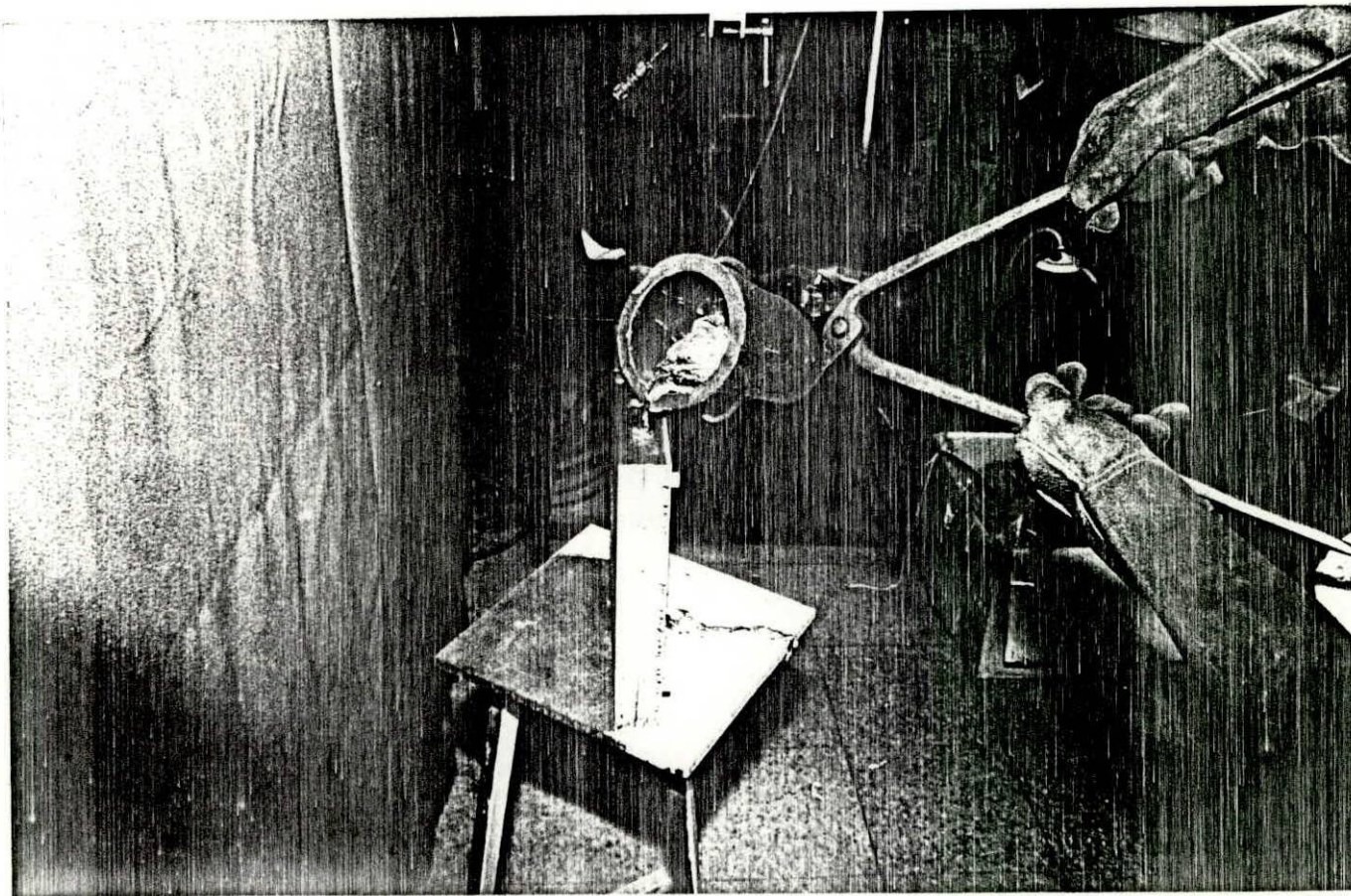
Figura 5-38. - Fundición de probetas para el ensayo de tracción
