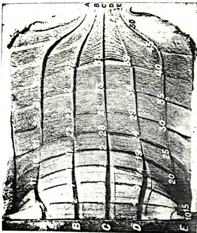
Figura 3-4b. - Extrusión parcial de un tocho con una cuadrícula, según un plano diametral
