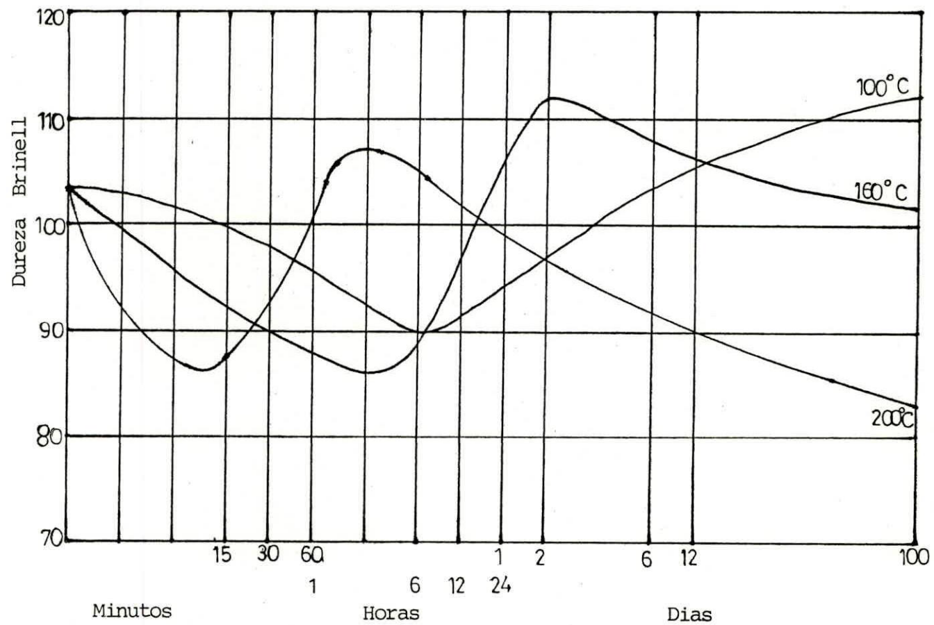
Figura 2-7.- Influencia de los calentamientos de corta duración sobre la dureza del Duraluminio.
