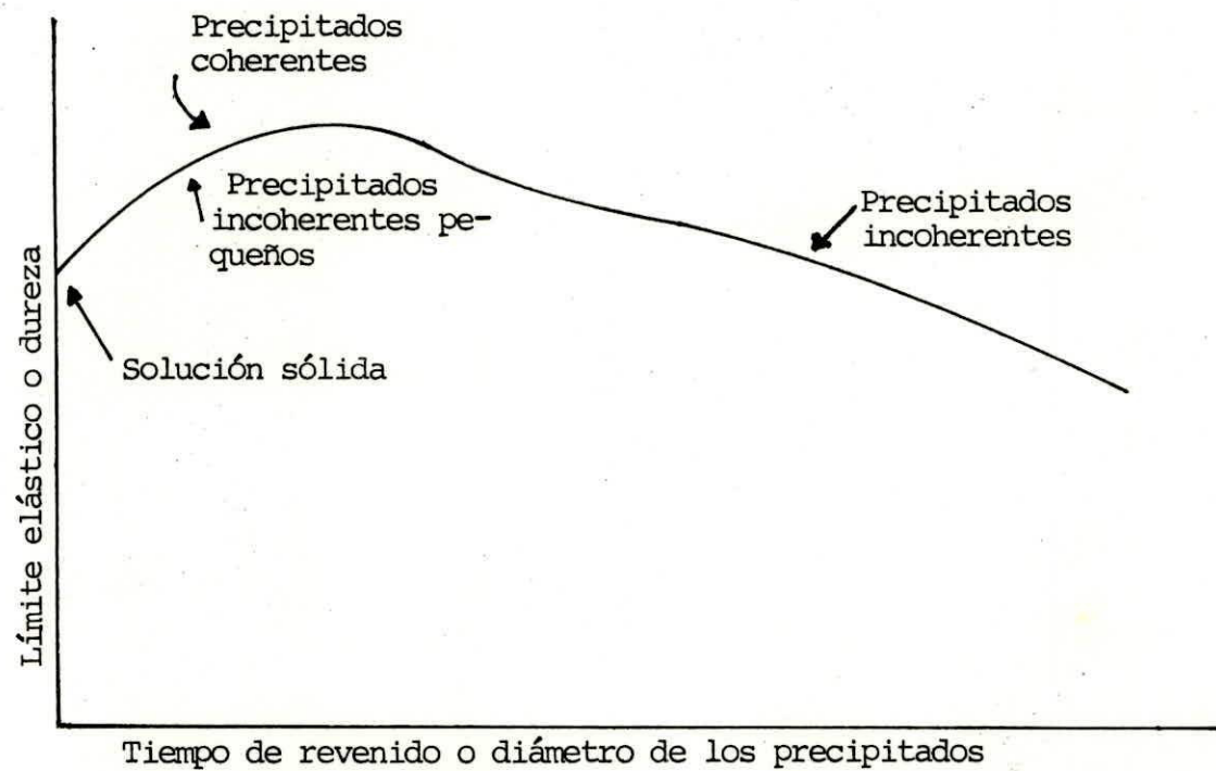
Figura 4-9.- Variación del límite elástico o de la dureza con el - tiempo de precipitación o el tamaño de los precipita- dos.
