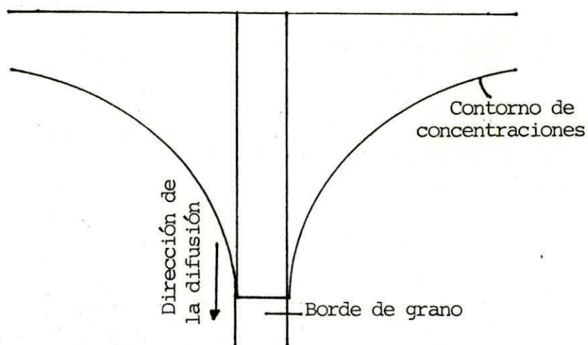
Figura 4-4.- Difusión en un borde de grano
