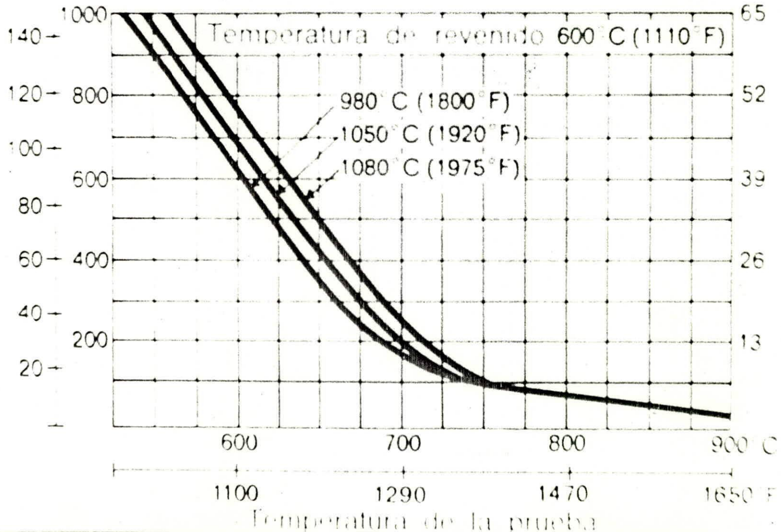
Figura 5-6b.- Resistencia a tensión a temperaturas elevadas para el acero ASSAB 8407
