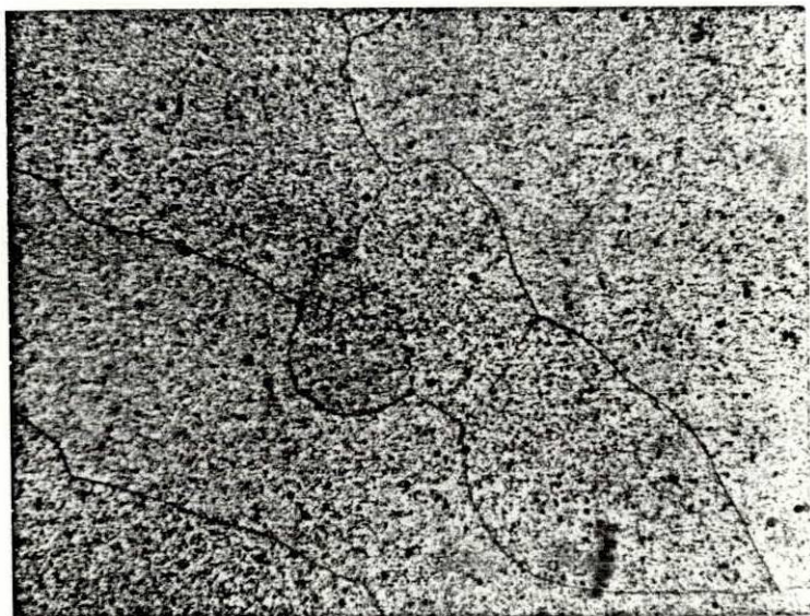
Figura 5-28.- Microestructura de una probeta extruída y enfria da al aire; posteriormente solubilizada a 570^{\circ}\text{C} durante 1 hora y enfriada al agua; envejecida a 160^{\circ}\text{C} durante 8 horas
