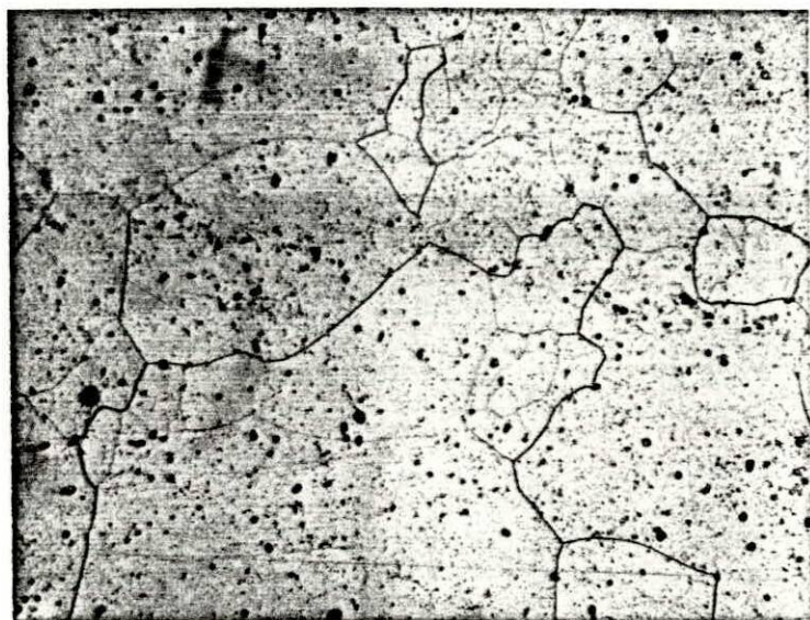
Figura 5-32.- Microestructura de una probeta extruída y enfriada al agua; posteriormente solubilizada a 570^{\circ}\text{C} durante 1 hora y enfriada en agua; envejecida a 160^{\circ}\text{C} durante 6 horas
