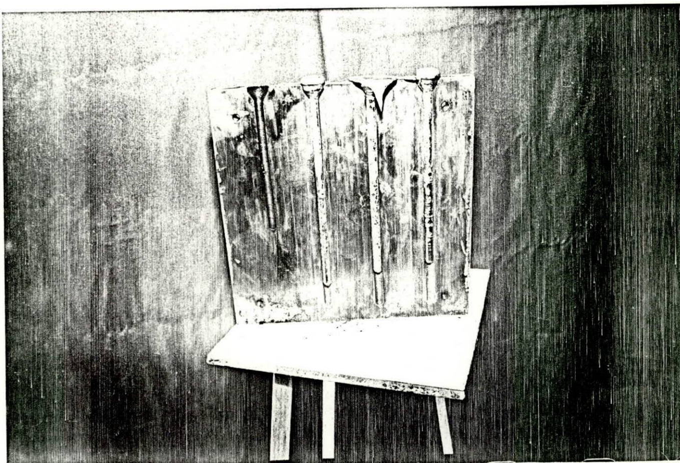
Figura 5-39. - Probetas fundidas para el ensayo de tracción
