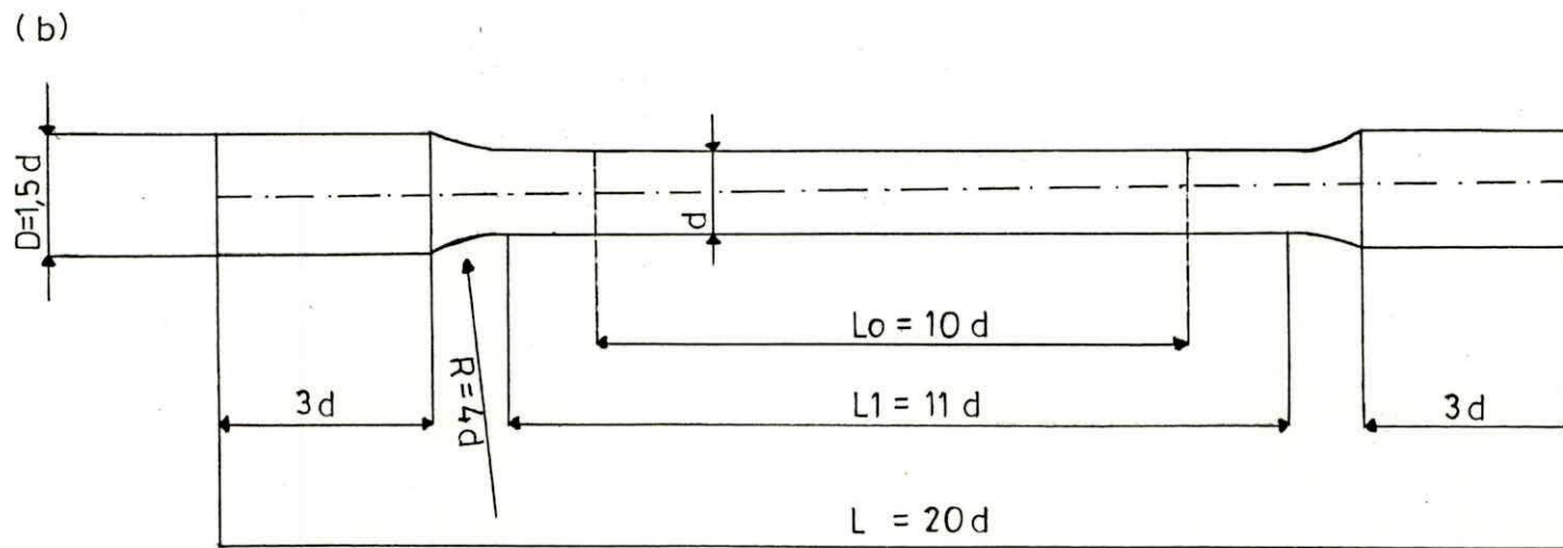
Figura 2-4.- Probetas Proporcionales; (a) Probeta Corta, (b) Probeta Larga
