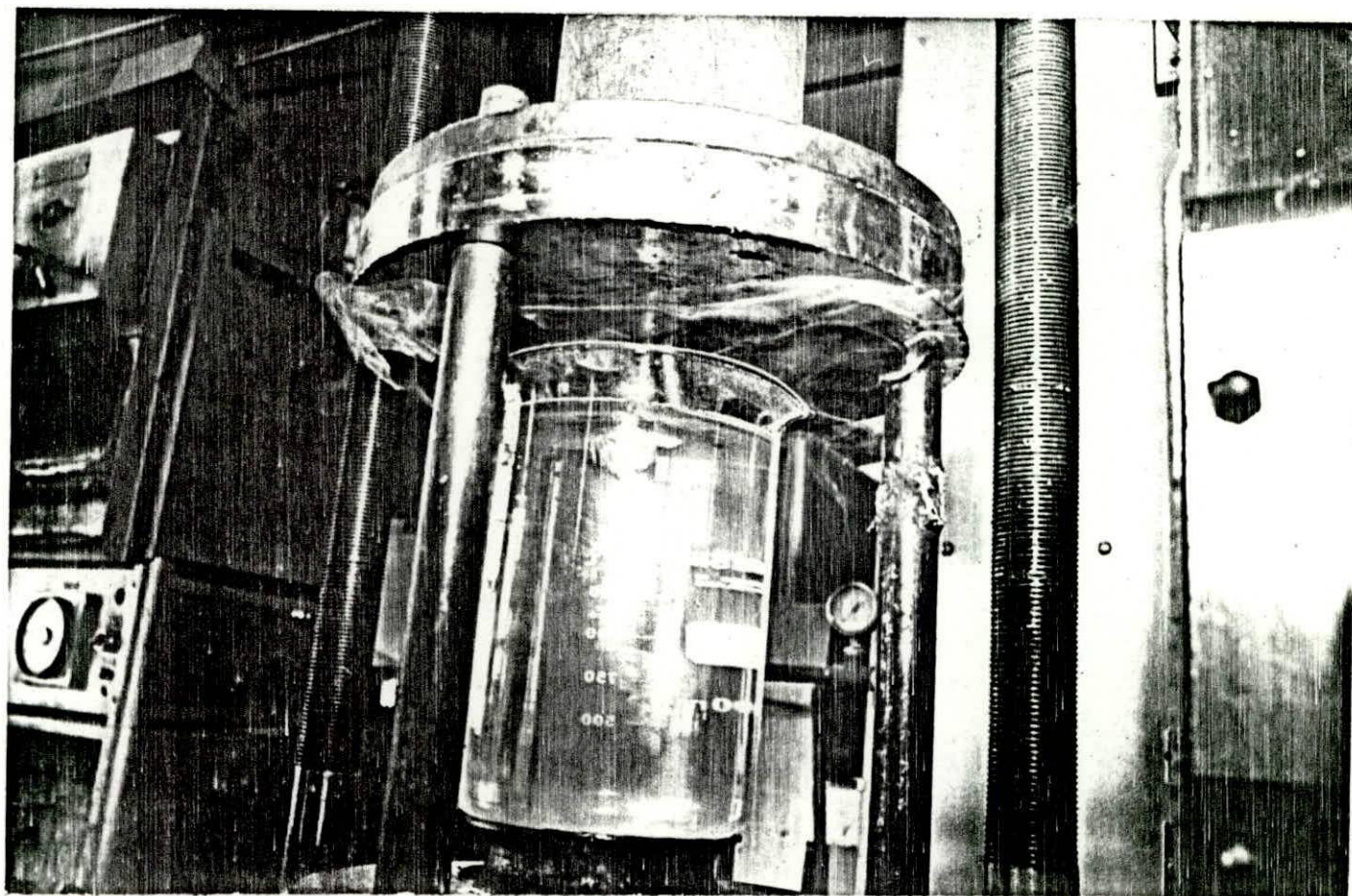
Figura 5-22.- Enfriamiento rápido directamente al agua del producto extruído
