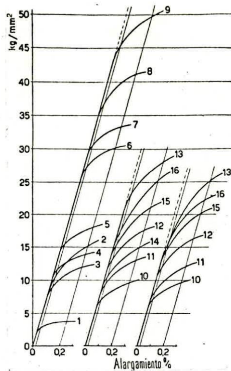
Figura 2-5.- Diagramas de tracción de algunas aleaciones de Al
