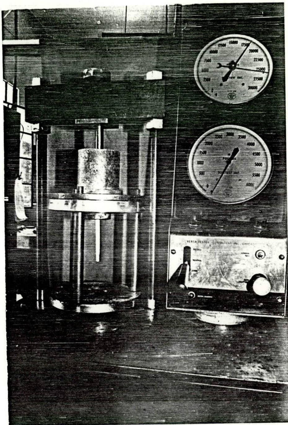
Figura 5-17. .- Inicio del proceso de extrusión
