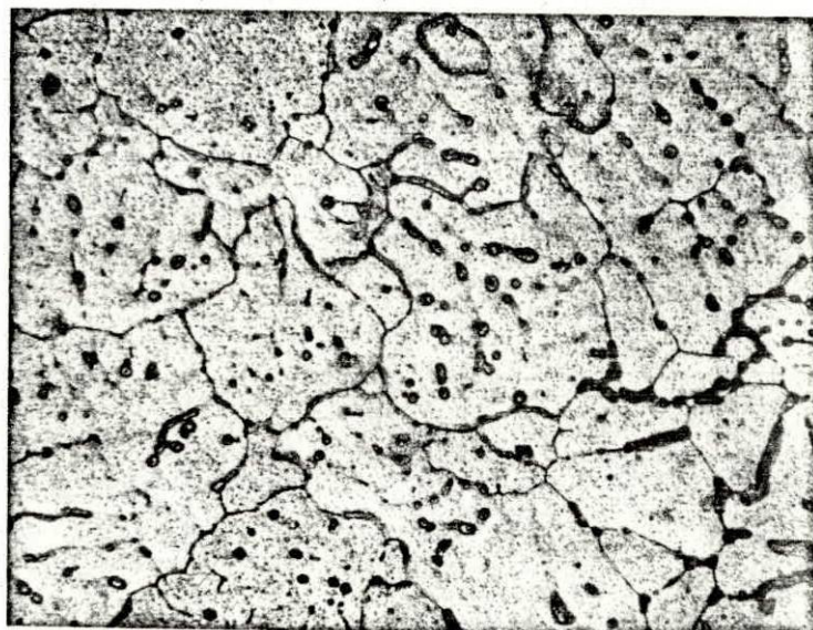
Figura 5-24. .- Microestructura del tocho fundido.
