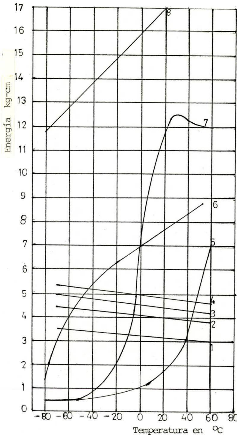
Figura 2-8.- Influencia de la temperatura sobre la tenacidad.
