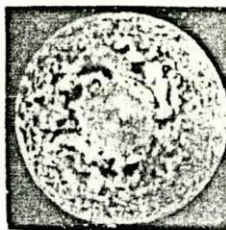
Figura 3-7.- Defecto de Extrusión de un tocho cilíndrico macizo
