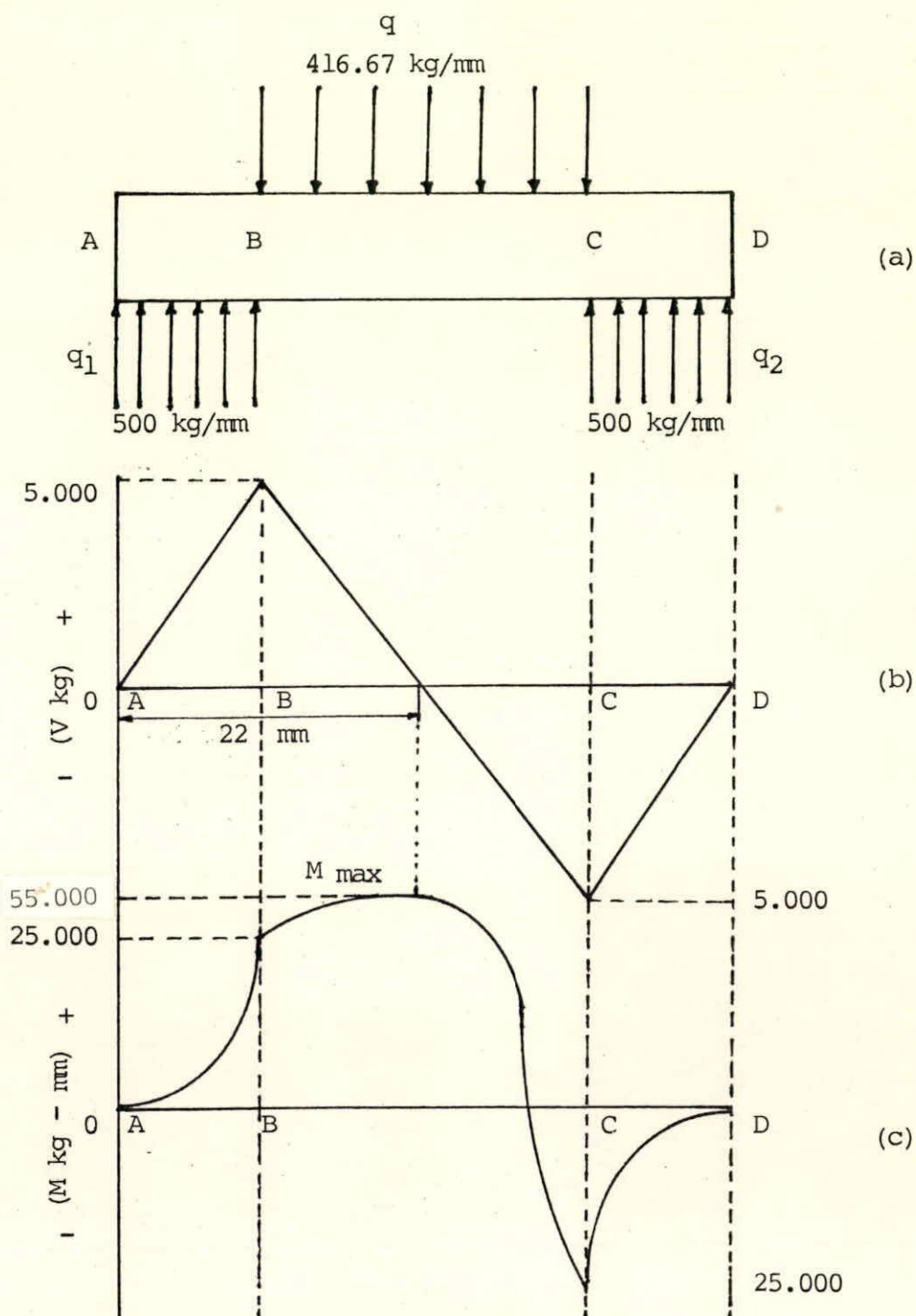
Figura 5-10.- Diagrama de cuerpo libre de la matriz completa (a), diagrama de fuerza cortante (b) y, diagrama del momento flector (c).
