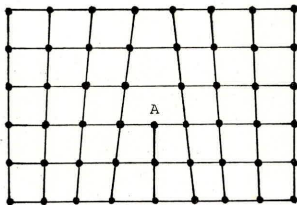
Figura 4-5.- Difusión a lo largo de una dislocación de cuña.
