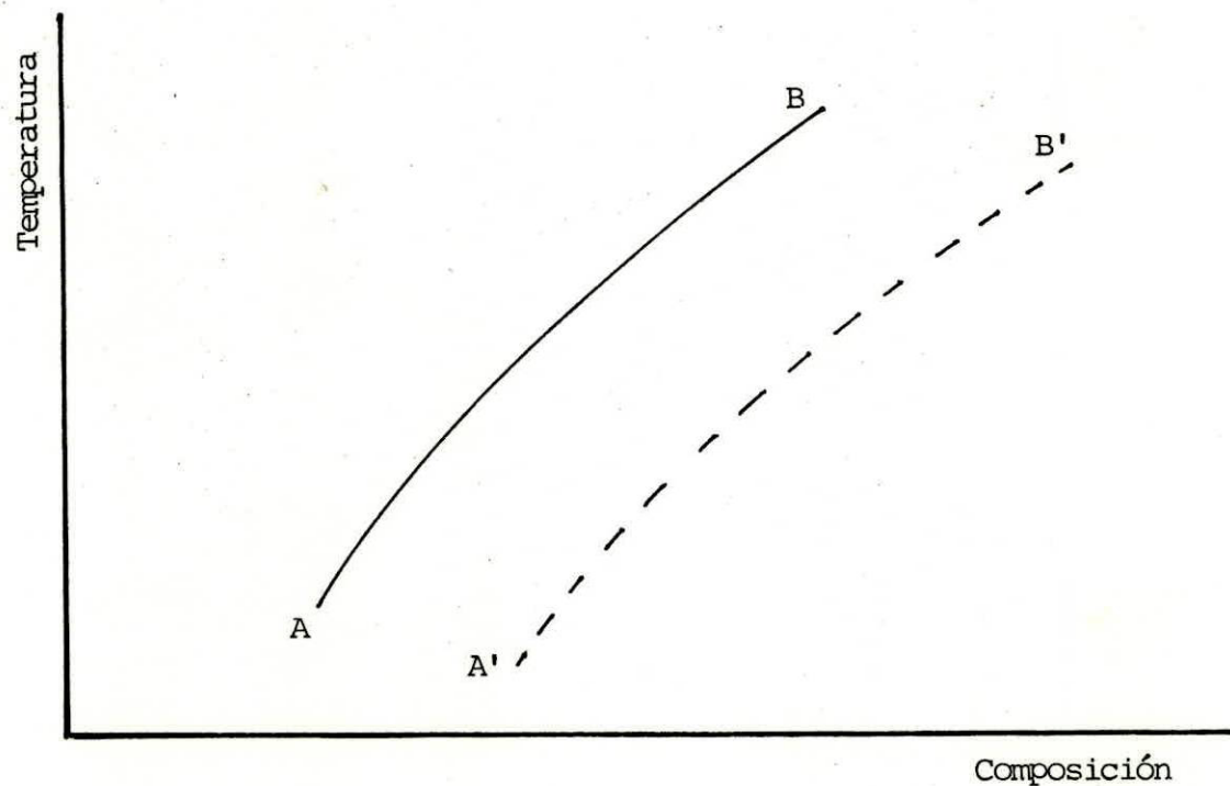
Figura 4-10.- Límite de solubilidad. AB representa el límite de solubilidad respecto a la precipitación de \beta , y A'B' es el correspondiente a la precipitación de \beta' .
