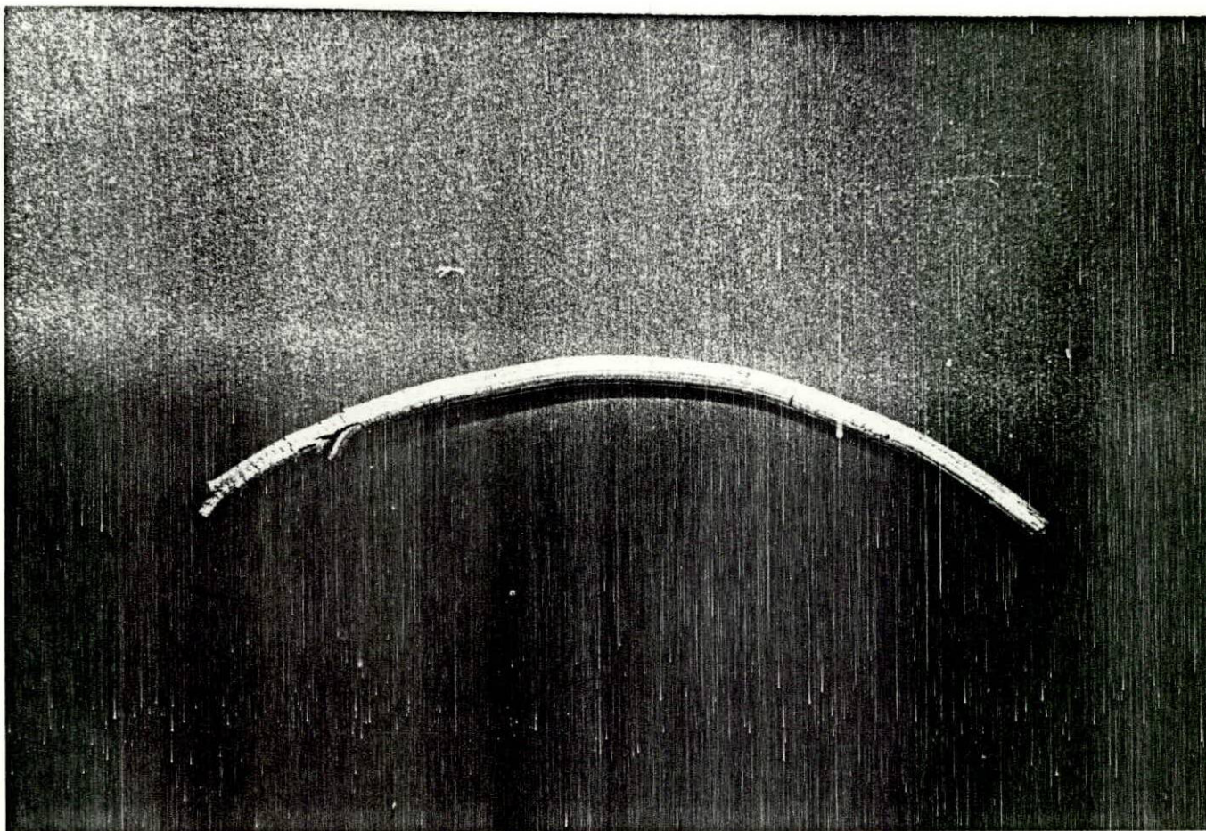
Figura 5-14.- Grietas en el producto extruído debido a una temperatura demasiado alta
