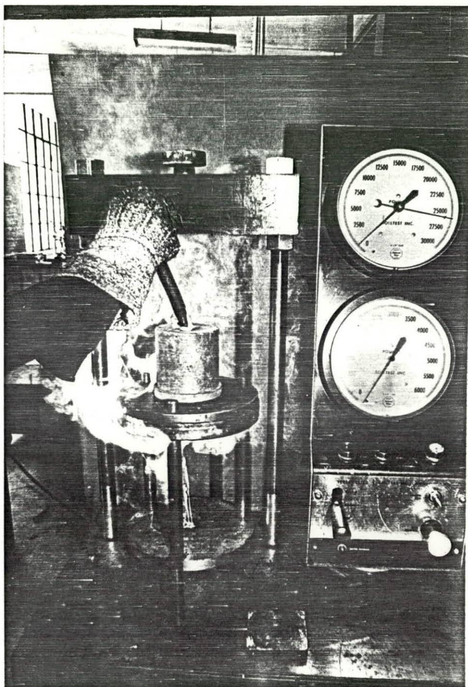
Figura 5-16. .- Lubricación inicial del recipiente antes del proceso de extrusión
