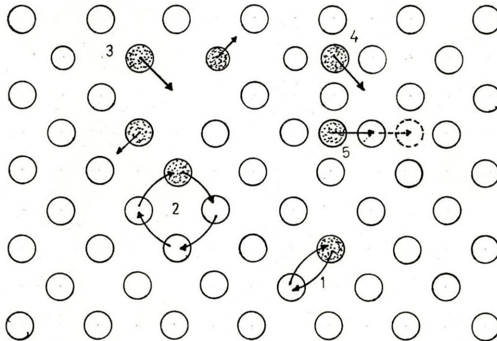
Figura 4-3.- Mecanismos elementales de la difusión
