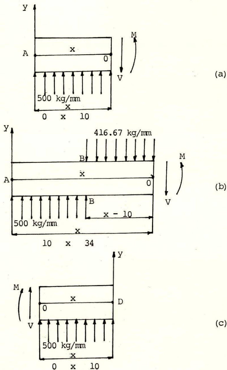
Figura 5-11.- Diagrama de cuerpo libre de las distintas secciones de la matriz
