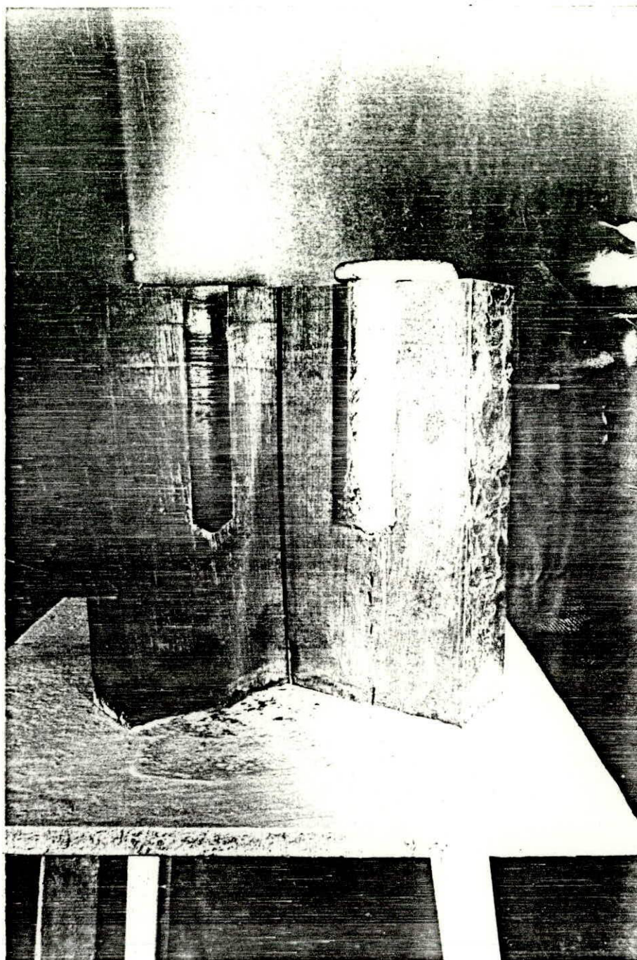
Figura 5-3.- Tocho fundido de la aleación 6063
