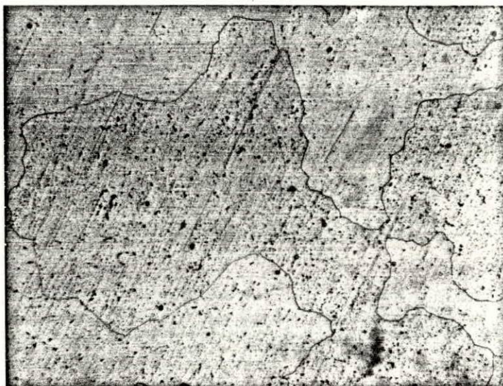
Figura 5-27. - Microestructura de una probeta extruída y enfriada - al aire; posteriormente solubilizada a 570°C durante una hora y enfriada al agua
