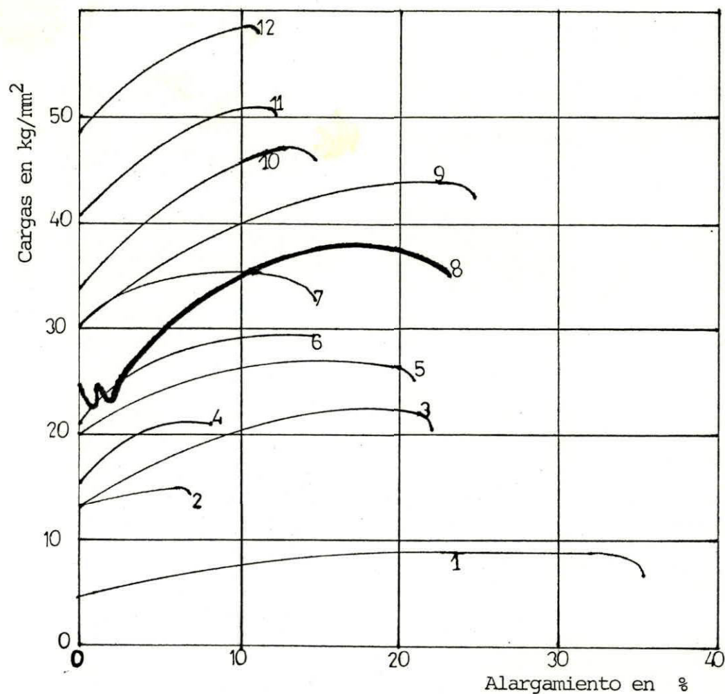
Figura 2-1.- Diagramas de tracción de diferentes aleaciones de Aluminio y del acero suave.
