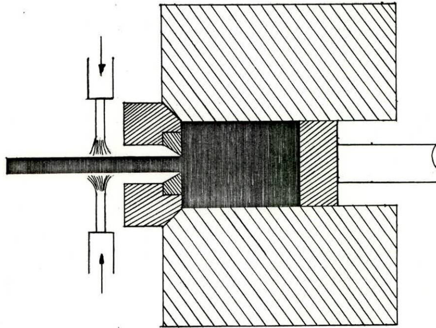
Figura 6-1.- Enfriamiento mediante un chorro de agua a la salida del producto extruído de la matriz
