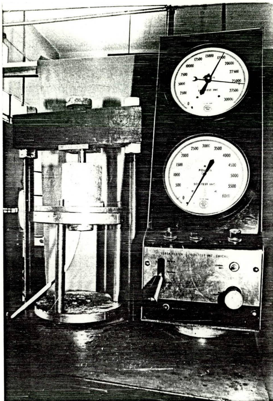
Figura 5-19. - Un tiempo anterior al final del proceso de extrusión
