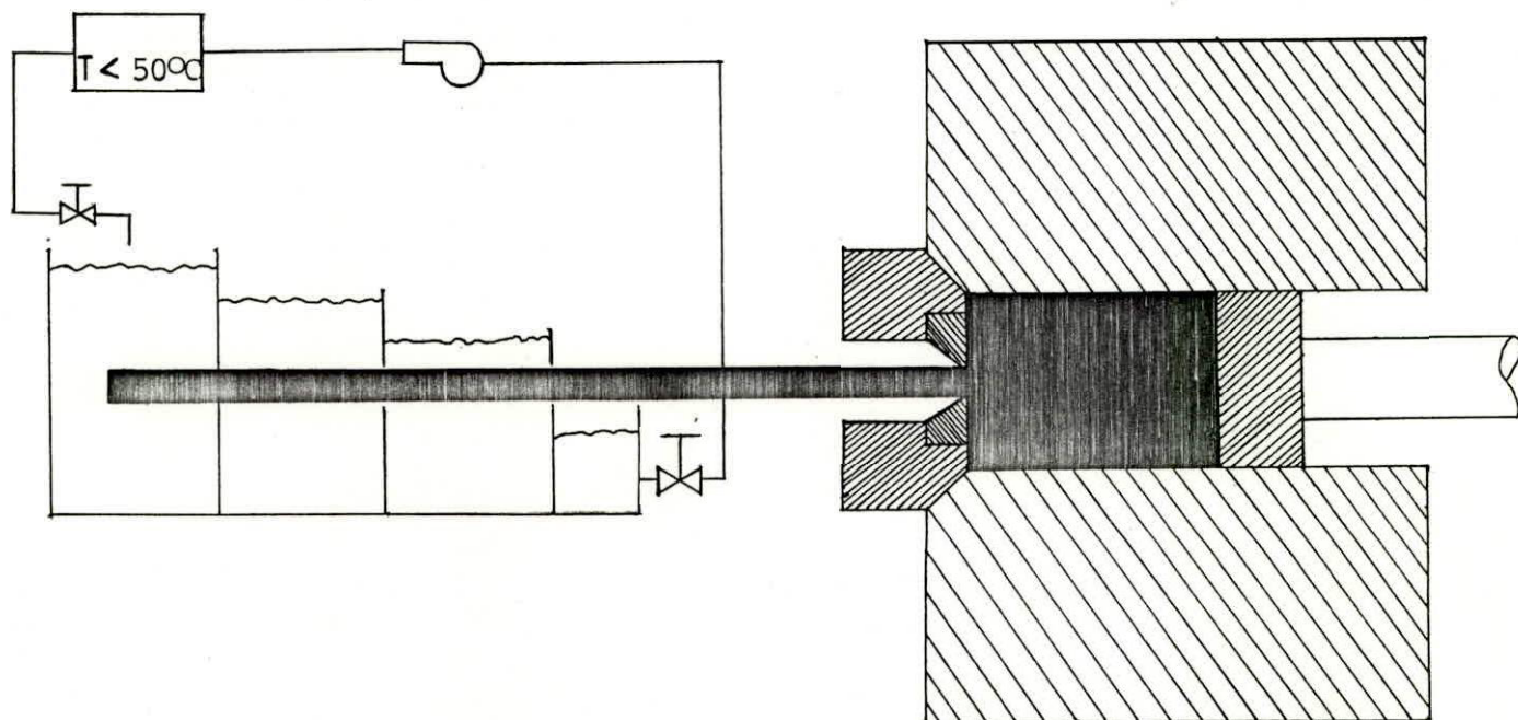
Figura 6-2.- Enfriamiento directo al agua mediante cubetas especiales
