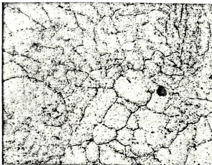
、 Figura 5-25. - Microestructura del tocho fundido y homogenizado
