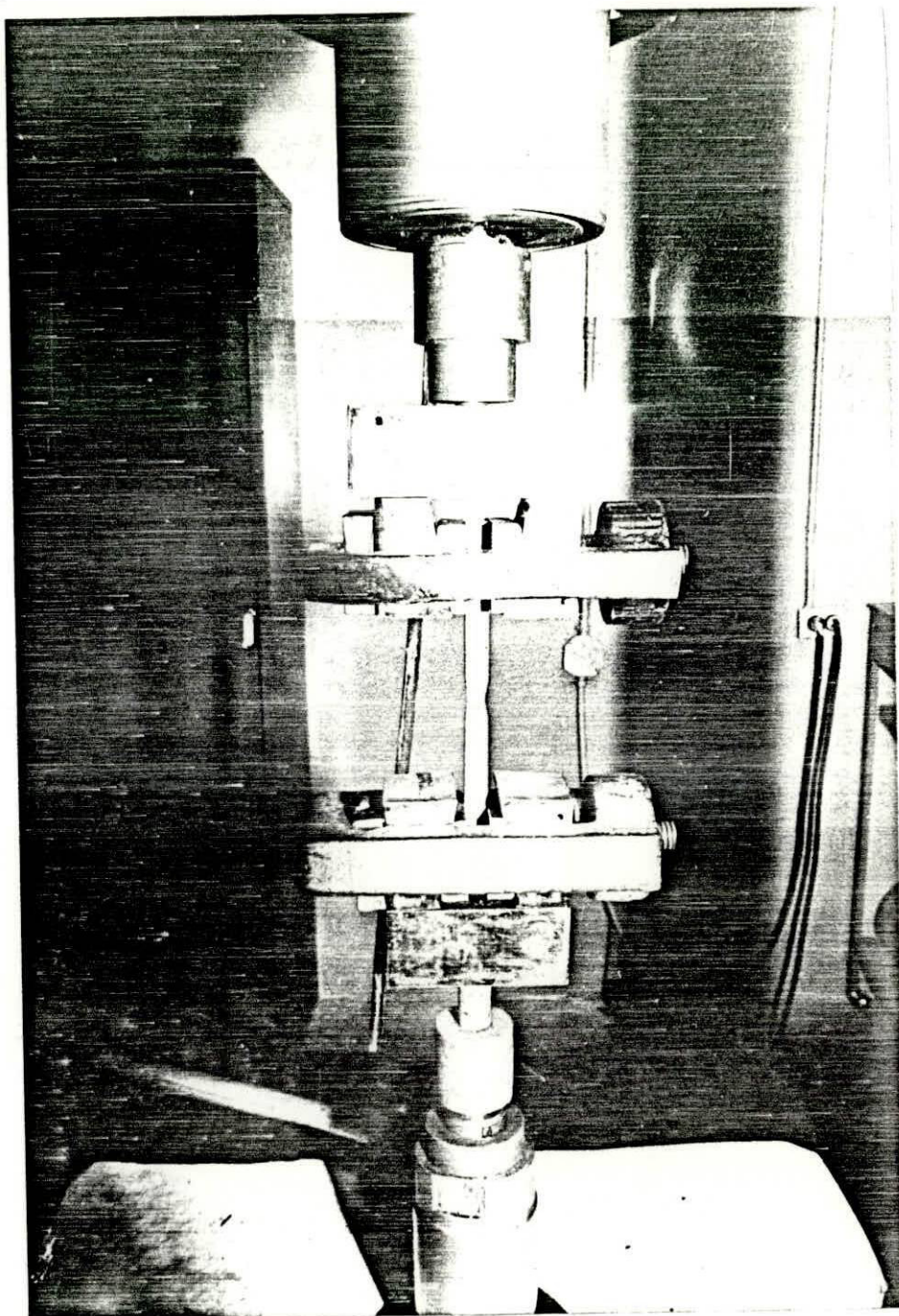
Figura 5-40.- Estricción durante el ensayo de tracción
