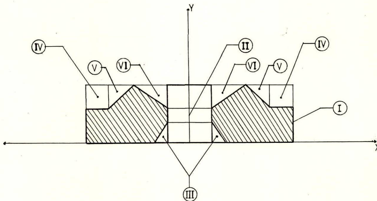
Figura 5-8.- División de la superficie de la matriz en distintas áreas para el cálculo del centro de gravedad ( Y_G ) y el momento de inercia ( I_G )
