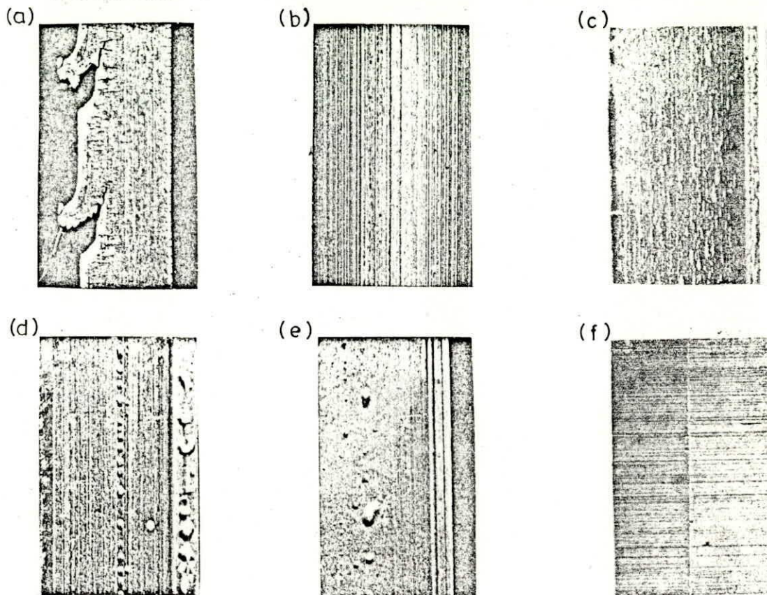
Figura 3-8.- Defectos de extrusión
