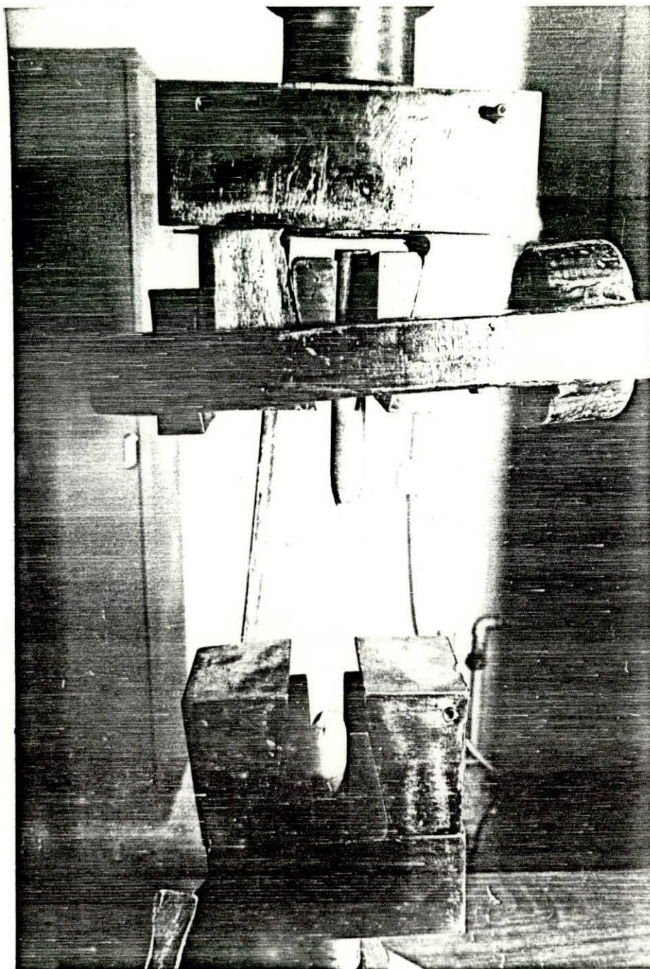
Figura 5-41.- Rotura de la probeta durante el ensayo de tracción
