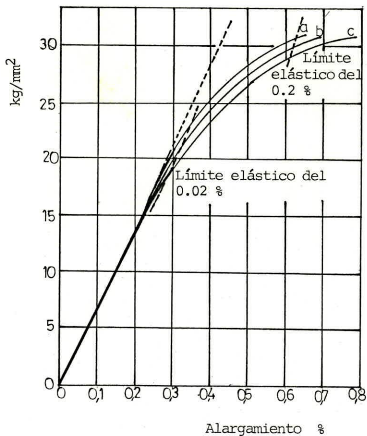
Figura 2-2.- Influencia de la velocidad de incremento de la carga en el ensayo de tracción sobre las curvas de precisión, del Duraluminio.
