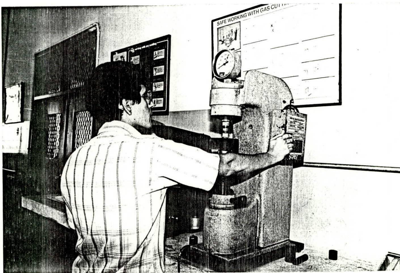
. Figura 5-37. .- Toma de dureza de una probeta
