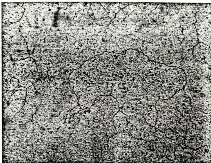
Figura 5-26.- Microestructura de una probeta extruída y enfriada al aire
