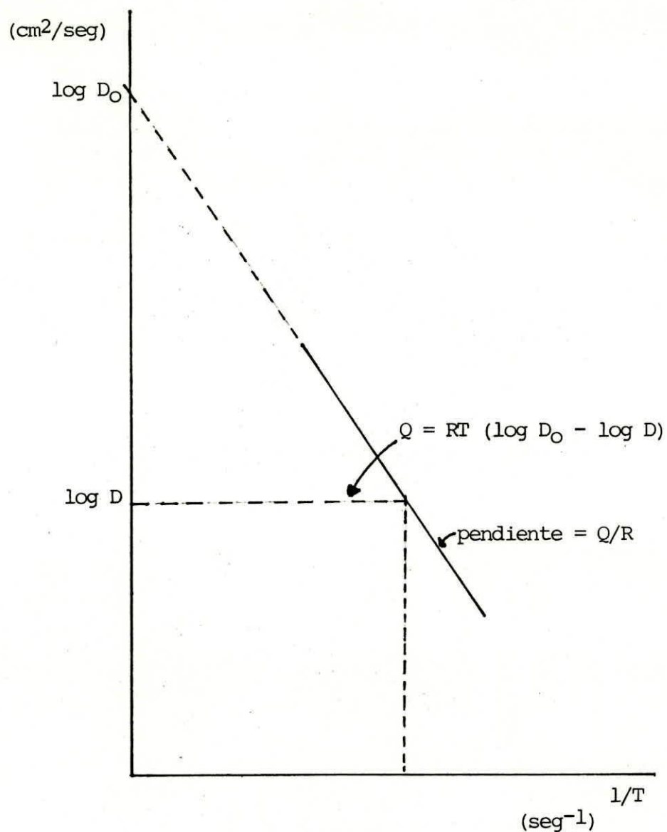
Figura 4-2.- Variación de la constante de difusión con la temperatura
