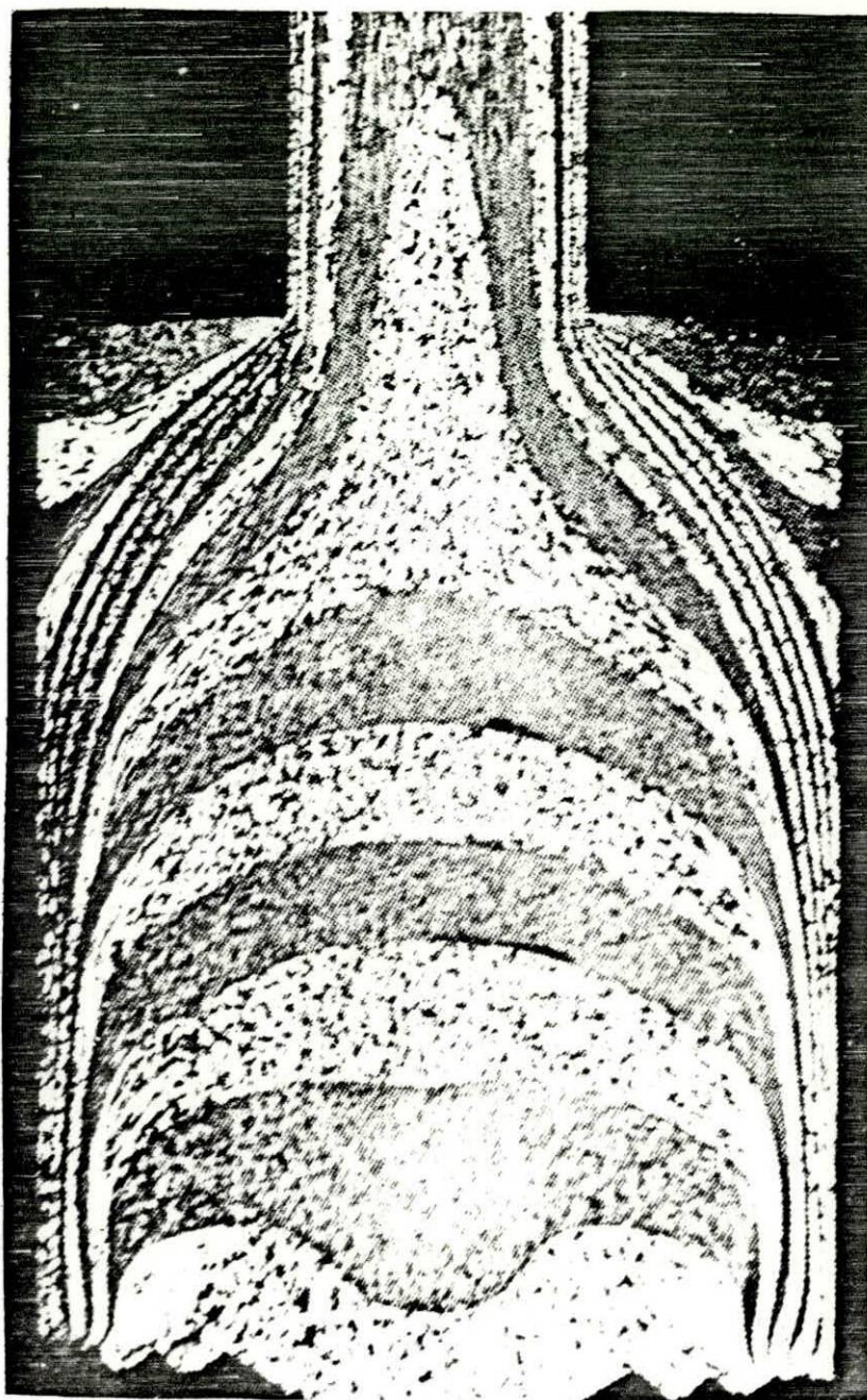
Figura 3-4a. - Proceso de fluencia en la extrusión directa
