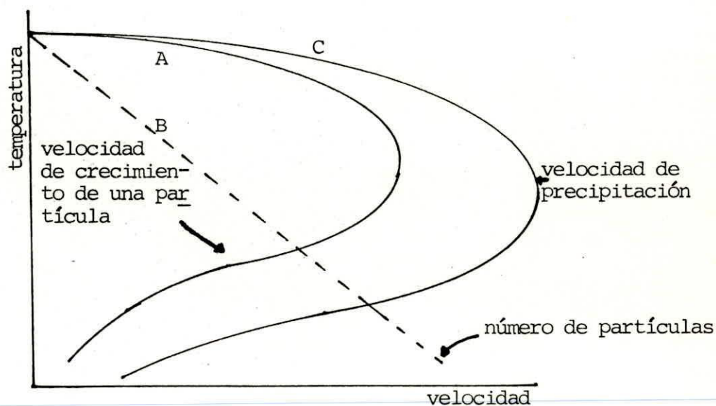
Figura 4-7. — Curvas de velocidad de crecimiento de una partícula y de velocidad de precipitación
