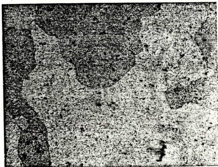
. Figura 5-36. - Microestructura de una probeta extruída y enfriada al agua; posteriormente envejecida a 160^{\circ}\text{C} durante 24 - horas
