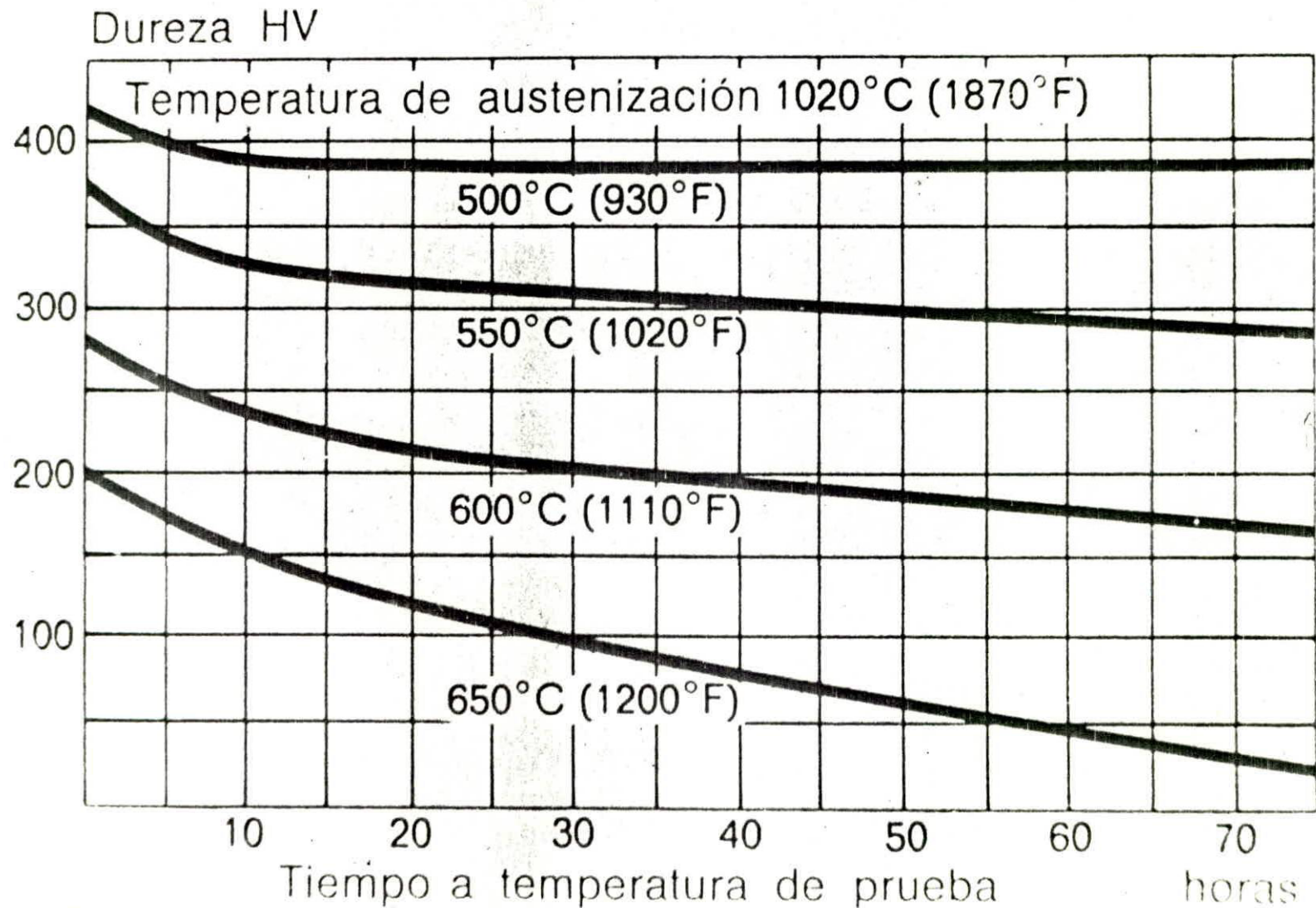
Figura 5-6a.- Dureza superficial a temperaturas elevadas para el acero ASSAB 8407
