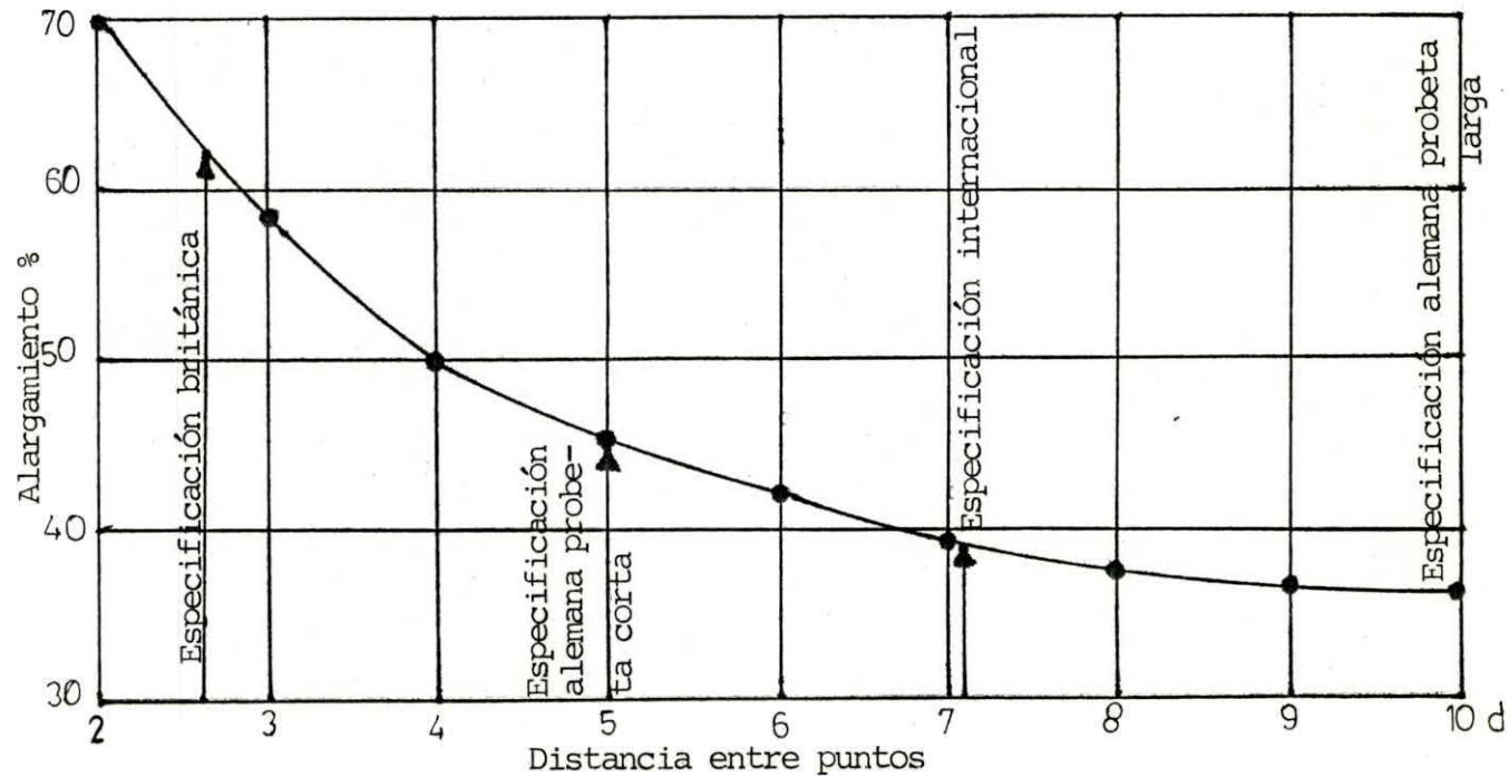
Figura 2-3.- Alargamientos de rotura en función de la distancia entre puntos de la probeta de Aluminio puro blando; probetas de 20 mm. de diámetro.
