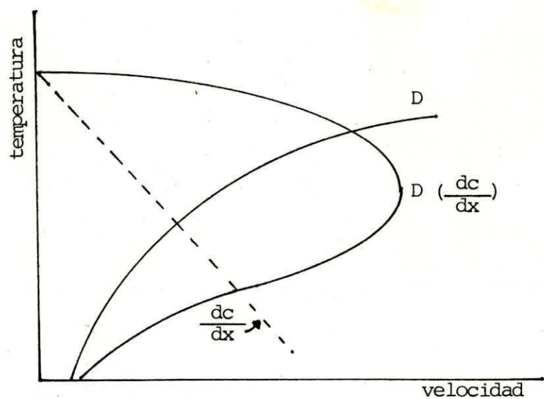
Figura 4-6. — Efecto de la temperatura en la velocidad de crecimiento de una partícula de precipitado
