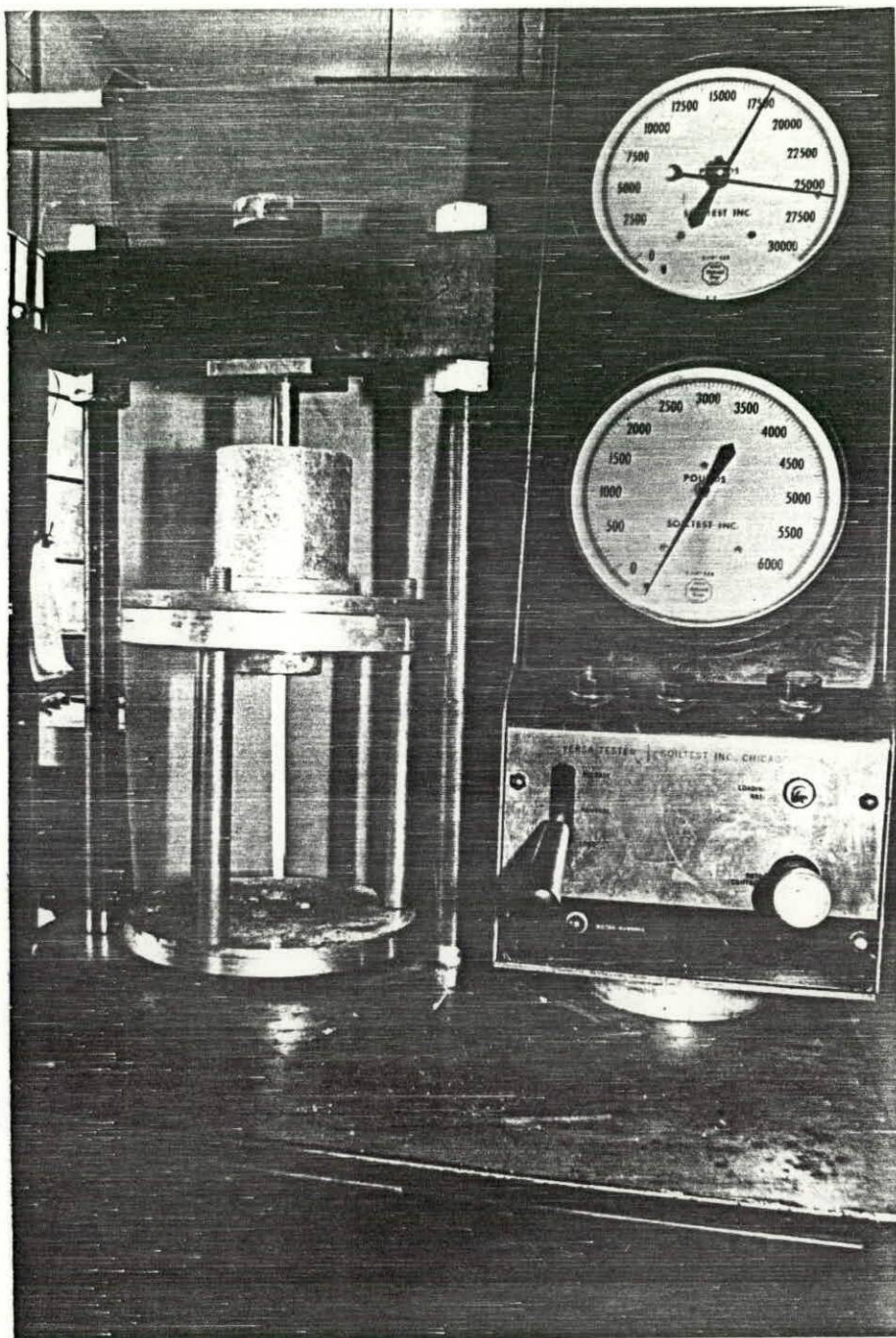
Figura 5-18. - Proceso de extrusión en marcha
