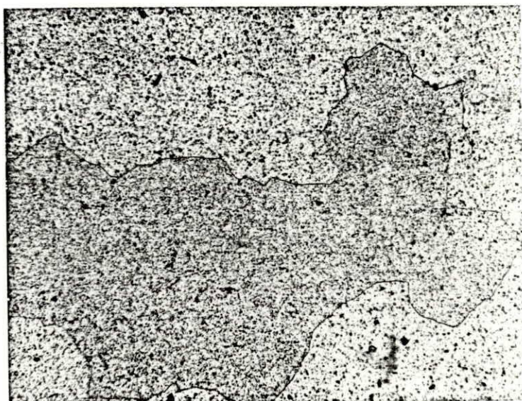
Figura 5-30. .- Microestructura de una probeta extruída y enfriada al agua; posteriormente solubilizada a 570°C durante 1 - hora y enfriada en agua
