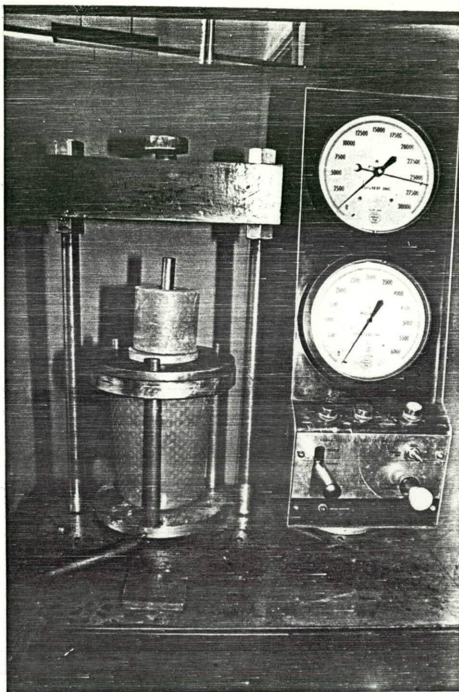
Figura 5-4.- Equipo utilizado en el proceso de extrusión
