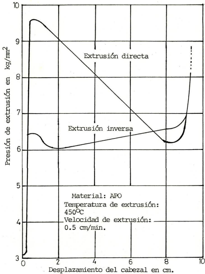
Figura 3-3.- Diagrama de la presión específica, en el caso de la extrusión directa y en el de la extrusión inversa.
