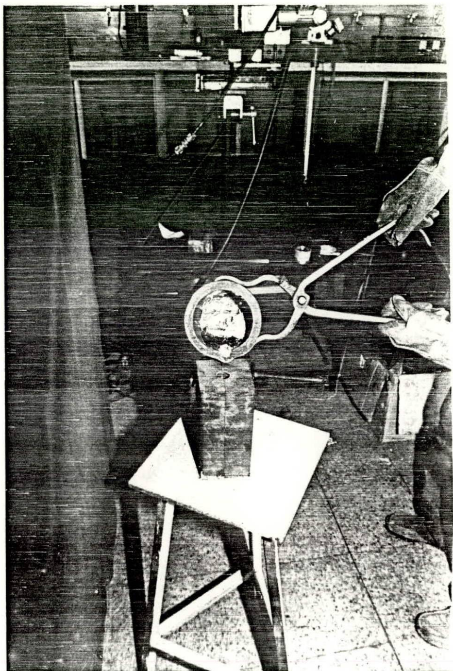
Figura 5-2.- Colada del material fundido en una lingotera precalentada a 250 C.
