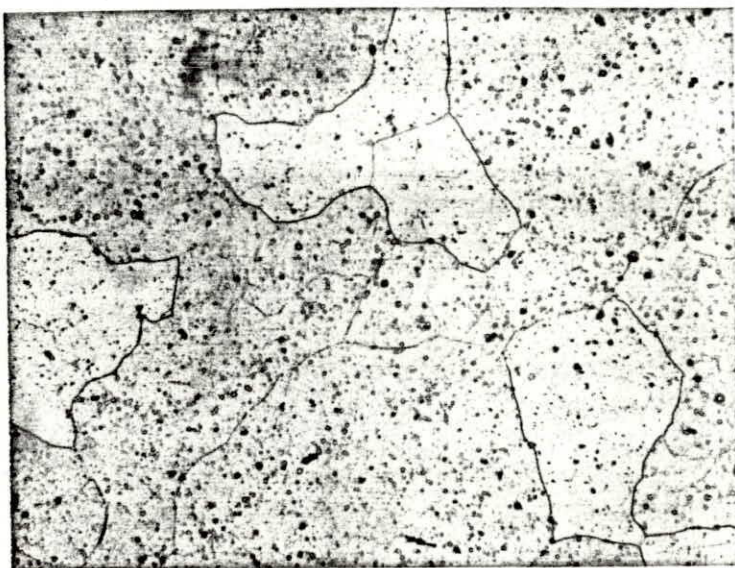
Figura 5-33.- Microestructura de una probeta extruída y enfriada al agua; posteriormente solubilizada a 570^{\circ}\text{C} durante 1 - hora y enfriada al agua; envejecida a 160^{\circ}\text{C} durante - 24 horas
