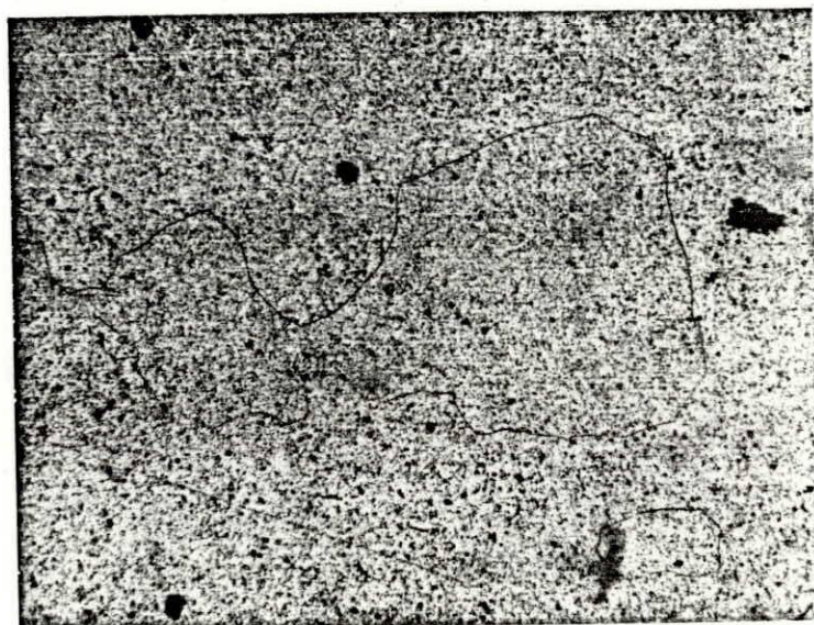
Figura 5-35.- Microestructura de una probeta extruída y enfriada al agua; posteriormente envejecida a 160^{\circ}\text{C} durante 6 horas
