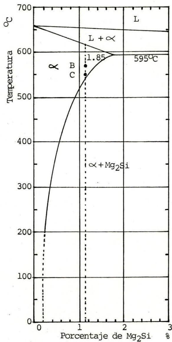
Figura 5-23. - Calentamiento uniforme hasta - una solución sólida completa -- α en el punto B. Disipación del calor a través del alambón (C)
