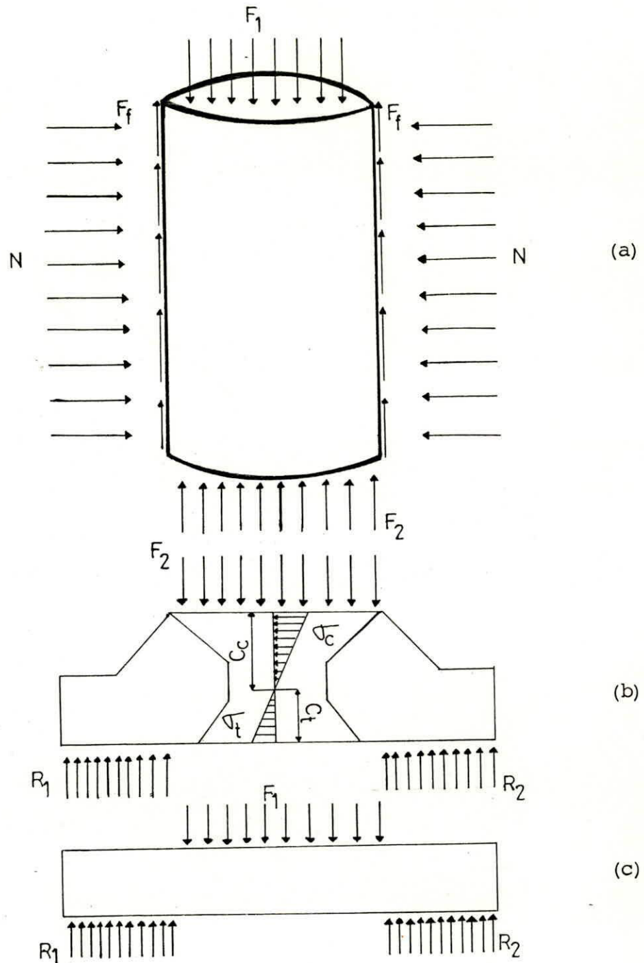
Figura 5-7.- Diagrama de cuerpo libre de las fuerzas que actúan en la matriz y el tocho
