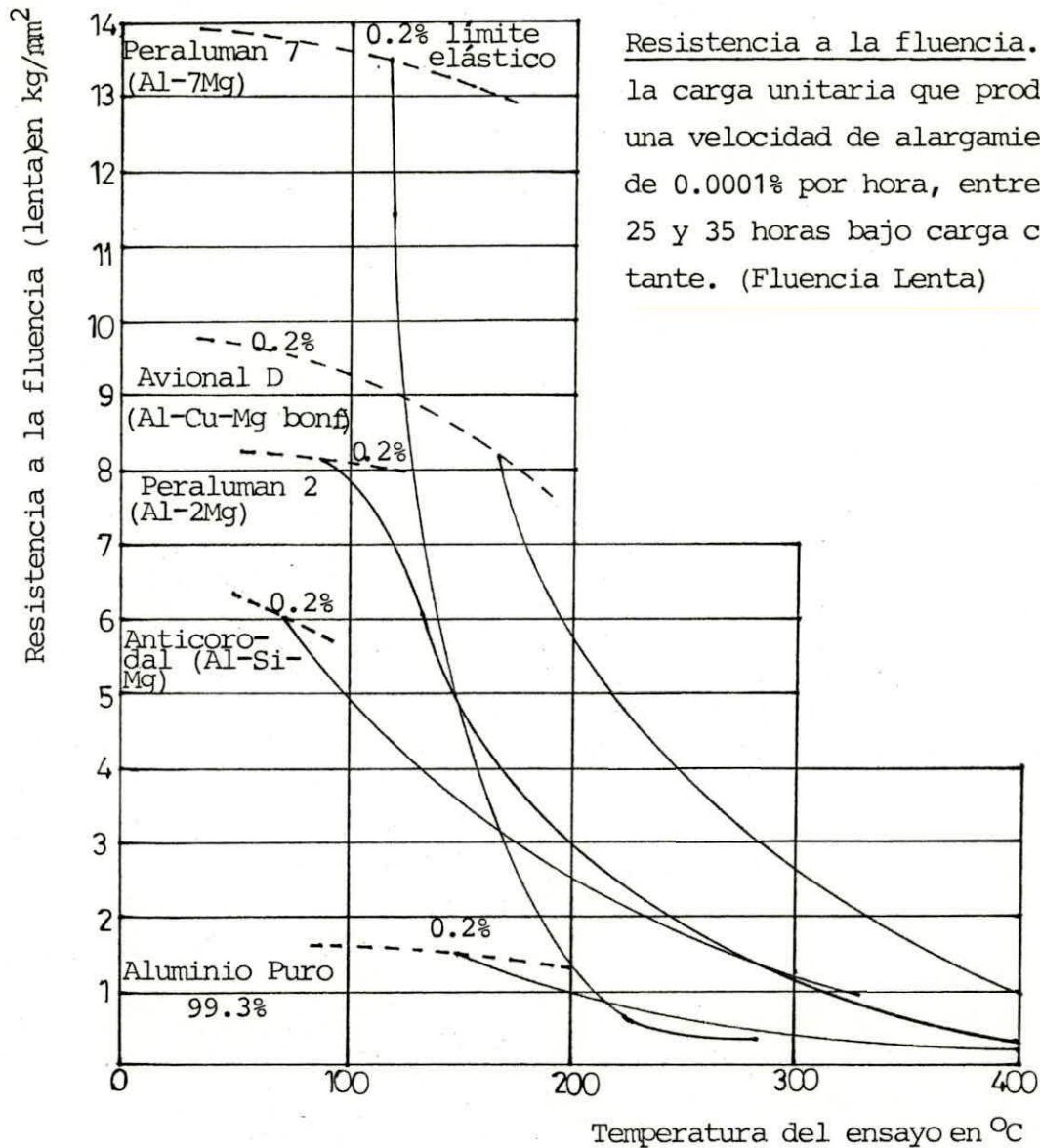
Figura 2-9.- Resistencia a la fluencia a temperaturas elevadas de aleaciones forjadas de Aluminio estabilizadas.
