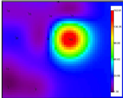
Gráfico 13 Acercamiento en el Mapa de Estimación de la Zona de alta Captura. 2003-2004.
