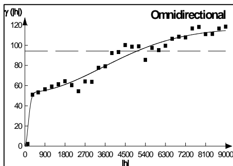
Gráfico 10 Semivariograma y Modelo Ajustado Capturas. 2003-2004
