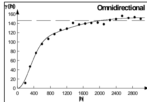
Gráfico 1 Semivariograma y Modelo Ajustado Capturas. 2002-2003
