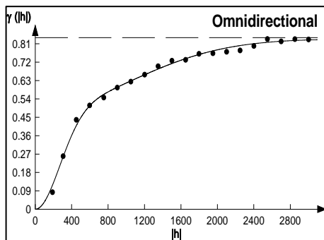
Gráfico 8 Semivariograma y Modelo Ajustado Intensidad. 2002-2003
