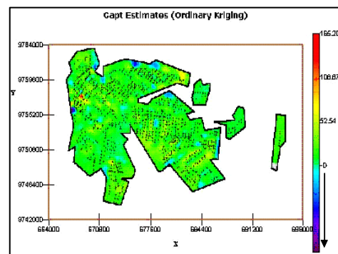
Gráfico 2 Mapa de Estimaciones Capturas. 2002-2003
