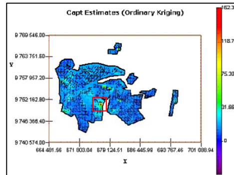
Gráfico 11 Mapa de Estimaciones Capturas. 2003-2004
