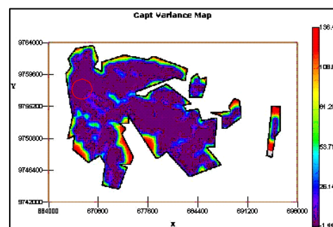
Gráfico 3 Mapa de Varianza Capturas. 2002-2003
