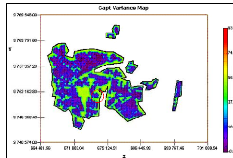
Gráfico 12 Mapa de Varianza Capturas. 2003-2004
