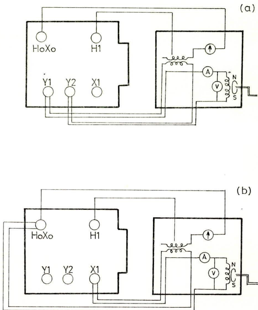
FIG.4.- MEDIDA DE LA RELACION DE TRANSFORMACION
