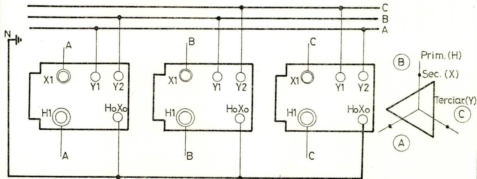
FIG. 1.- CONEXIONADO GENERAL DEL BANCO TRIFASICO
