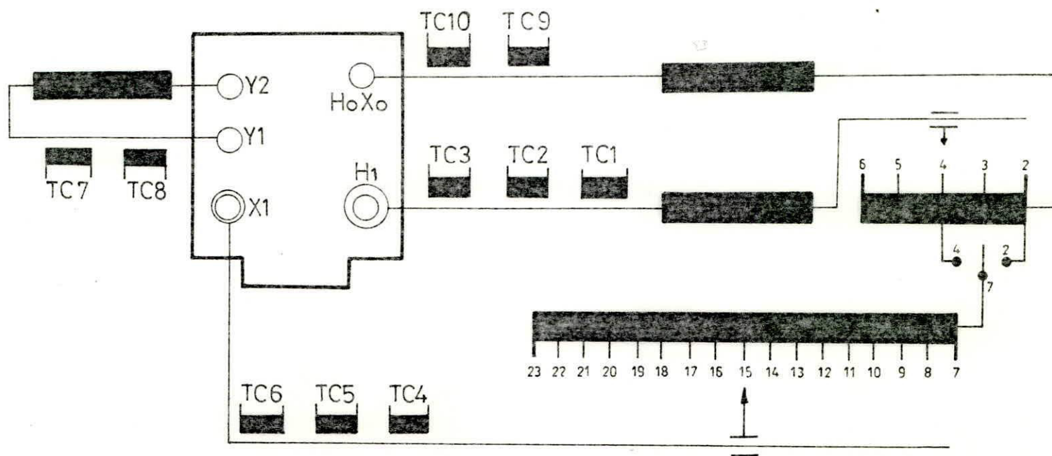
FIG. 2.- UBICACION DE BOBINAS Y TC'S. DESARROLLO INTERNO DE CONEXIONES
