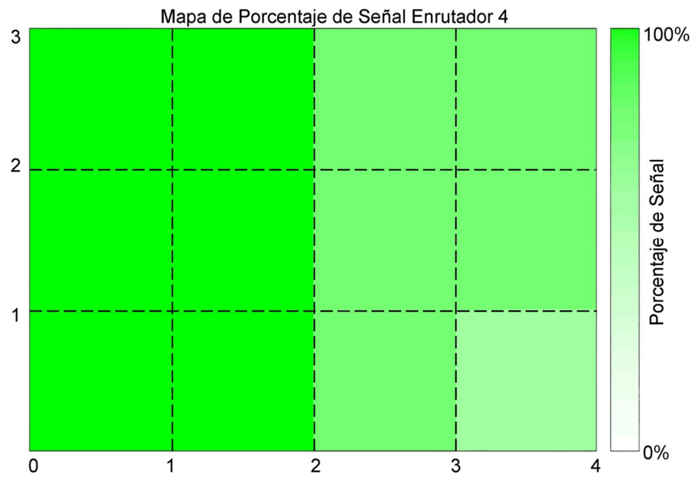
Fig. 4.10 Mapa de Porcentaje de señal Enrutador 4
