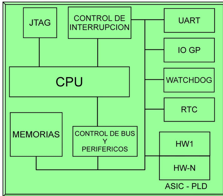
Fig. 2.10 Arquitectura de un Sistema Embebido
