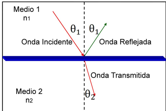
Fig. 2.5 Desvío de la onda al pasar de un medio a otro
