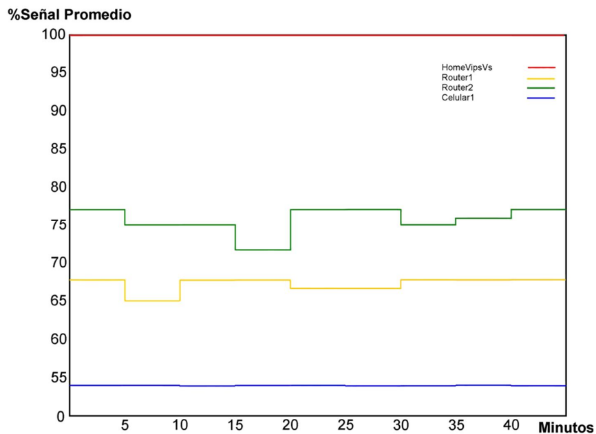
Fig. 4.2 Gráfico Porcentaje de la señal promedio vs tiempo
