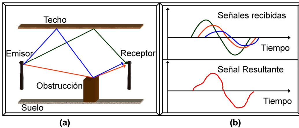
Fig. 2.7 Propagación en multitrayectoria (a) Multitrayectoria entre el emisor y receptor (b) Efecto en el tiempo y en la onda resultante de la propagación en multitrayectorias
