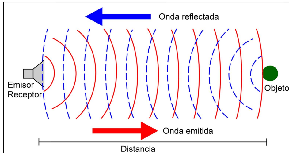
Fig. 2.4 Reflexión de las ondas
