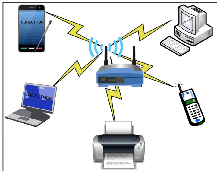
Fig. 2.1 Dispositivos Wi-Fi
