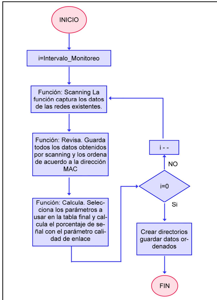
Fig. 3.5 Diagrama de flujo del script de monitoreo
