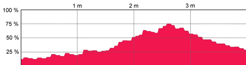
Fig. 4.4 Gráfico carga del procesador del enrutador durante la ejecución
