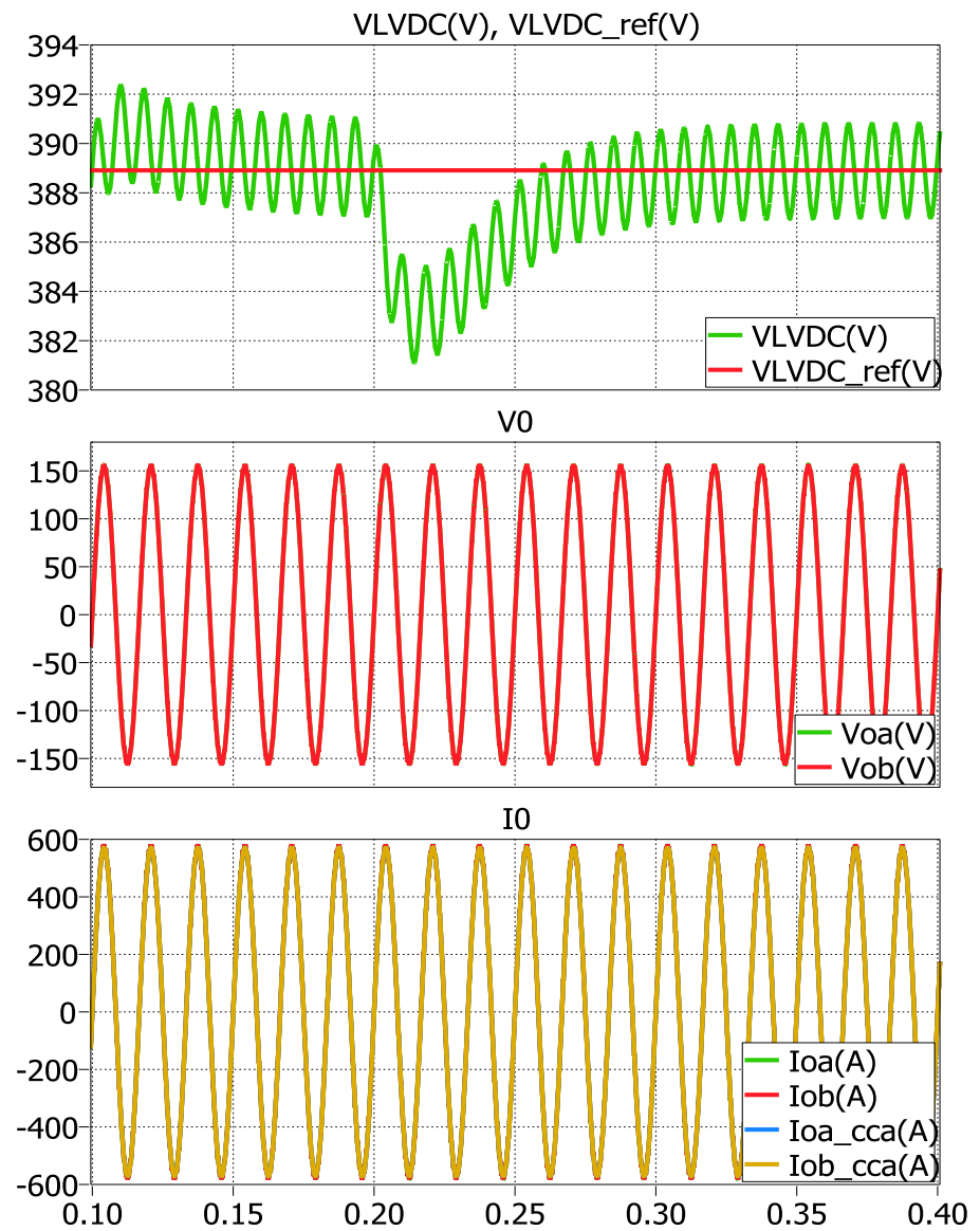
Fig. 5.10. Voltajes LVDC, voltaje de salida del inversor y corrientes de salida del inversor
