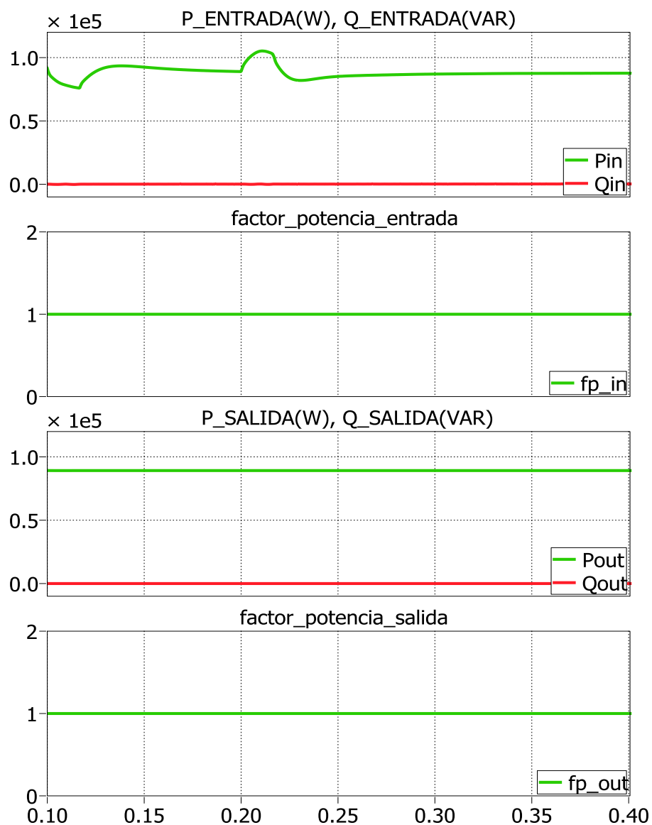
Fig. 5.5. Potencia de entrada y salida, fp de entrada y salida
