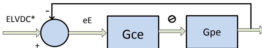
Fig. 4.7 Diagrama de bloque del controlador del DAB.
