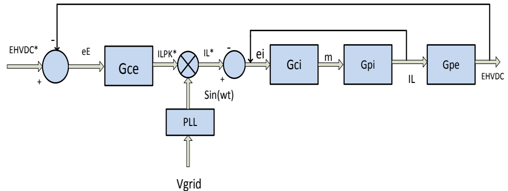
Fig. 4.2. Diagrama de bloque del controlador de la primera etapa AC-DC
