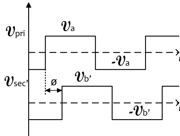
Fig. 2.16 Ondas V_{pri} y V_{sec'} y ángulo de desfase \phi para el calculo de la potencia P.
