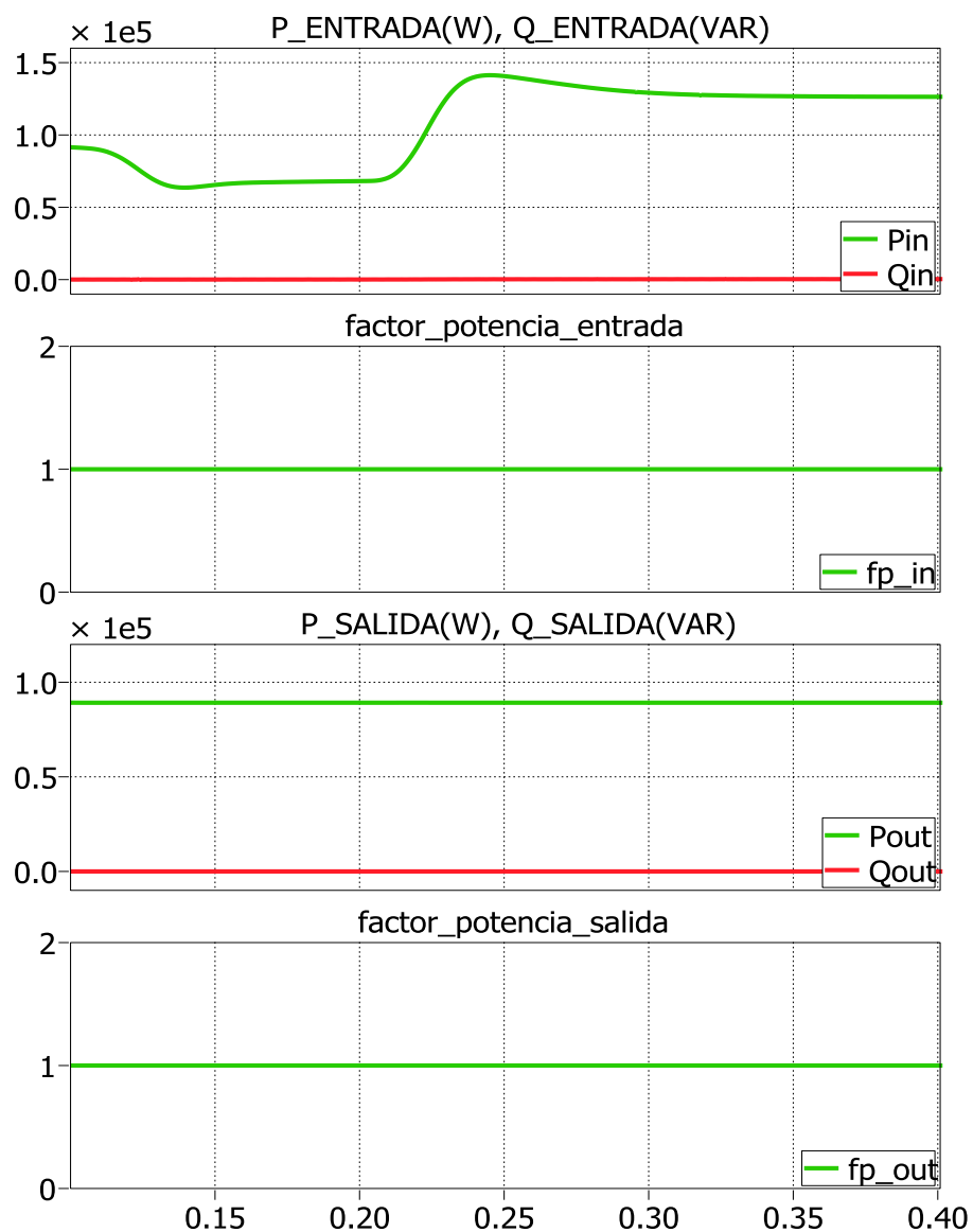
Fig. 5.11. Potencia de entrada y salida, fp de entrada y salida
