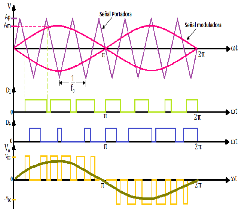
Fig. 2.13 Modulación .por ancho de pulso unipolar.
