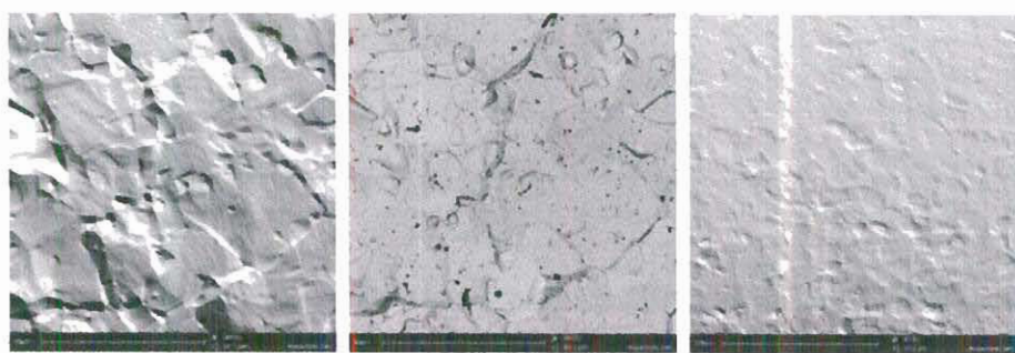
FIGURA 4. 33 Imágenes de SEM del Titanio con Dopamina, reacción de 24 horas por el método de Self Assembly , (a) Topografía B, (b) Imagen completa y (c) Topografía A.
