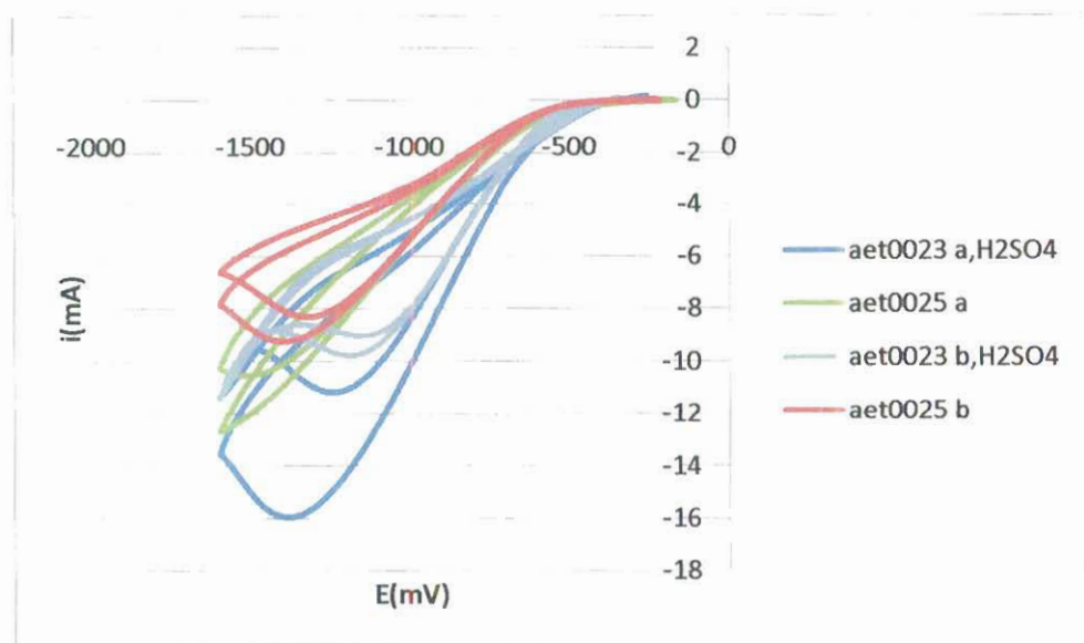
FIGURA 4. 7 Voltamogramas cíclicos registrados en solución acuosa que contiene monómero AEMA, entre Vca y -1.6 V. velocidad de barrido 20 mV/s. AET0023A-B solución con H_2SO_4 . AET0025A-B solución sin H_2SO_4 .
