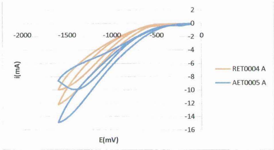
FIGURA 4. 5 Voltamogramas cíclicos registrados en solución acuosa que contiene H 2 SO 4 , entre Vca y -1.6 V. velocidad de barrido 20 mV/s. RET0004A solución sin monómero. AET0005A solución con monómero.
