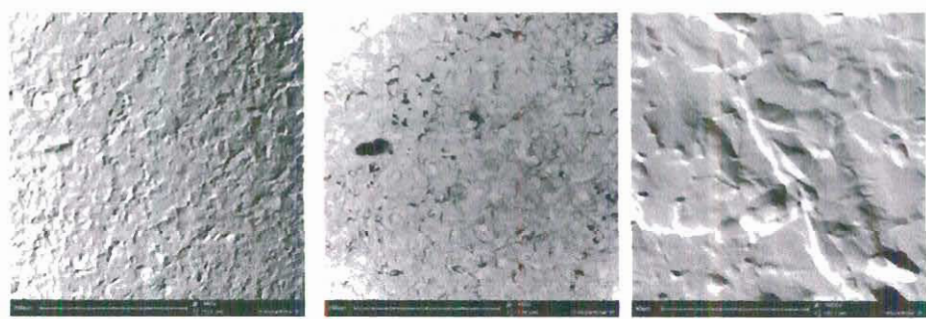
FIGURA 4. 32 Imágenes de SEM del Titanio con Dopamina, reacción de 3 horas por el método de Self Assembly , (a) Topografía B, (b) Imagen completa y (c) Topografía A.
