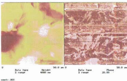
FIGURA 4. 36 Imágenes de titanio comercial en AFM
