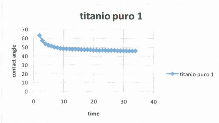
FIGURA 4. 16 Variación del ángulo de contacto en el tiempo para el titanio puro
