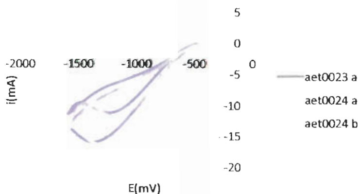
FIGURA 4. 6 Voltamogramas ciclicos registrados en solución acuosa que contiene monómero AEMA, entre Vca y -1.6 V. velocidad de barrido 20 mV/s. AET0023A-B 5 barridos de 2 ciclos. AET0024A 10 barridos de un ciclo.
