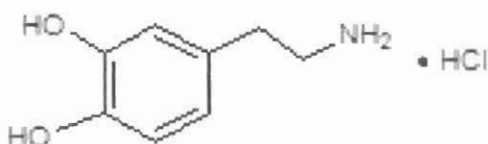
Figura 1. 10 Molécula de dopamina
