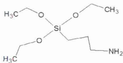
FIGURA 1. 5 Fórmula Molecular de APTES
