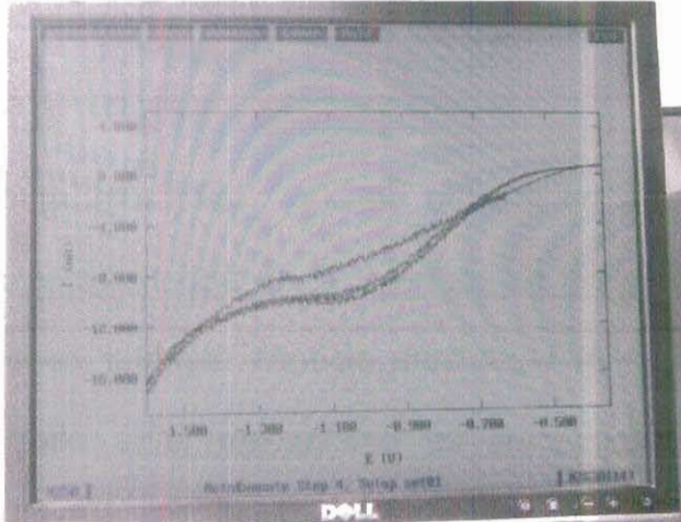
Figura 3. 7 Voltamograma en ejecución del programa M 270.
