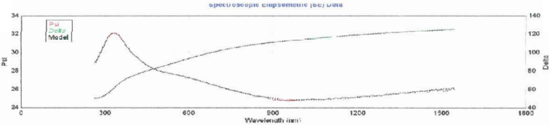
FIGURA 4. 55 Ajuste de curva del titanio referencial para la primera medición
