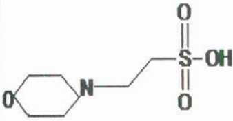
Figura 1. 12 MES: Ácido 2-(N-morfolina) etanosulfónico
