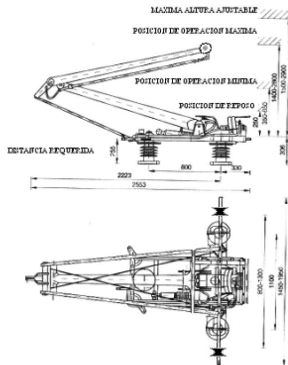
Fig. 2.3 (6) Pantógrafo DSA-350S
