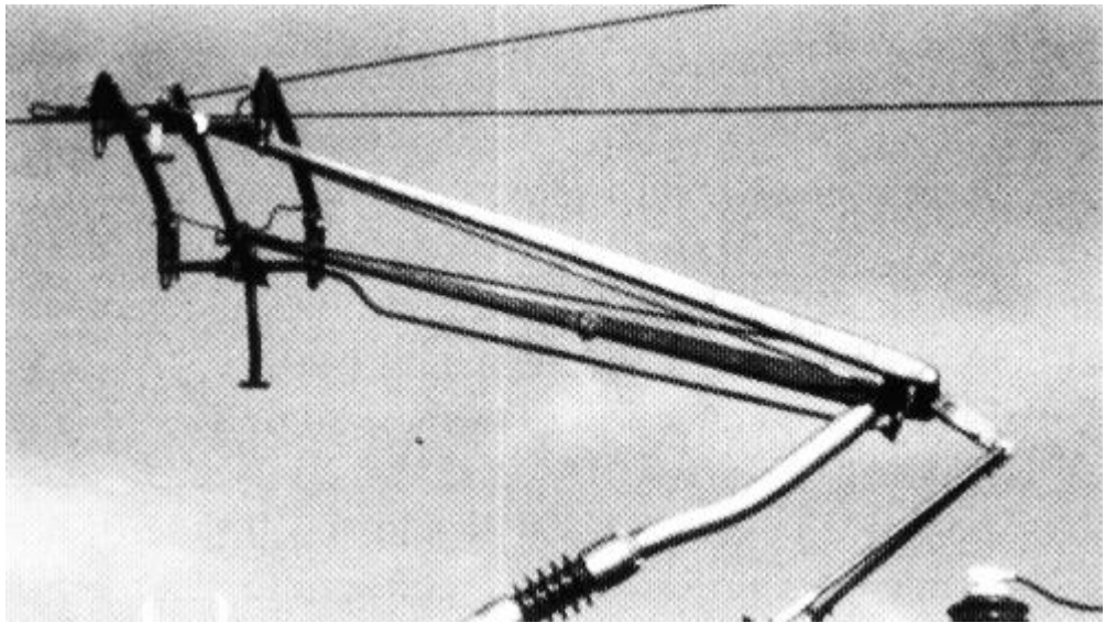
Fig. 2.8 (6) Pantógrafo DSA-350S
