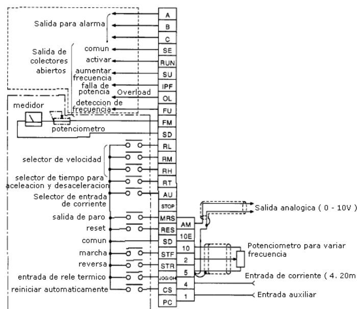
Fig. 3. 19 Grafico del Circuito de Control del Inversor
