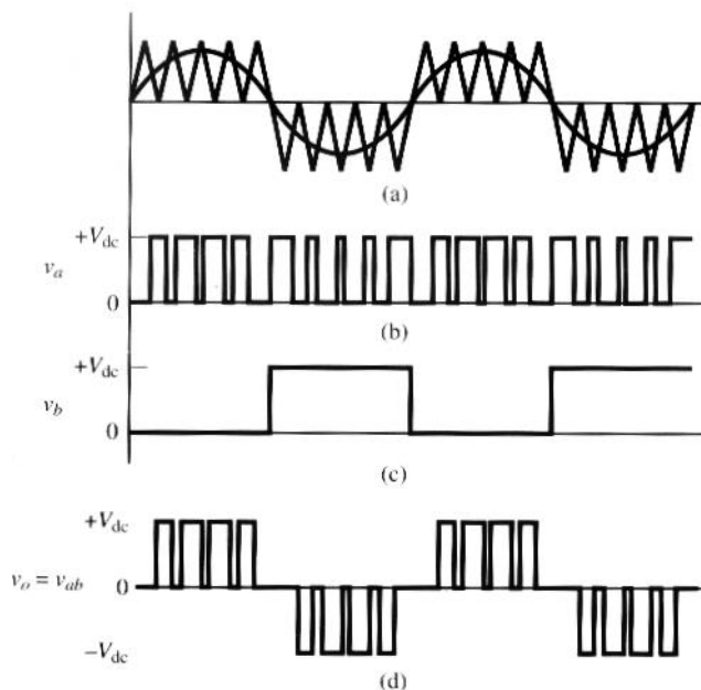
Fig. 1.11 (2) PWM Unipolar con interruptores de alta y baja frecuencia (a) Señal de Control y Referencia (b) v_a (c) v_b (d) Salida v_a - v_b
