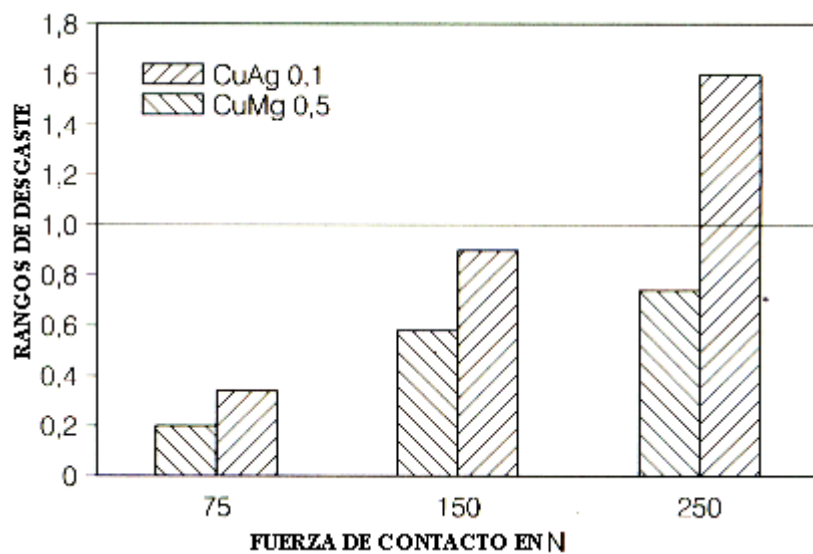
Fig. 2.11 (6) Rangos de Desgaste vs Fuerza de Contacto
