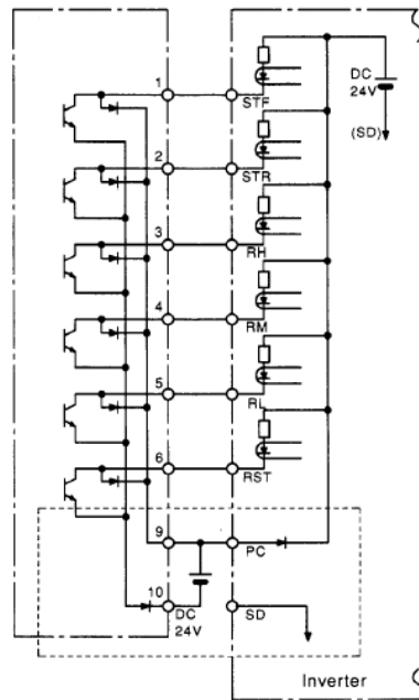
Fig. 3. 20 Gráfico del Esquema de los Transistores del Inversor
