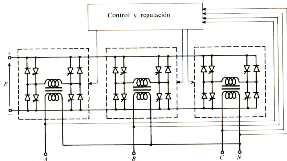
Fig. 1.18 (3) Ondulador Trifásico
