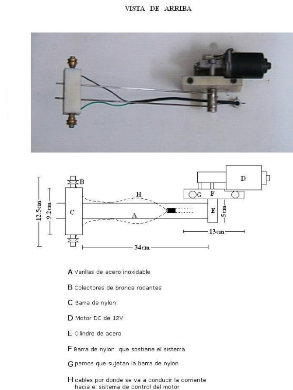
Fig. 3. 14 Vista Superior del Pantógrafo con sus Respetivos Elementos
