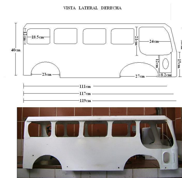
Fig. 3. 5 Vista Lateral Derecha de la Carrocería del Bus
