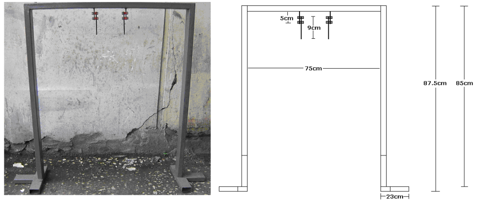
Fig. 3. 2 Arcos que Sostienen las Líneas de Tensión
