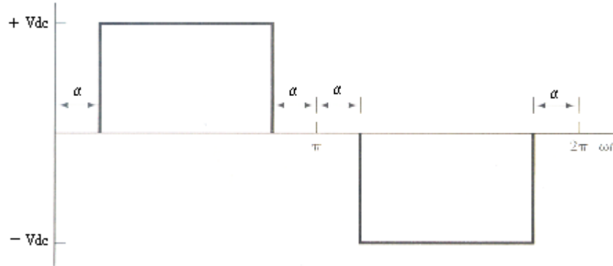
FIG. 1.9 Forma de Onda del Voltaje de Salida con Angulo de Control
