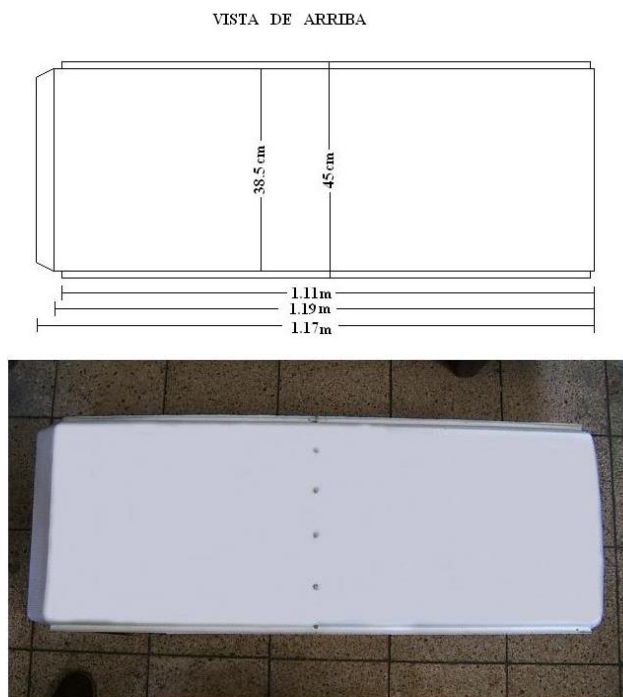
Fig. 3. 4 Vista Superior de la Carrocería del Bus
