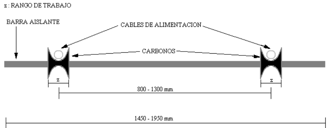
Fig. 2.4 Vista Frontal del Pantógrafo
