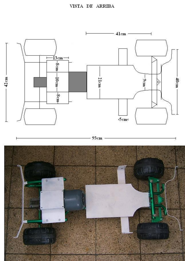
Fig. 3. 8 Vista Aérea del chasis del bus
