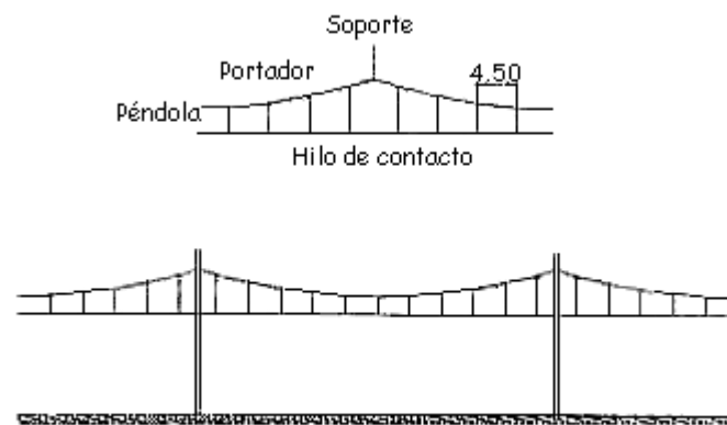
Fig. 2.23 (6) Catenaria Ligera
