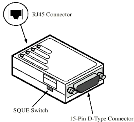
FIGURA 4.10 CONVERTIDOR AUI-RJ45
