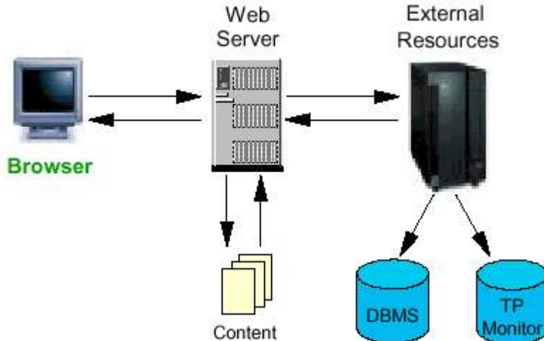
Figura 7.1: Componentes de una aplicación Web.
