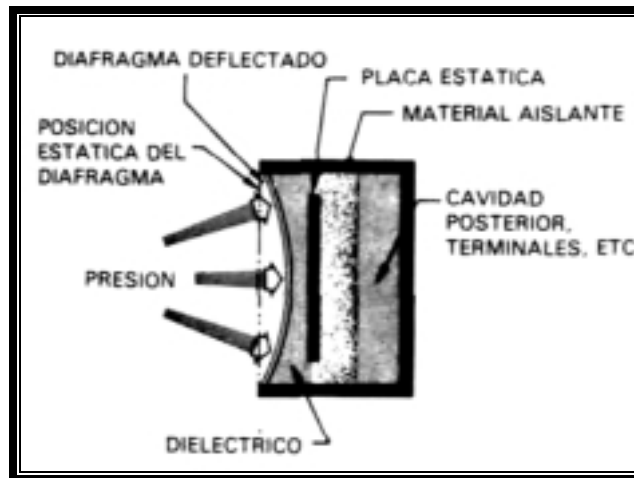
Figura 1.6 Transductor capacitivo
