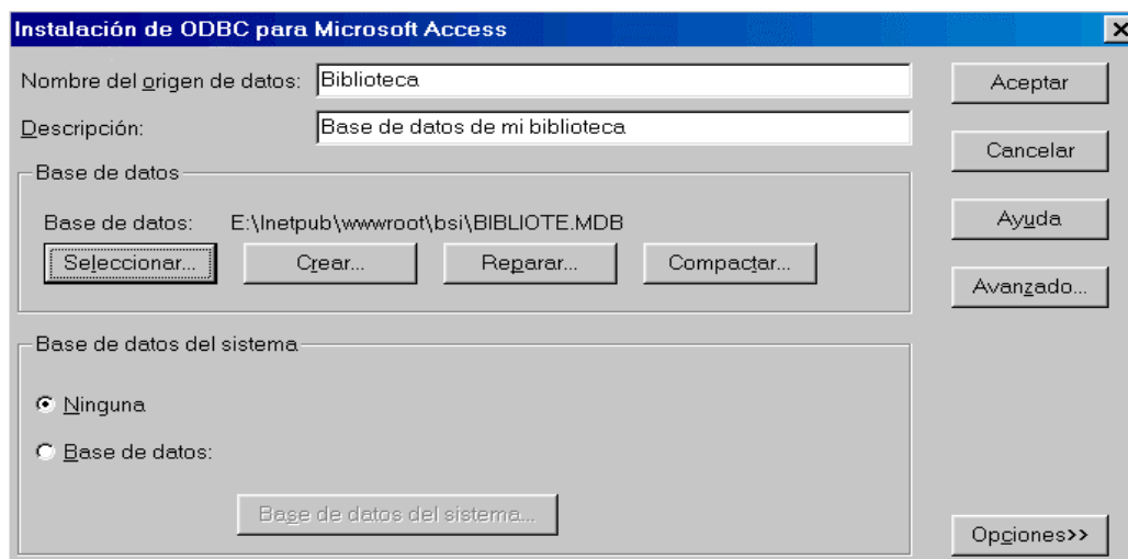
Figura 4.3 Instalación ODBC
