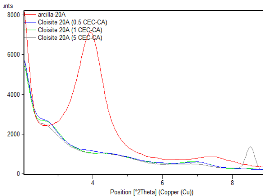
Figura 4.4: Difractograma de Cloisite 20A
