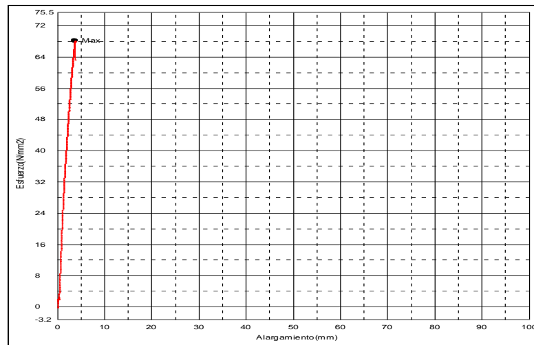
Figura 4.45: Relación: Esfuerzo y Alargamiento Fuente: Burgos O., Chávez M., Vera G.
