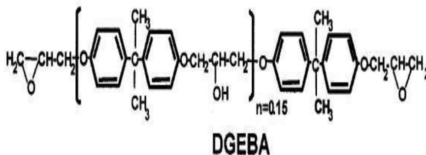
Figura 3.6: Estructura química de la resina EPON828
