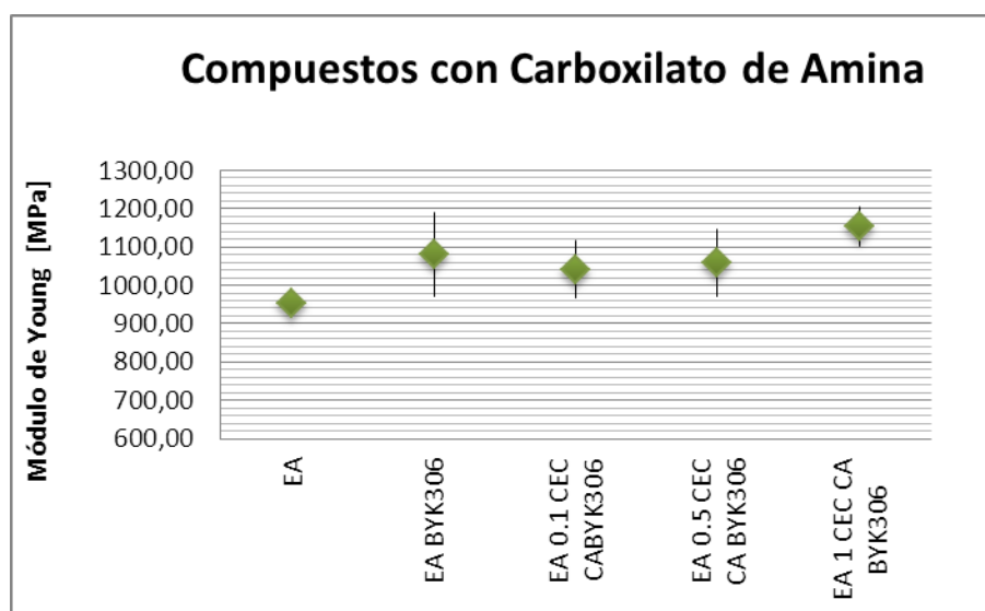
Figura 4.47: Módulo de Young de los compuestos con carboxilato de amina
