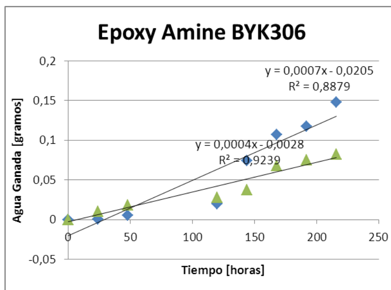
Figura 4.53: Agua ganada vs tiempo: EA BYK306
