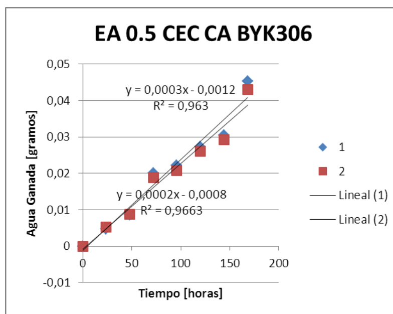
Figura 4.55: Agua ganada vs tiempo: EA 0.5 CEC CA BYK306
