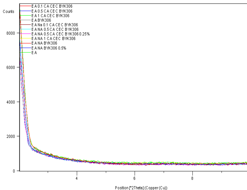
Figura 4.5: Difractograma de los nanocompuestos con Cloisite Na
