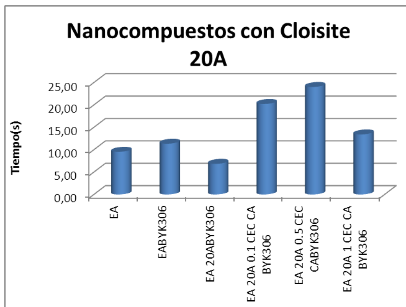
Figura 4.87: Tiempo consumido para los nanocompuestos con Cloisite 20A
