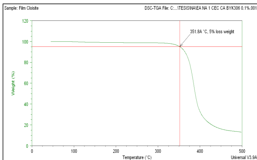
Figura 4.39: Temperatura de descomposición y porcentaje de pérdida de peso: EA Na 1 CEC CA BYK306
