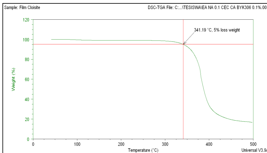
Figura 4.37: Temperatura de descomposición y porcentaje de pérdida de peso: EA Na 0.1 CEC CA BYK306 Fuente: Burgos O., Chávez M., Vera G.
