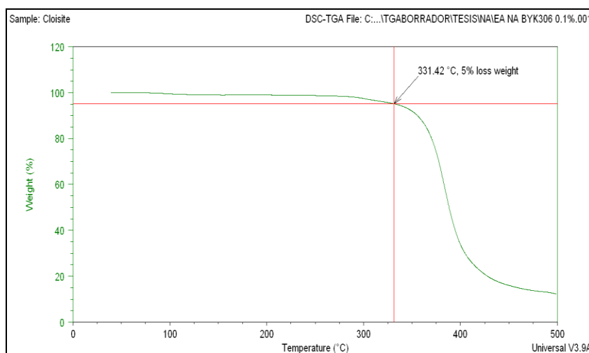
Figura 4.36: Temperatura de descomposición y porcentaje de pérdida de peso: EA Na BYK306 Fuente: Burgos O., Chávez M., Vera G.
