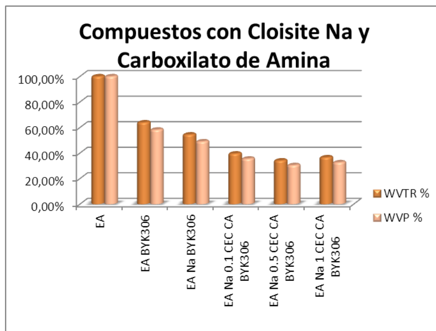
Figura 4.67: WVTR y WVP del compuesto con Cloisite Na
