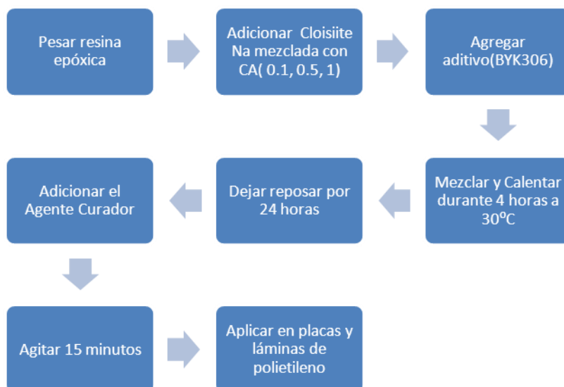
Figura 3.62: Proceso de preparación de compuestos # 7, 8 y 9 de mezclas con Cloisite Na
