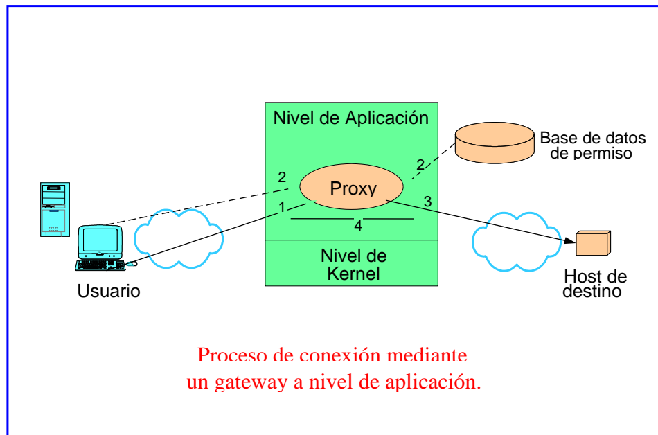
FIG. 2.8 Gateway a nivel de aplicación.
