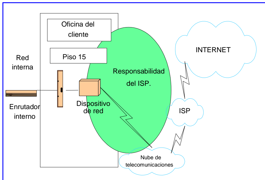
FIG. 3.14 Zonas de la solución no claramente definidas por el ISP
