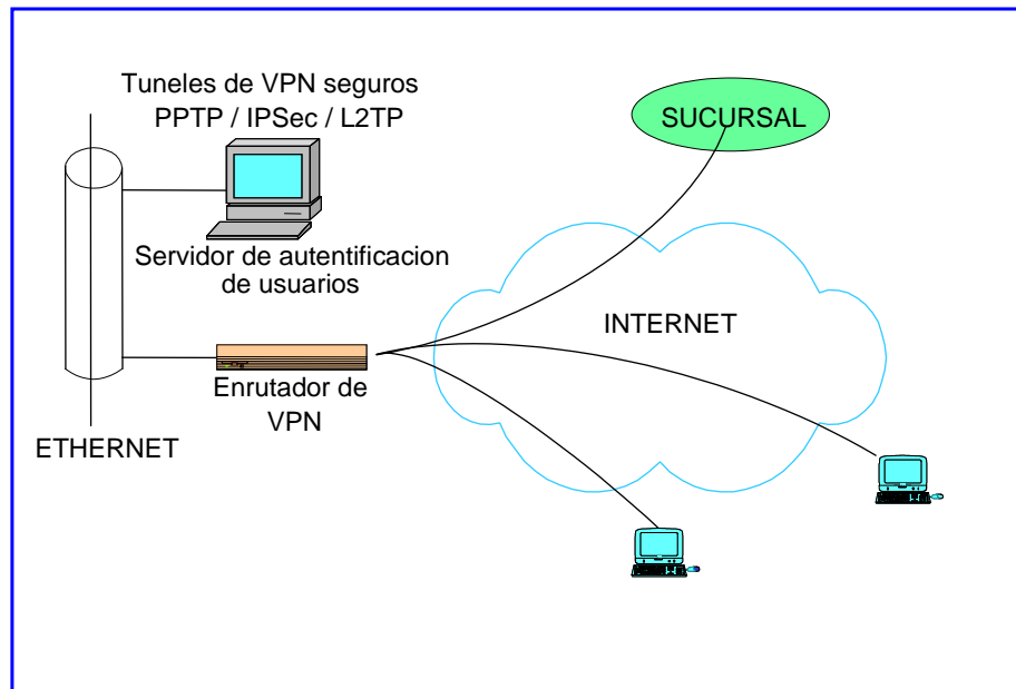
FIG. 3.17 VPN basada en enrutador.
