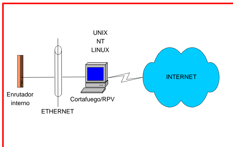
FIG. 3.15.- VPN basada en cortafuego.
