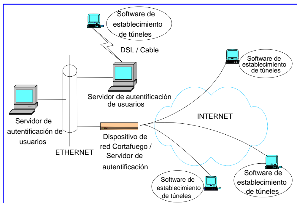
FIG. 3.18 Escenario de acceso remoto.
