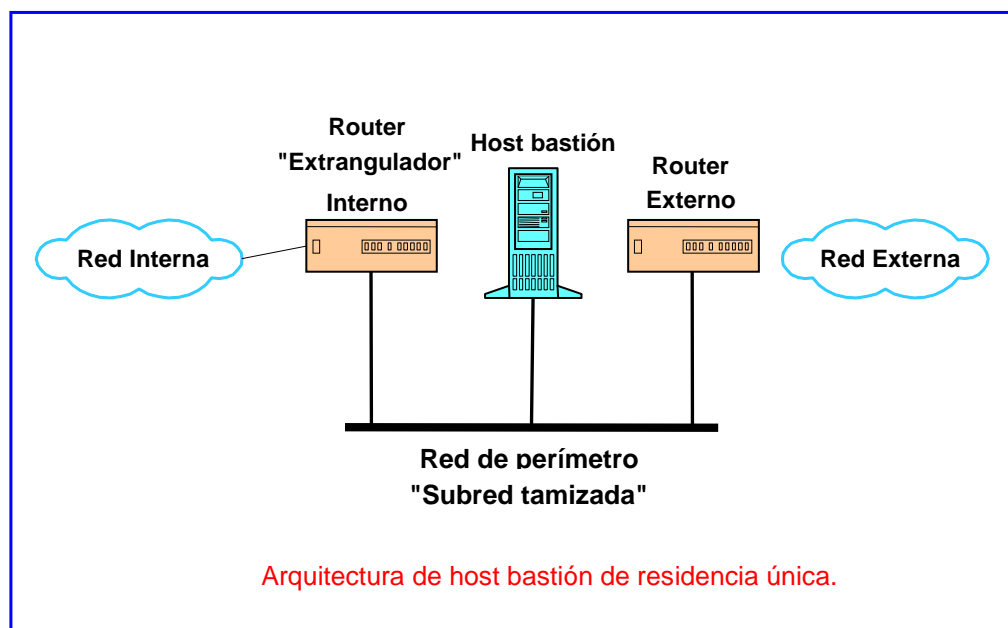
FIG. 2.5 Cortafuegos basados en un host Bastión.
