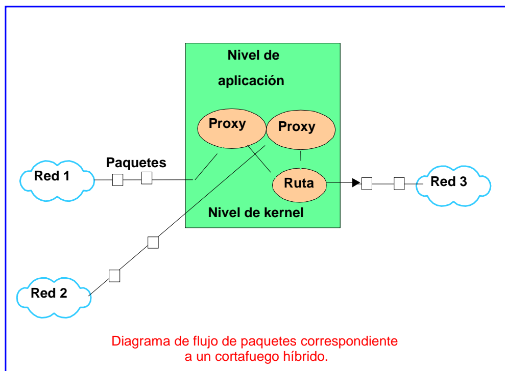
FIG. 2.4 Cortafuegos híbridos.
