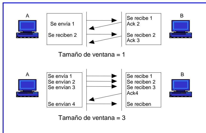
FIG. 1.15.- Confiabilidad con ventanas.
