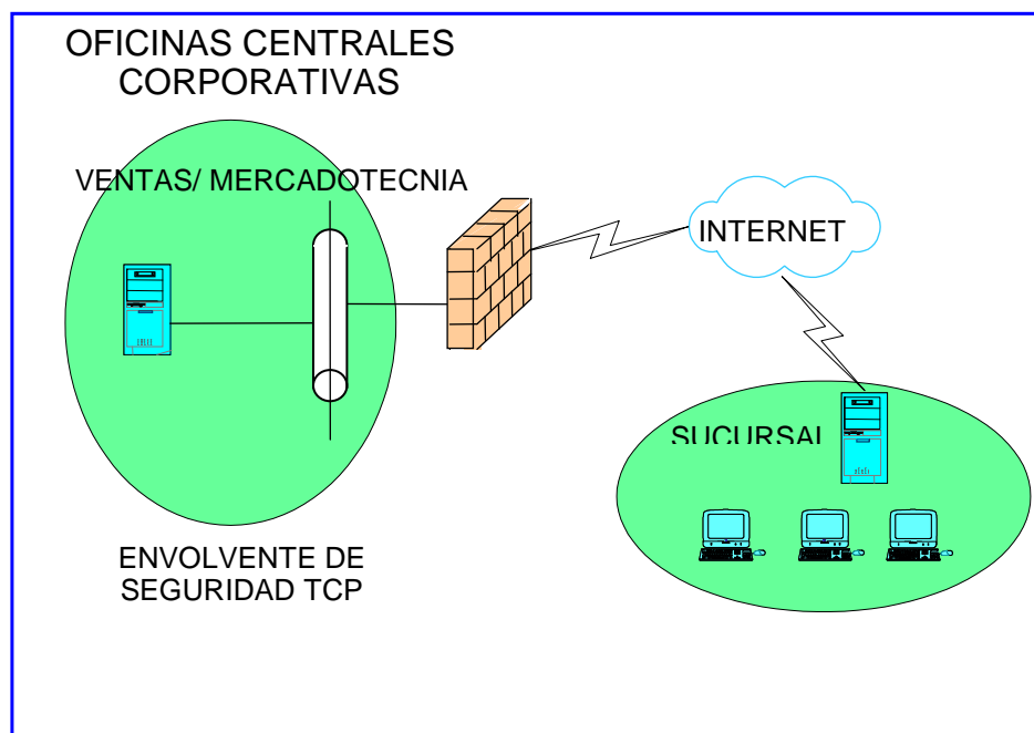
FIG. 3.2 VPN corporativa con sistema mainframe heredado.
