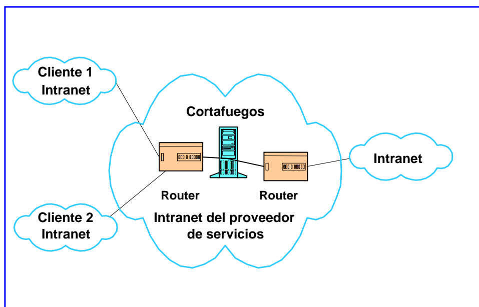
Fig.2.6 Cortafuegos Basados en Redes.
