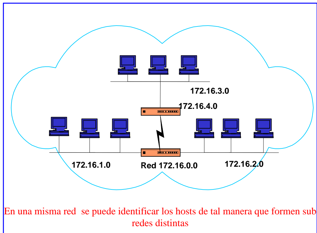
FIG. 1.13.- Direccionamiento con subredes.
