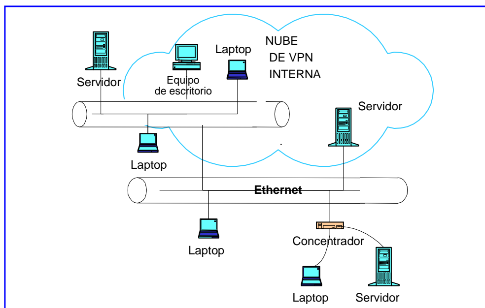
FIG. 3.6 Una VPN interna.
