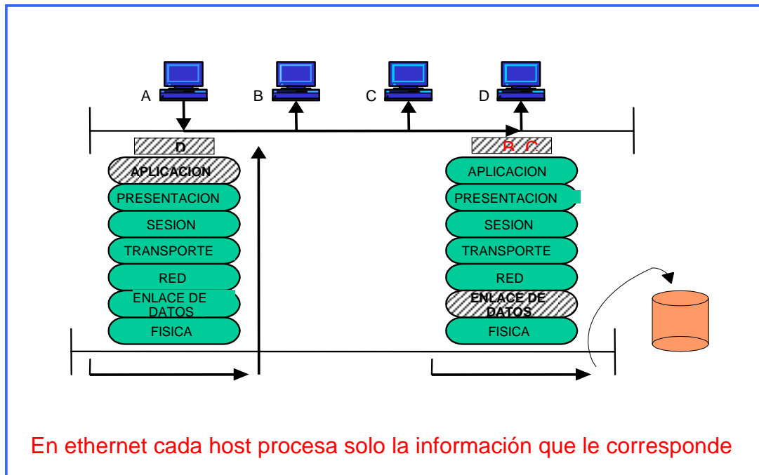
FIG. 1.8 Operación de Ethernet/802.3
