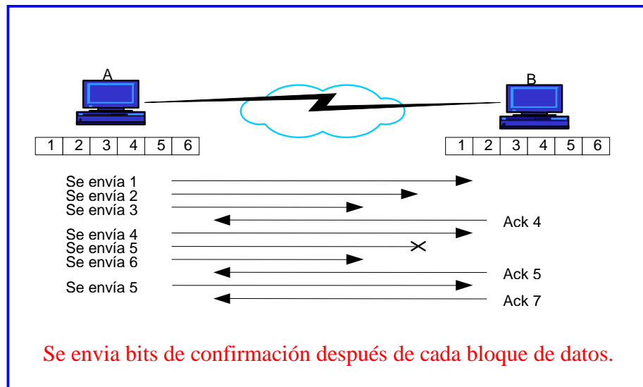
FIG. 1.16.- Técnica de acuse de recibo.
