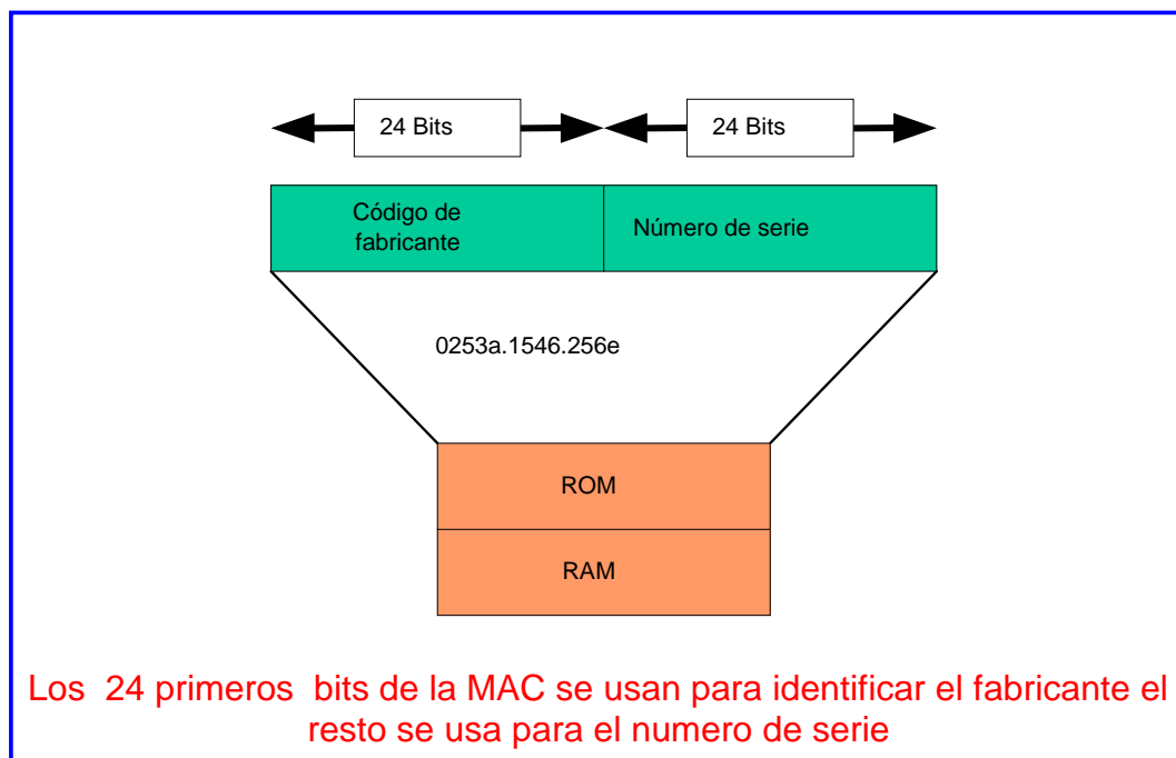
FIG. 1.11 Direccionamiento MAC.
