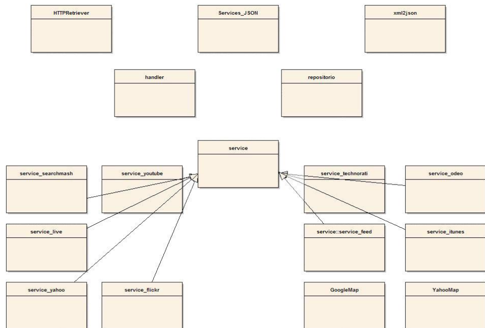
Figura 3.7: Diagrama Simplificado de Clases.
