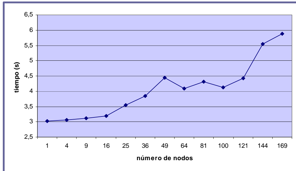
Fig 5.28: Tiempo de convergencia con tráfico al 10%
