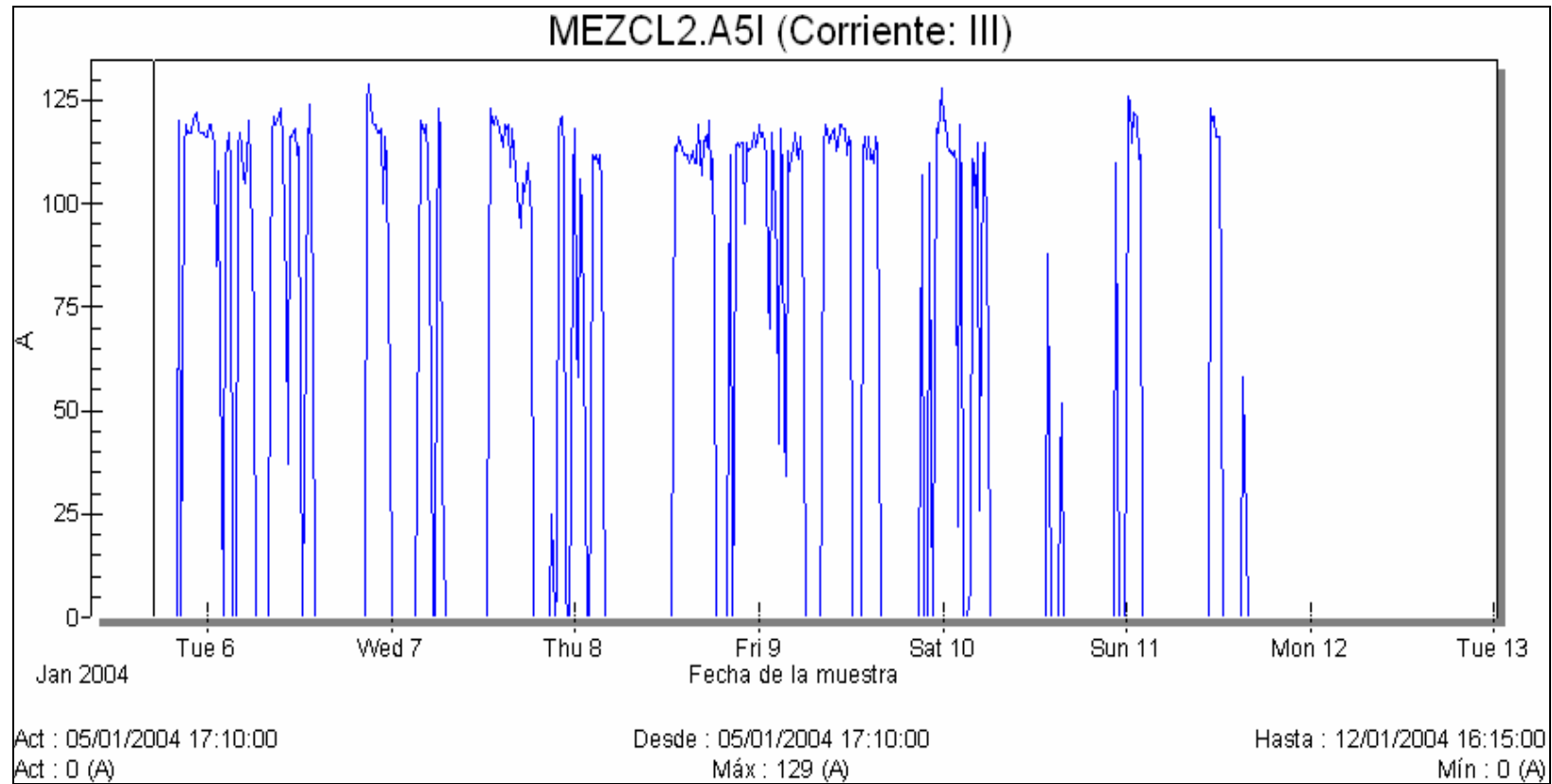
Figura 3.18 Variaciones de la corriente trifásica de Mezclado
