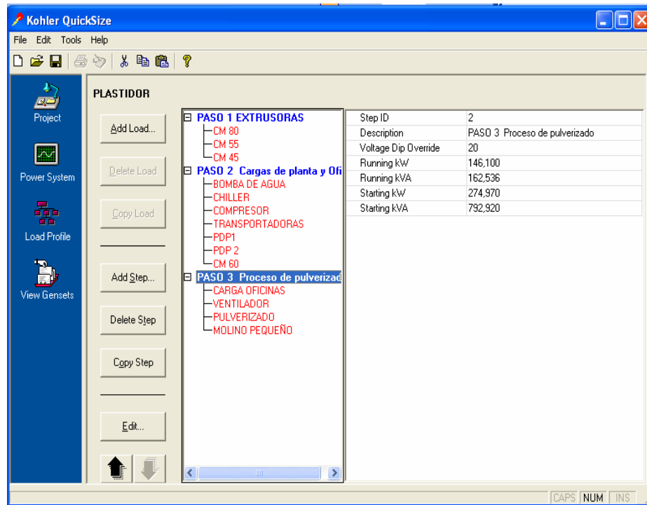
Figura 7.4 Pantalla de distribución de cargas del Software Kohler Quick Size
