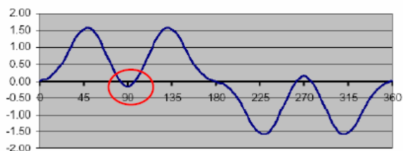
Figura 5.2 Distorsión armónica de corriente
