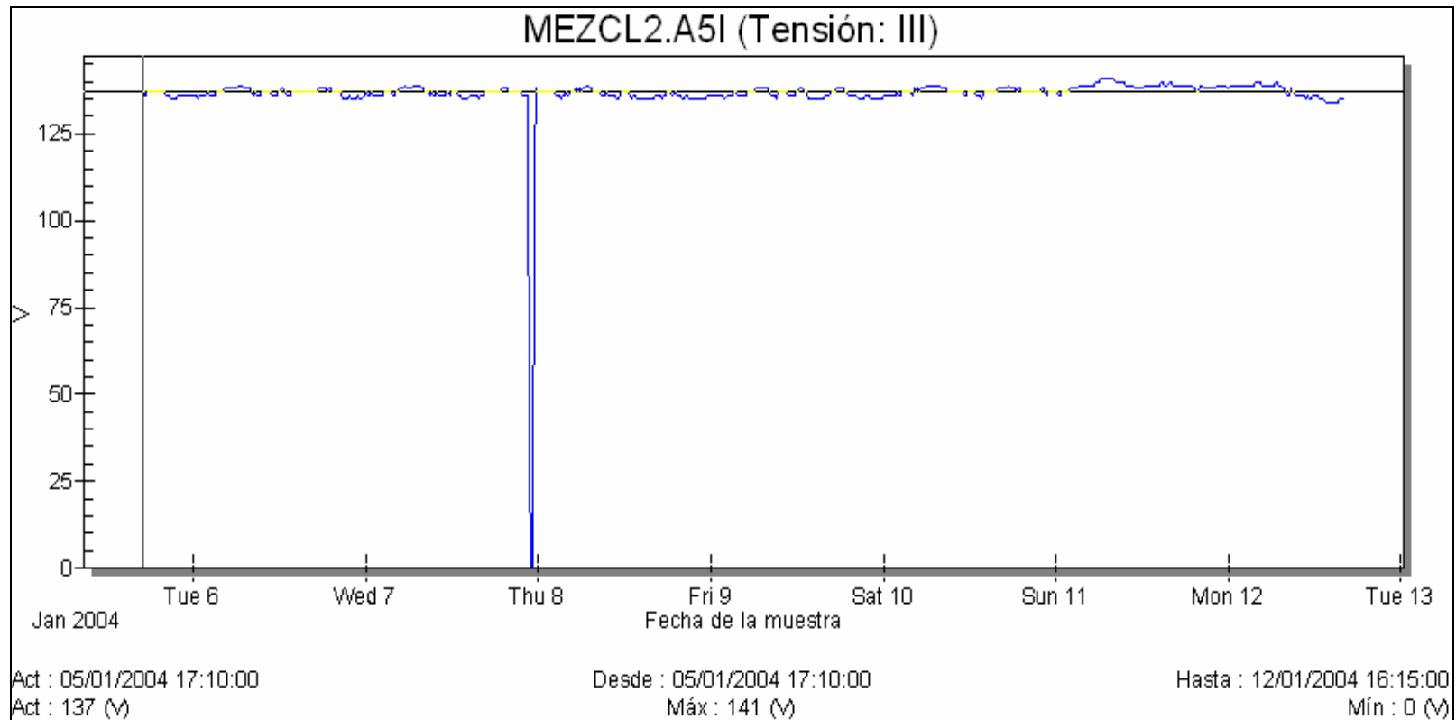
Figura 3.17 Variaciones del voltaje trifásico de Mezclado
