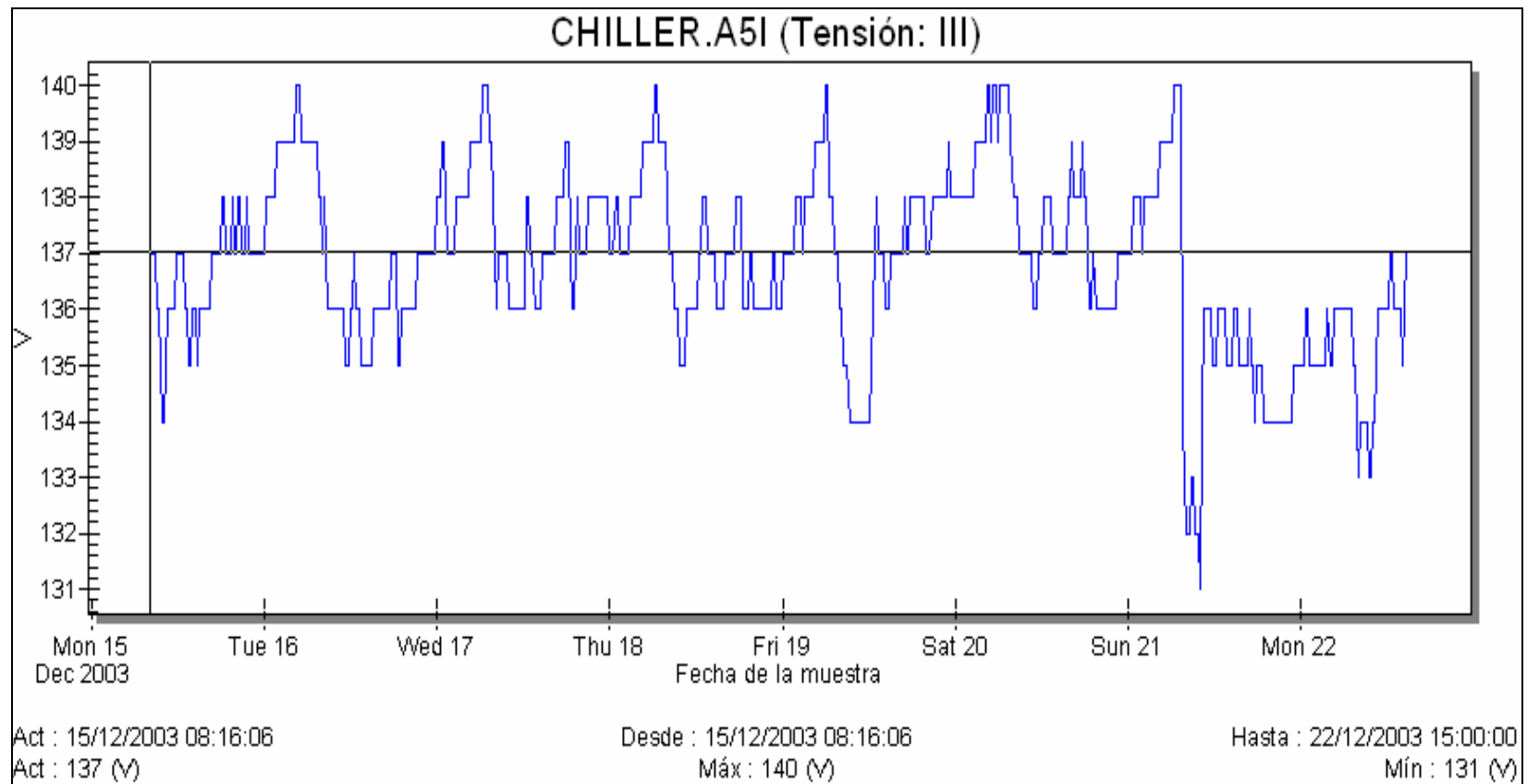
Figura 3.11 Variaciones del voltaje trifásico de Chiller
