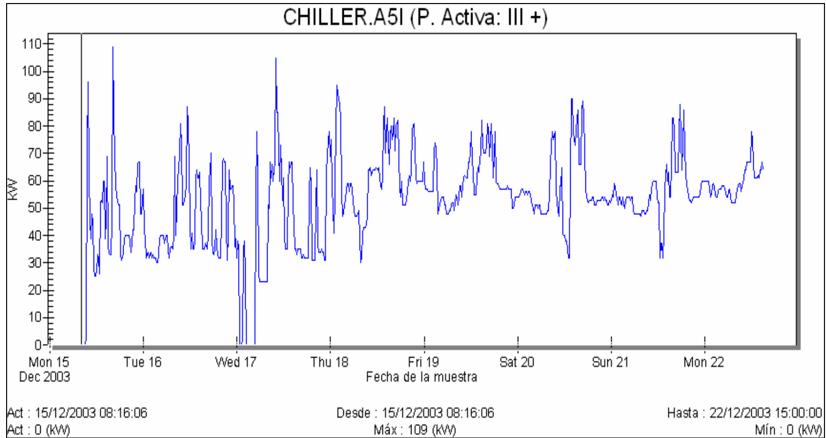
Figura 3.13 Variaciones de la potencia activa de Chiller
