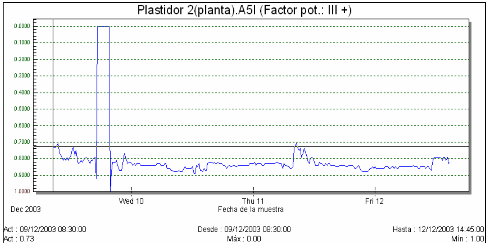
Figura 3.9 Variaciones del factor de potencia de Planta
