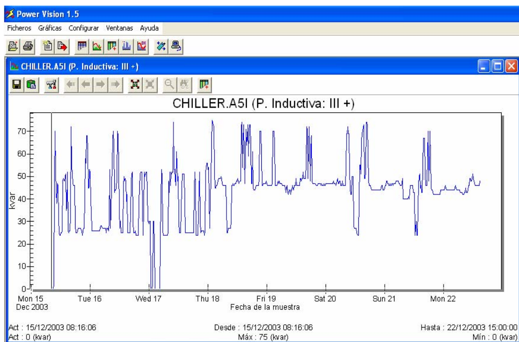
Figura 3.2 Visualización del Software Power Vision – Potencia Inductiva
