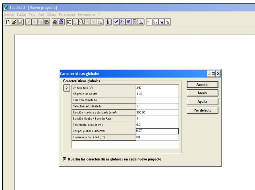
Figura 4.1 Ecodial: Tabla de datos generales requeridos.
