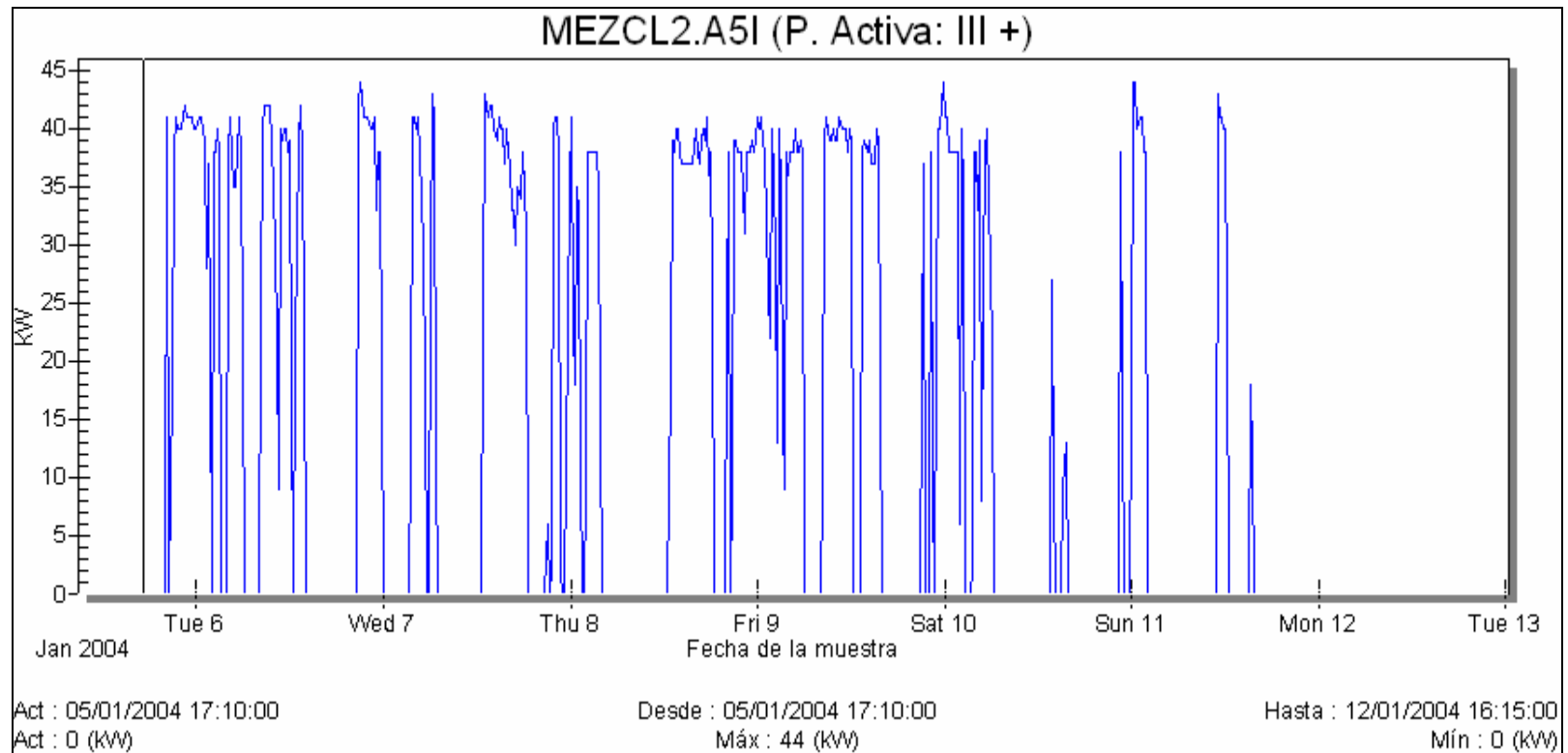
Figura 3.19 Variaciones de la potencia activa de Mezclado
