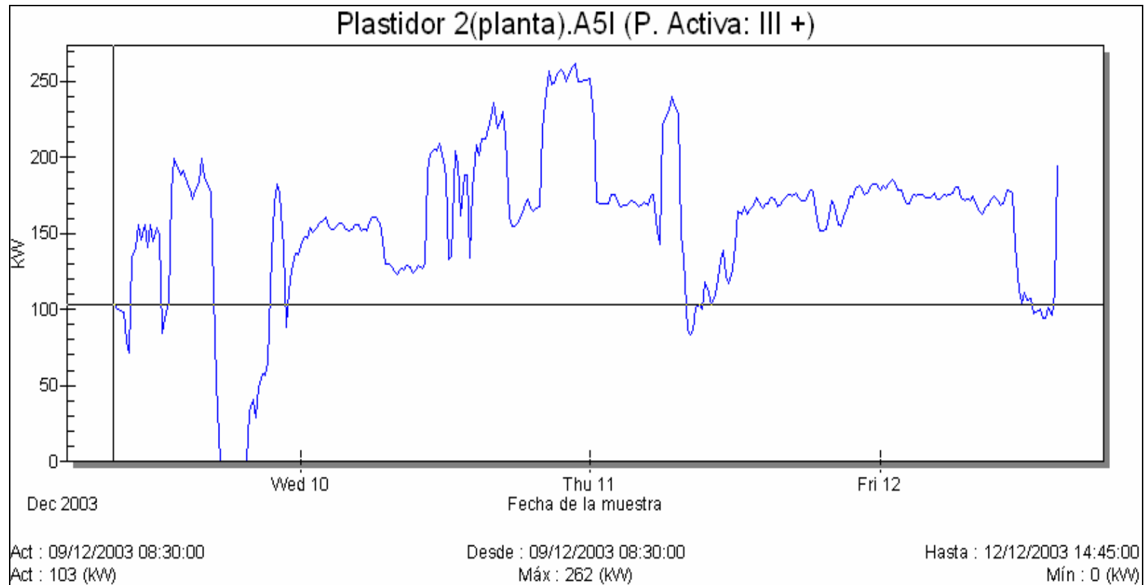
Figura 3.7 Variaciones de la potencia activa de Planta
