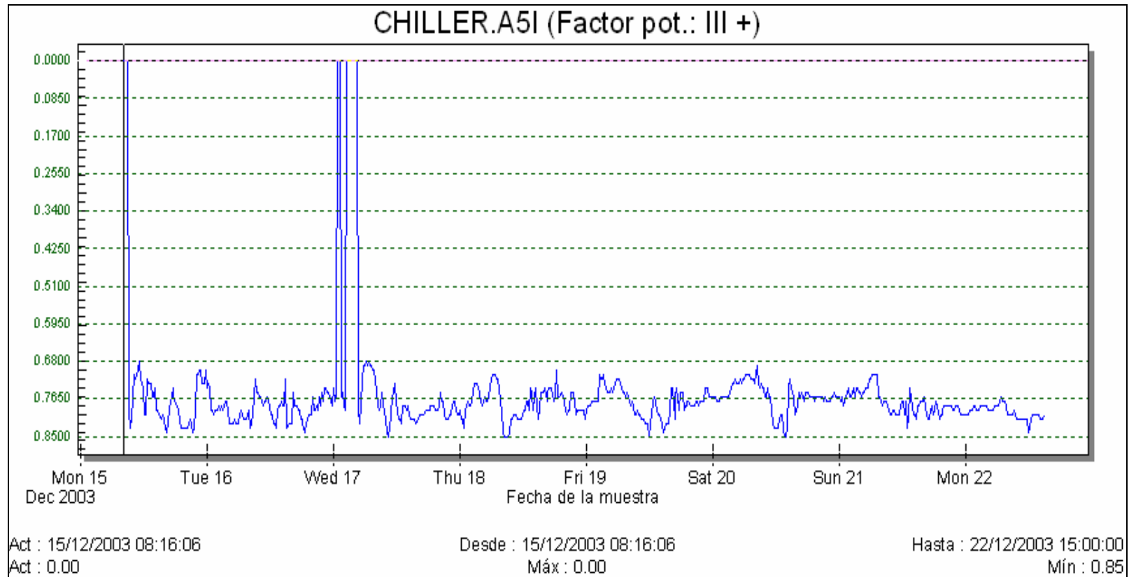
Figura 3.15 Variaciones del factor de potencia de Chiller
