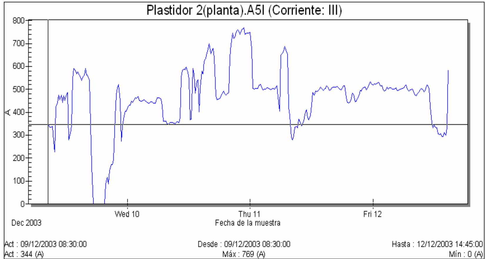
Figura 3.6 Variaciones de la corriente trifásica de Planta
