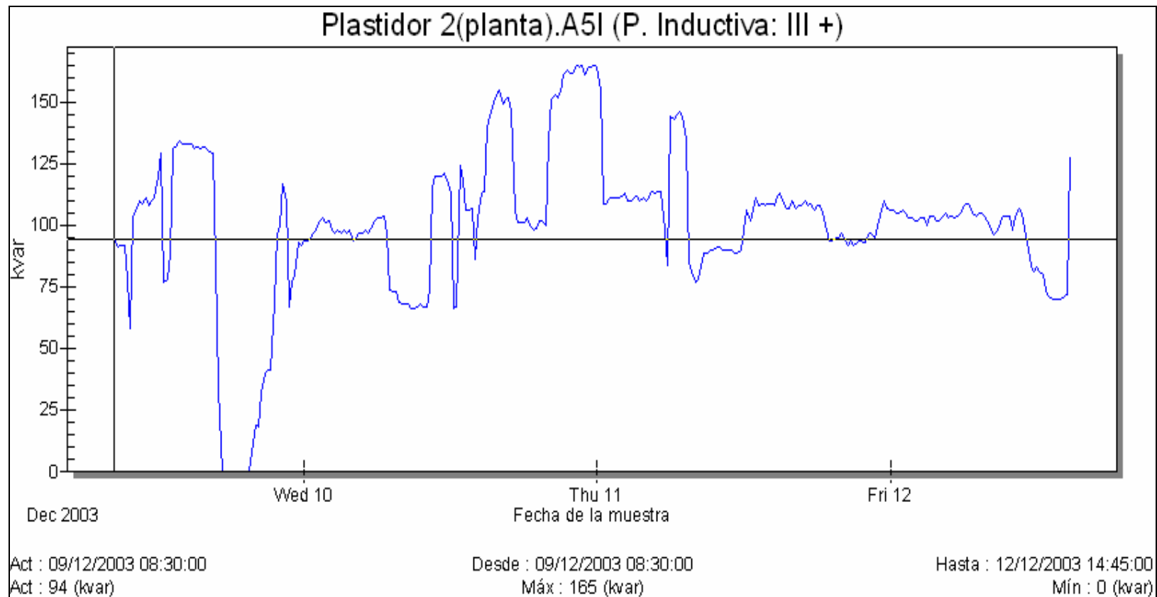
Figura 3.8 Variaciones de la potencia inductiva de Planta
