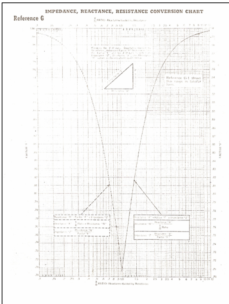
Figura F.1 Referencia G: Relación de Impedancia, Reactancia y Resistencia
