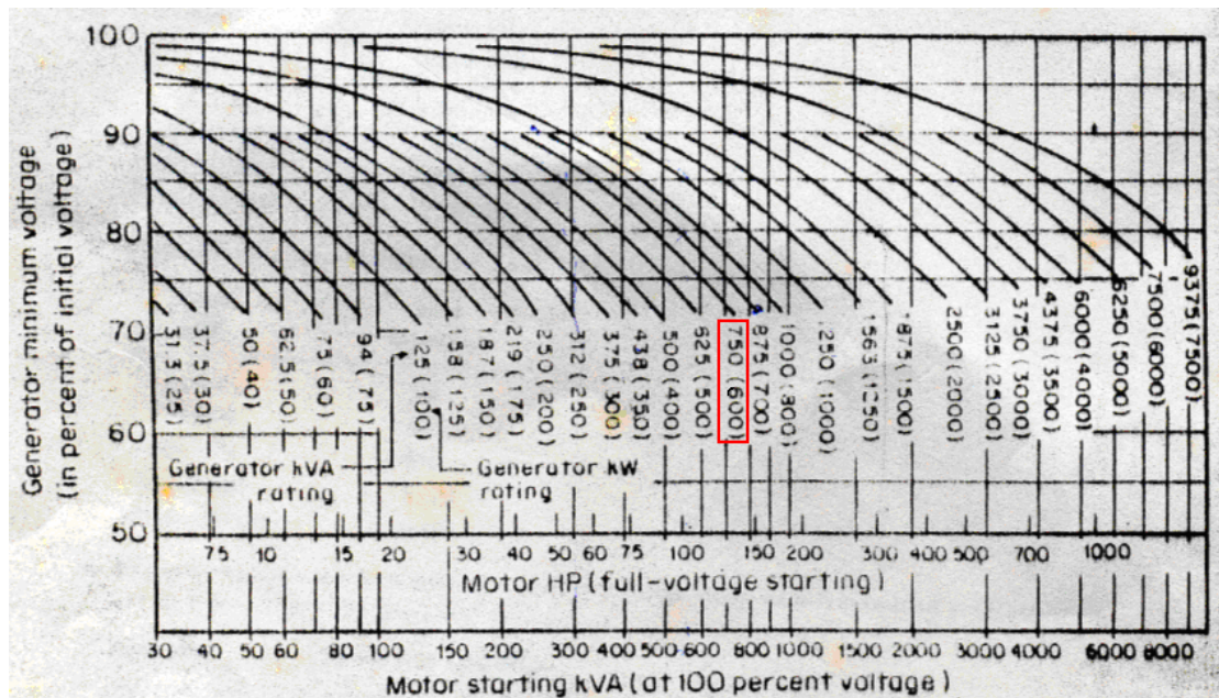
Figura 7.5 Curvas de selección de Generadores
