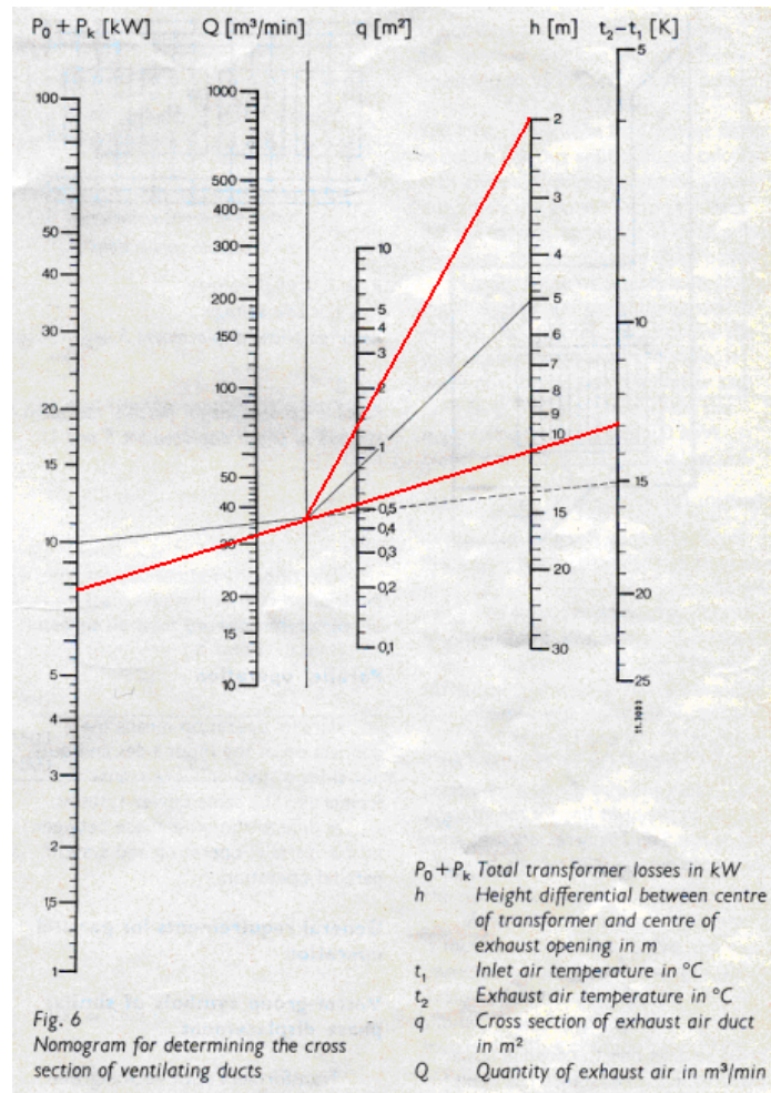
Figura 7.2 Diagrama para determinar el área de los ductos de ventilación
