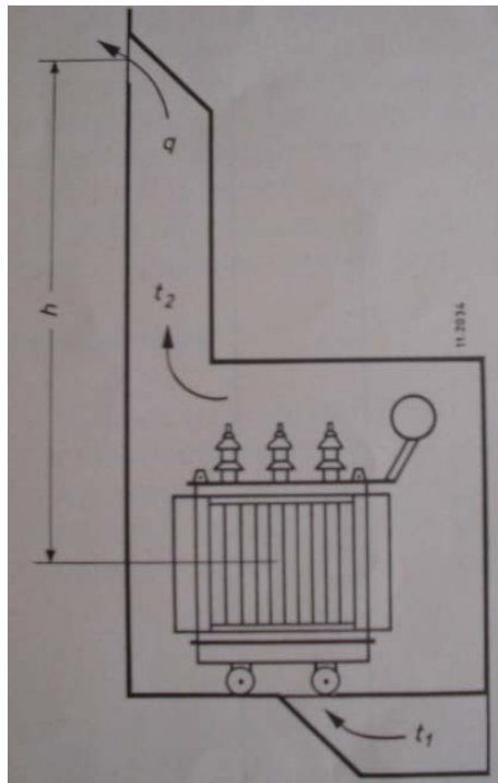
Figura 7.1 Constantes y variables requeridas en el cálculo de ductos
