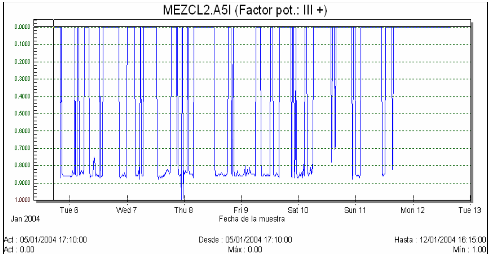
Figura 3.21 Variaciones del factor de potencia de Mezclado
