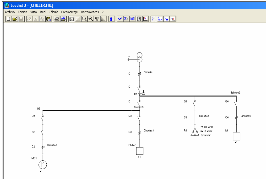
Figura 4.2 Esquema eléctrico
