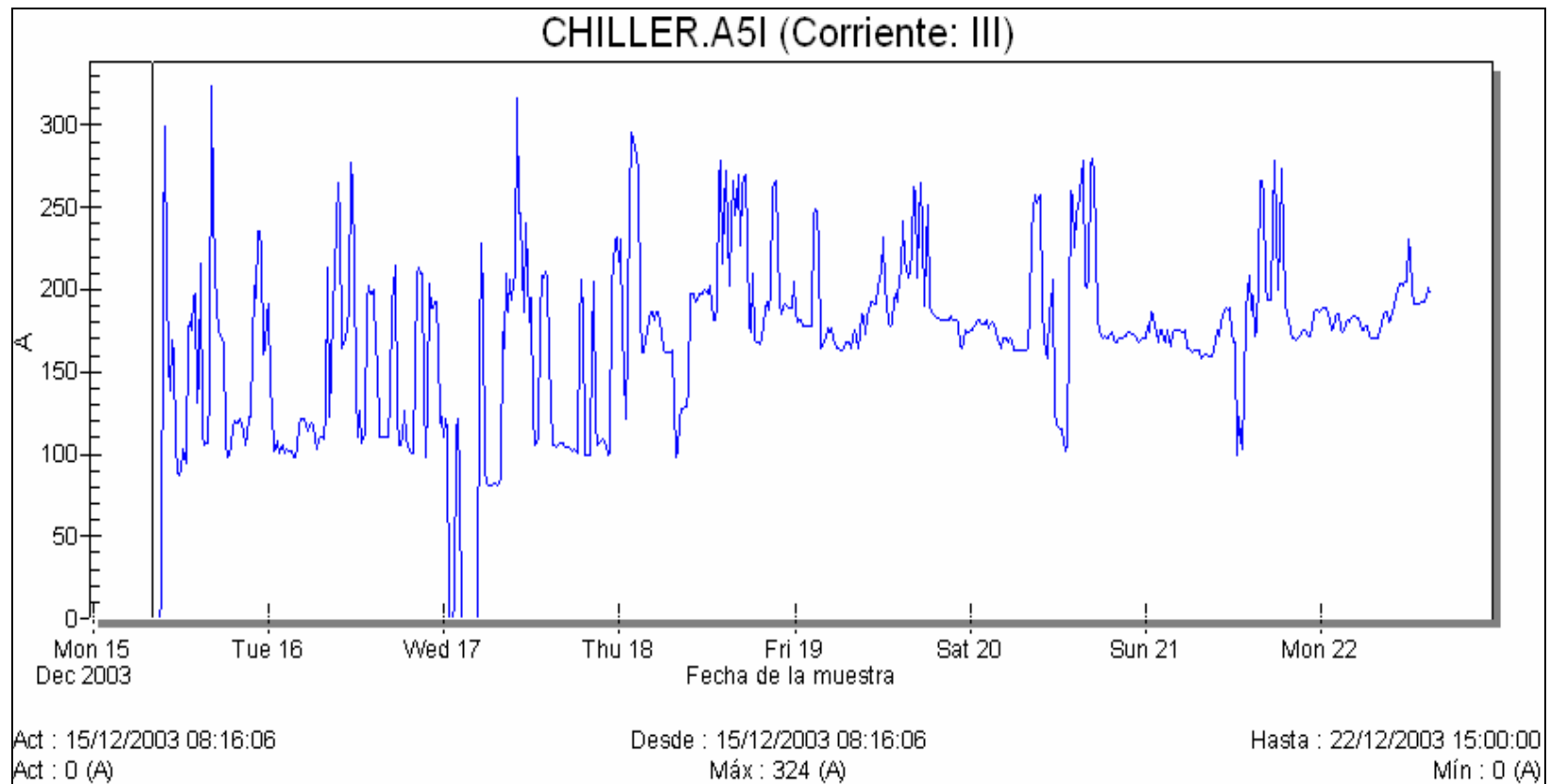
Figura 3.12 Variaciones de la corriente trifásica de Chiller
