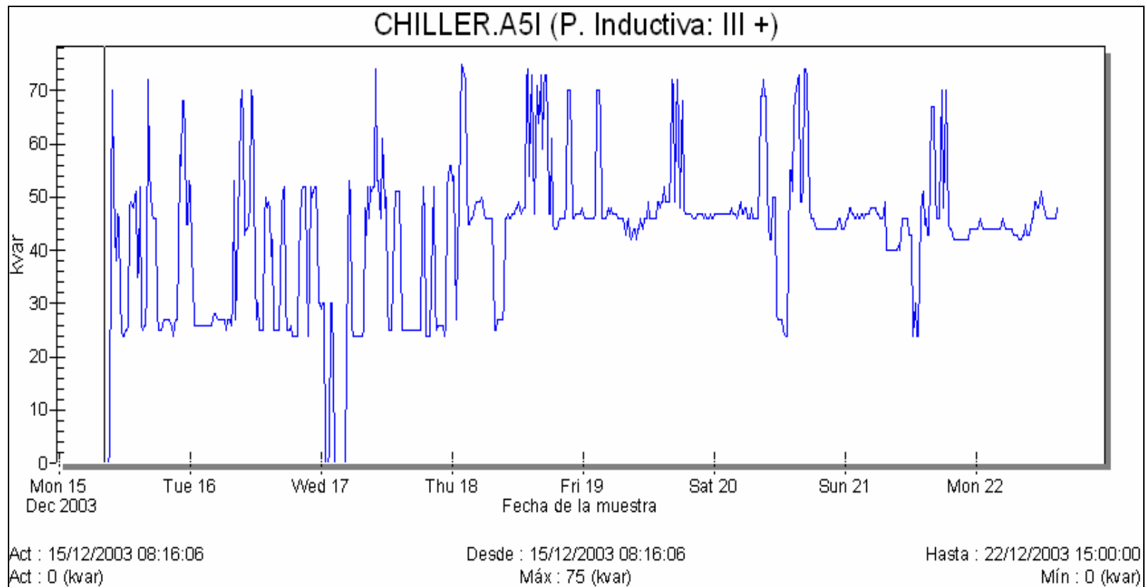
Figura 3.14 Variaciones de la potencia inductiva de Chiller
