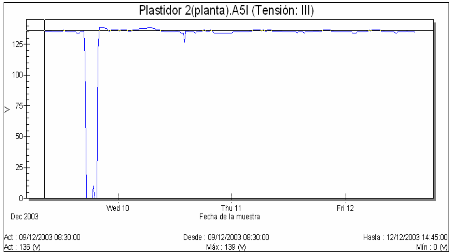
Figura 3.5 Variaciones del voltaje trifásico de Planta
