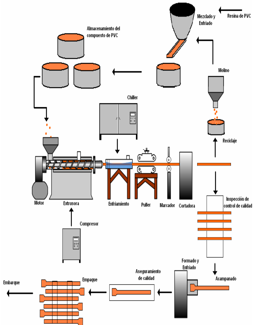
FIGURA 2.1 Proceso de Fabricación de tuberías PVC
