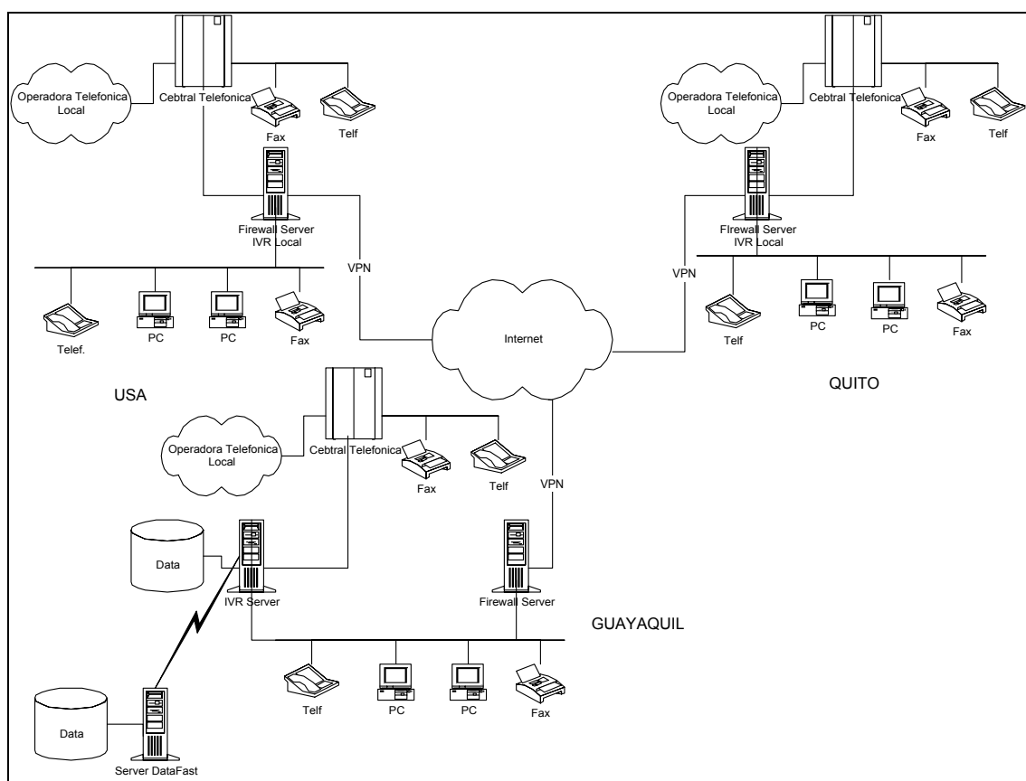
Figura 17. Diagrama de red a implementar para la institución ABC
