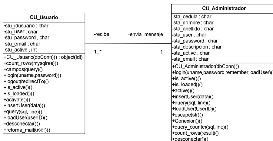
Figura A.4.- Diagrama de clases
