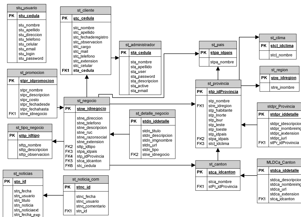
Figura A.3.- Modelo Lógico
