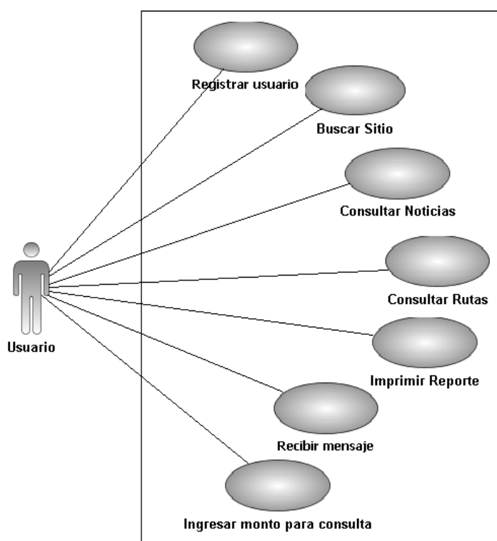
Figura A.1. Diagrama de Casos de Uso
