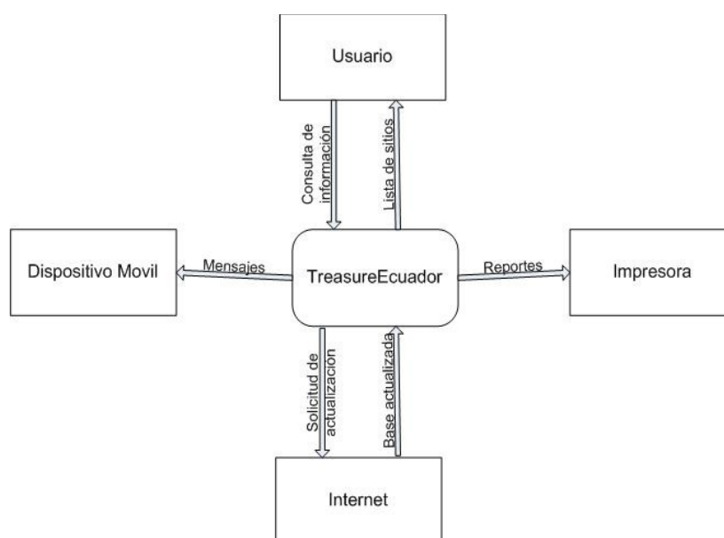
Figura A.2. Diagrama arquitectónico de TreasureEcuador
