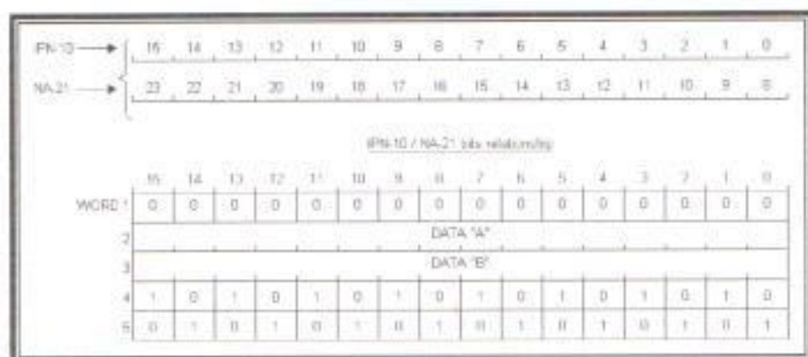
Figura No. 2-25 Buffer de Prueba del IPN-10 a la NA-21 cuando la NA-21 está inactiva
