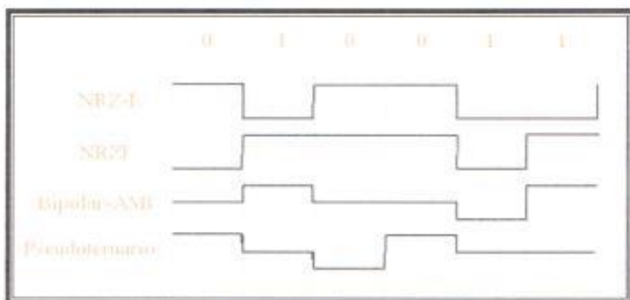
Figura No. 1-3 Codificación NRZ y Binario Multinivel
