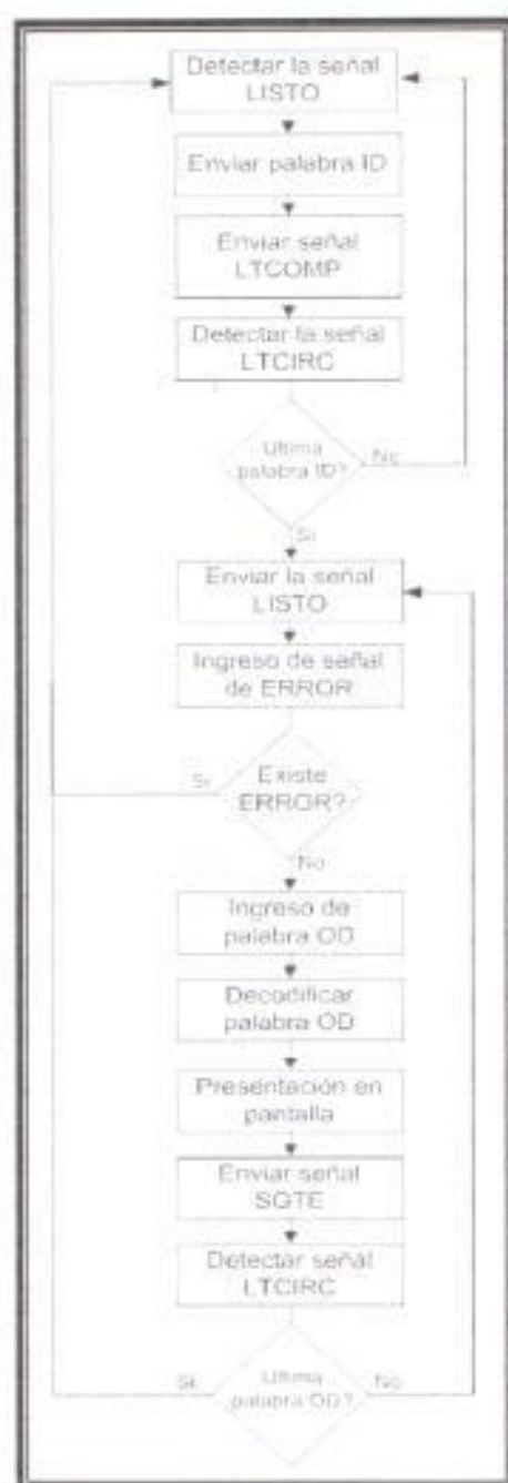
Figura No. 3-14 Diagrama de Flujo de la Subrutina ADQdatos
