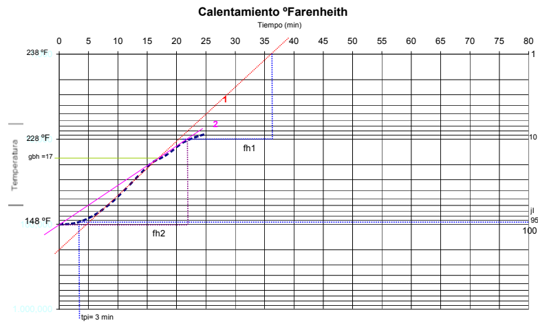
FIGURA 2.4 GRÁFICO DE DATOS DEL CALENTAMIENTO
