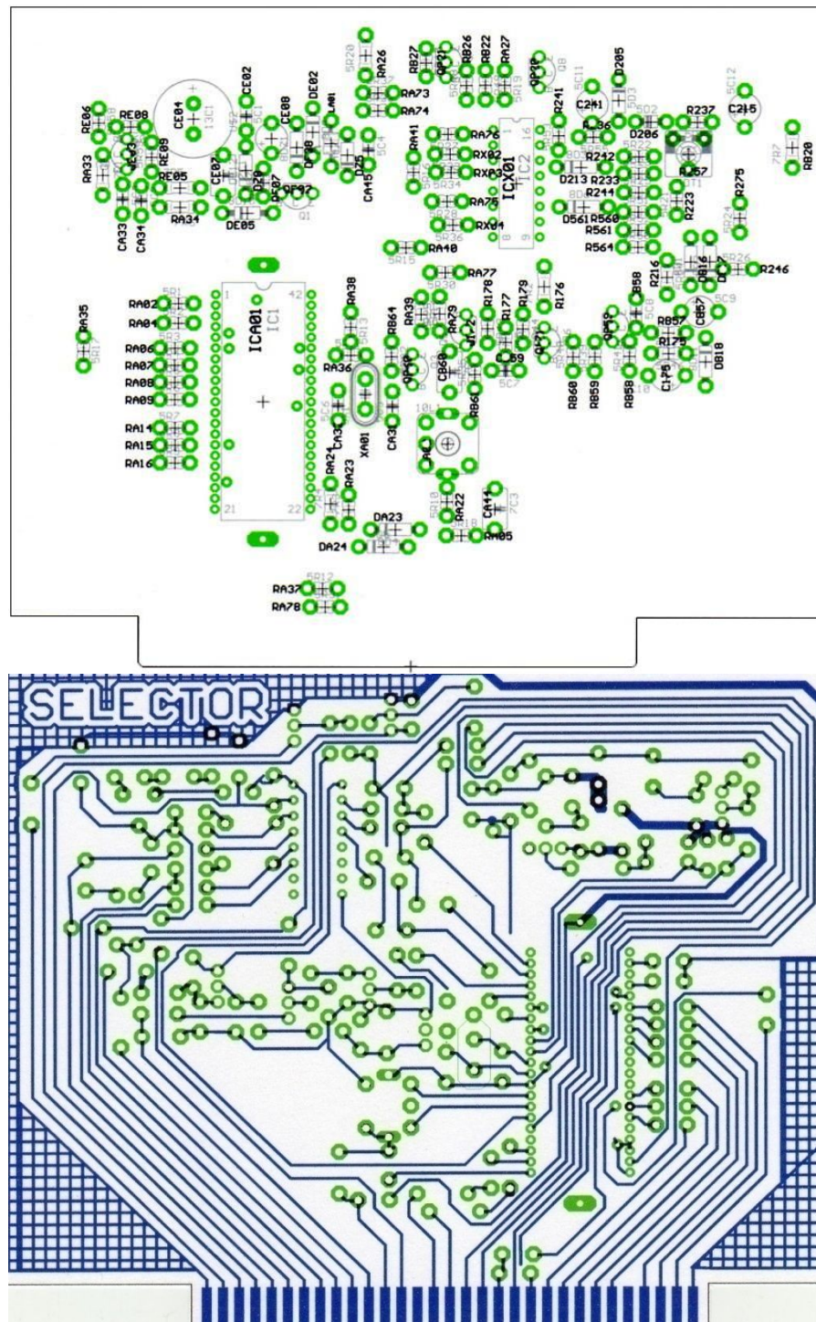
Figura 2.3.3 Sección SELECTOR trazado superior e inferior
