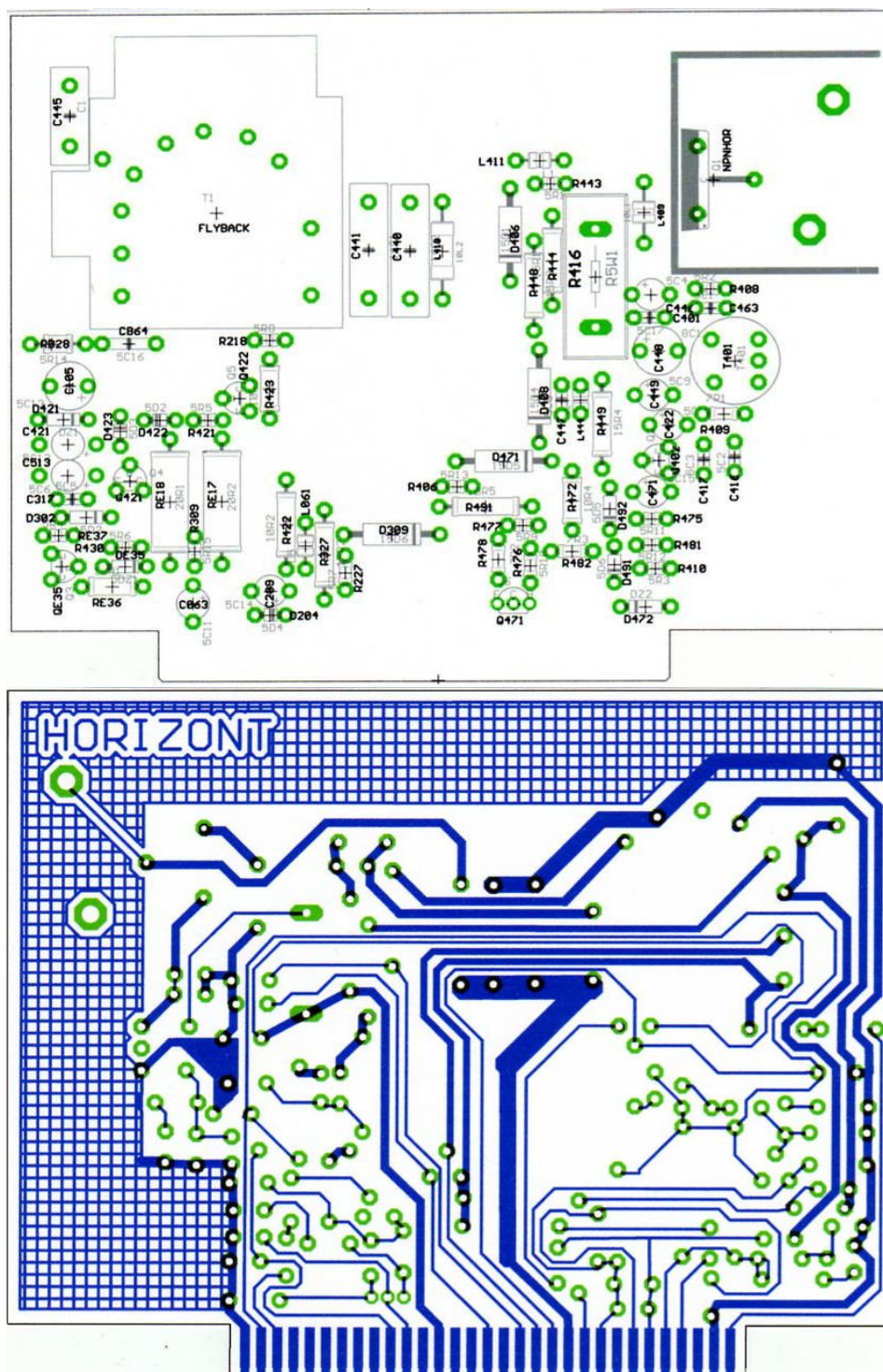
Figura 2.3.5 Sección HORIZONTAL trazado superior e inferior
