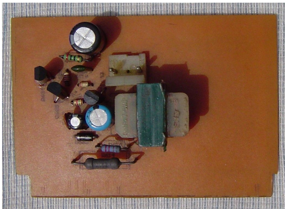
Figura A.7 Sección Sonido
