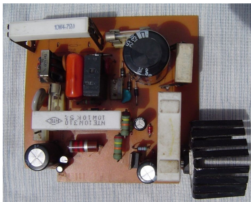
Figura A.2 Sección Fuente
