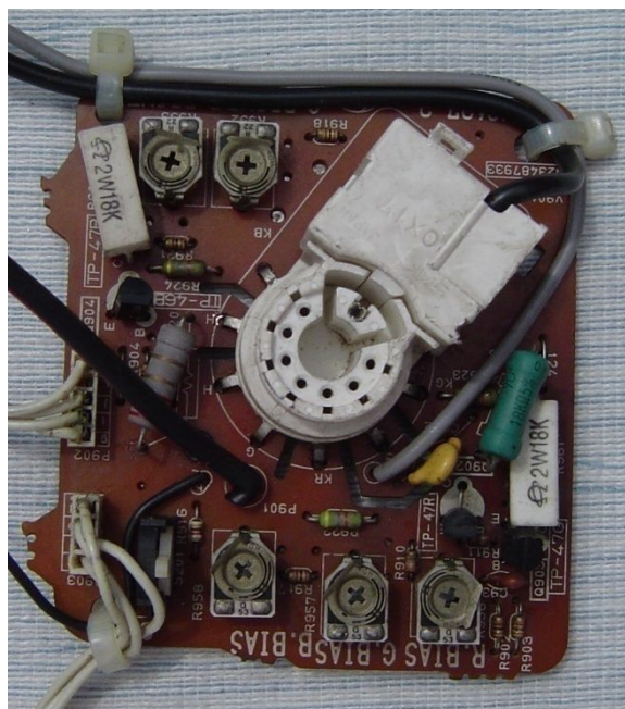
Figura A.8 Sección Socket
