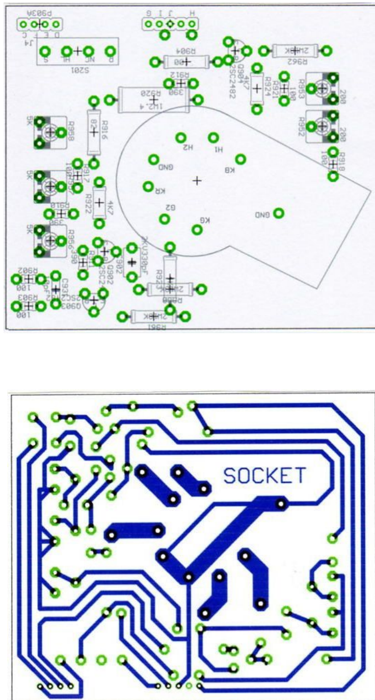
Figura 2.3.8 Sección SOCKET trazado superior e inferior
