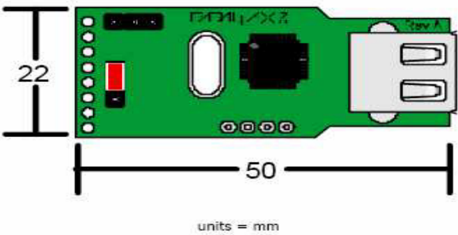
FIGURA 2-5: Dimensiones del Datalogger
