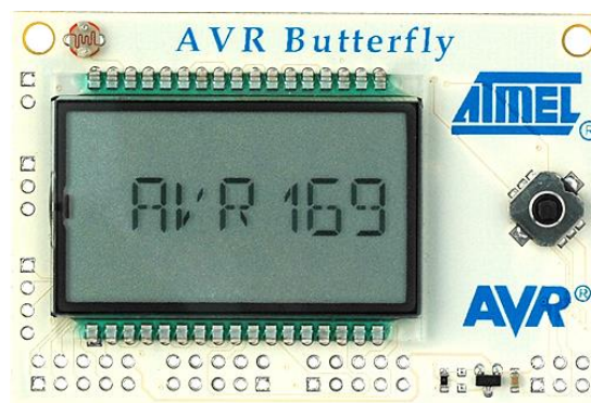
FIG. 2.7 AVR BUTTERFLY
