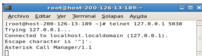
Fig 4.1 Conexión al puerto 5038 a través de telnet.
