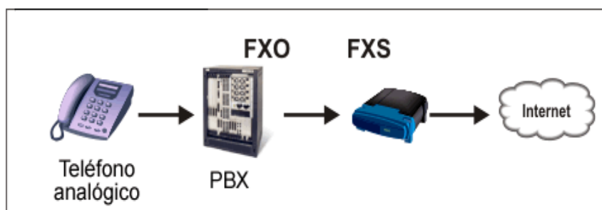
Fig. 2.3 Conexión FXS a una central PBX.
