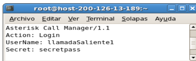
Fig 4.2 Envío de paquete para realizar conexión a AMI.
