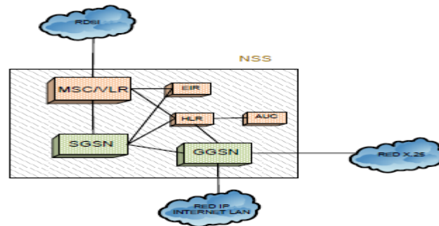
Ilustración 22 Elementos de la red NSS
