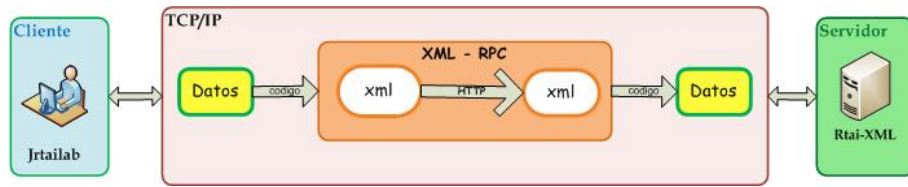
Figura 4.4. Comunicación XML-RPC
