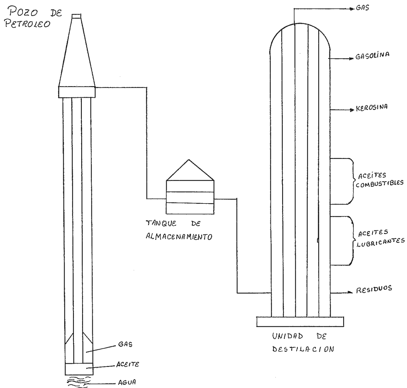
Fig. 4.- Aceite: Refinación y elaboración
