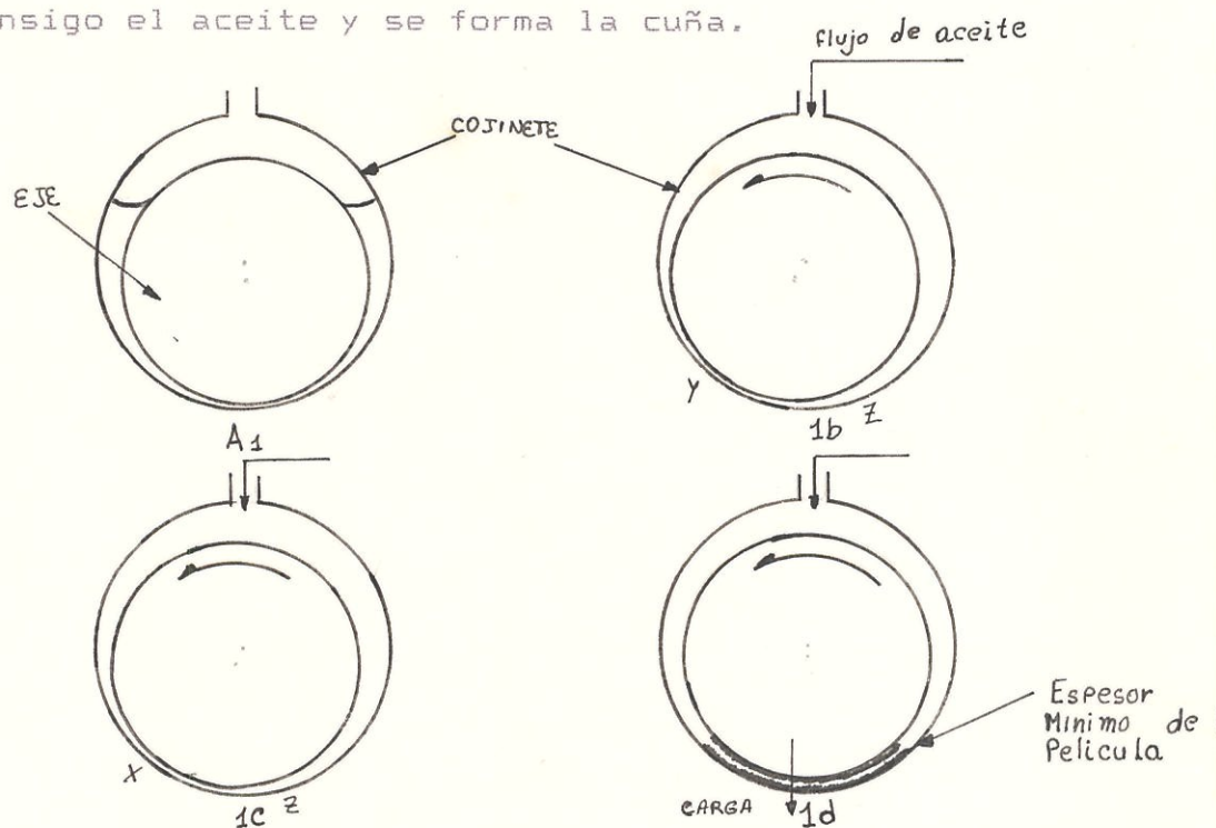
Fig. 3.- Acción hidrodinámica y formación de la película de aceite.
