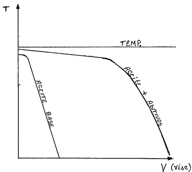
Fig. # 8.- Índice de viscosidad
