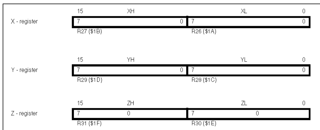
Figura 2.10 AVR-CPU Registros X, Y y Z.
