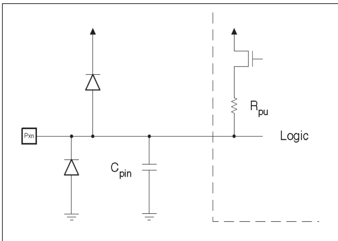
Figura 2.19 Diagrama Equivalente de un pin de E/S
