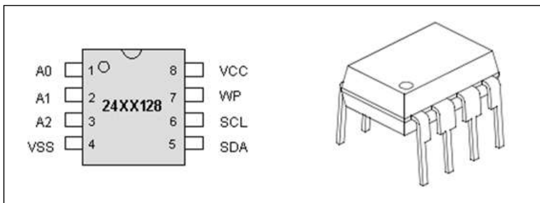
Figura 3.4 Esquema físico de EEPROM serial de la familia 24XX128
