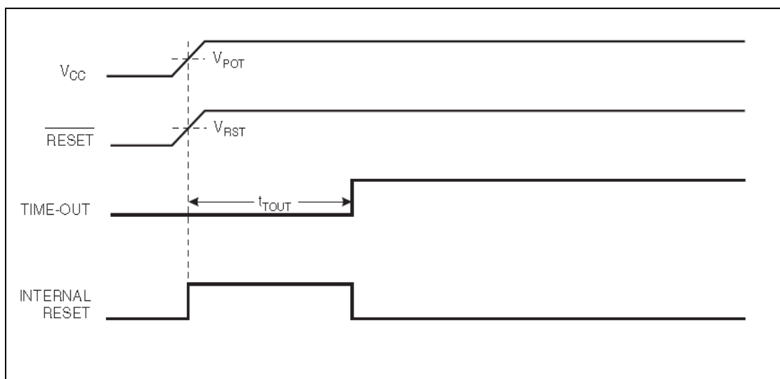
Figura 2.14 Inicio del MCU el reset tiende al nivel de Vcc
