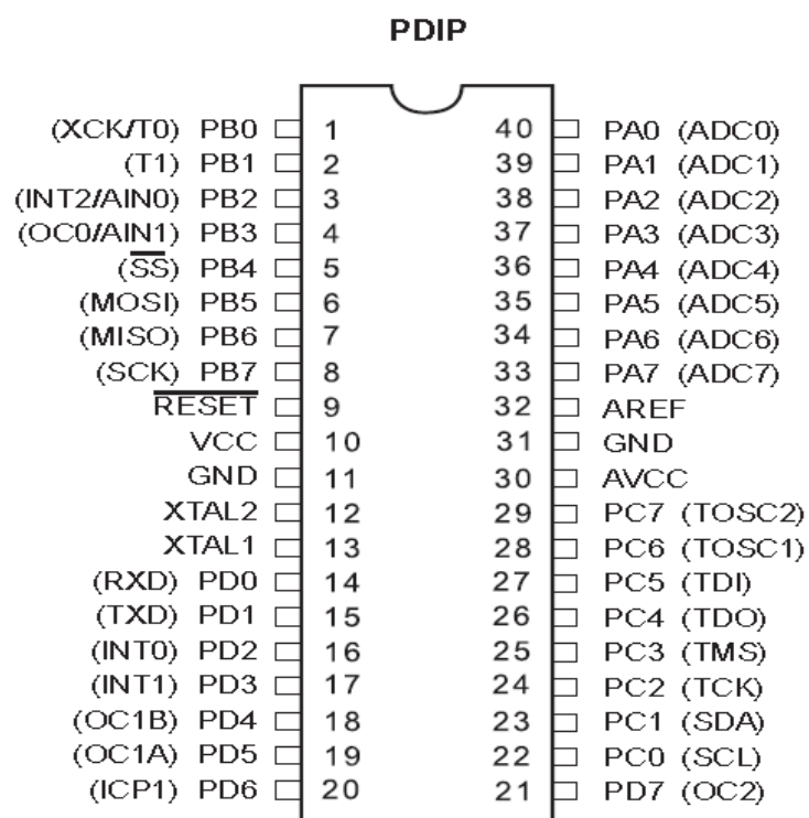
Figura 2.6 Pines correspondientes al MCU ATmega32
