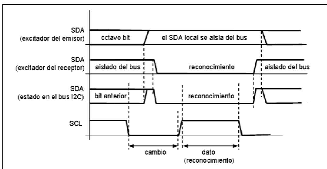
Figura 1.7 Proceso de reconocimiento en el bus I2C
