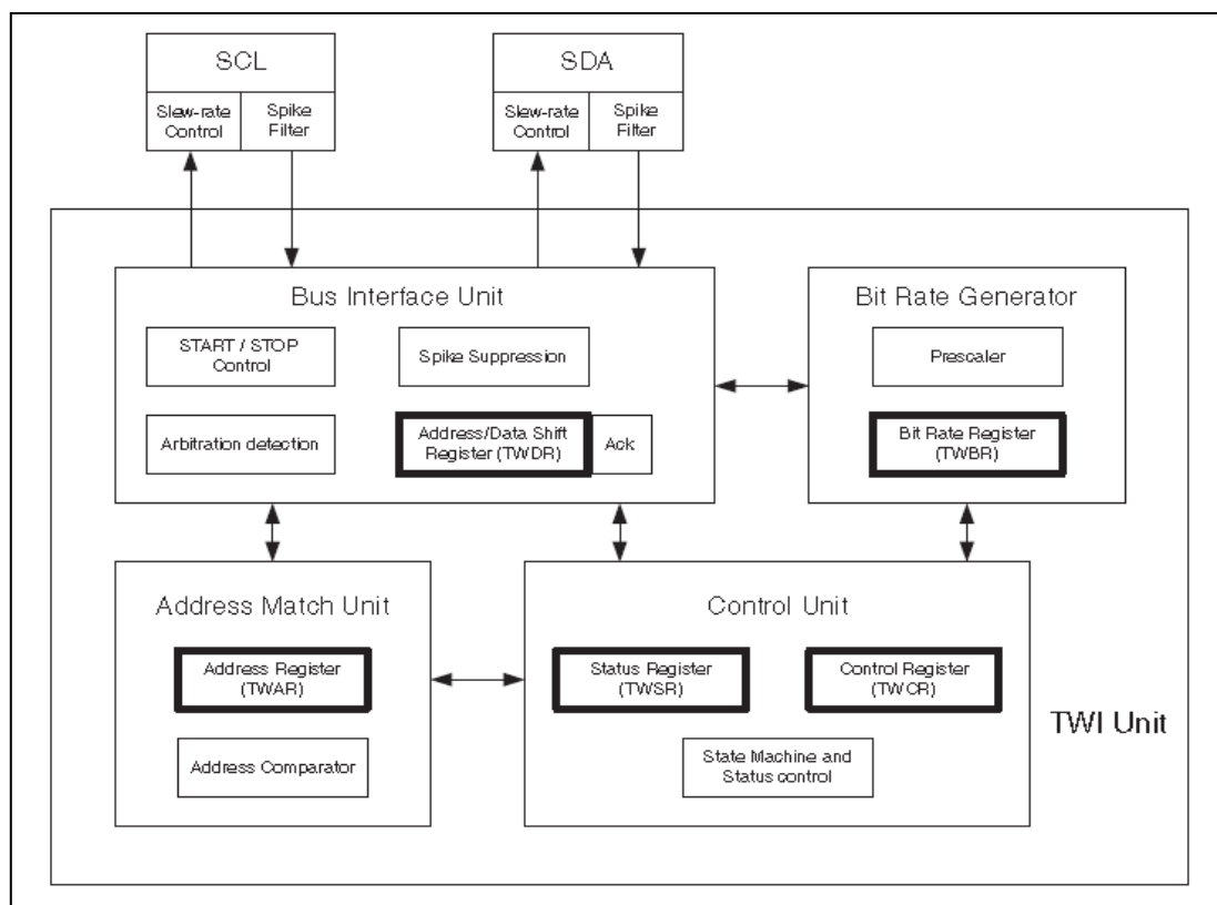
Figura 2.21 Descripción General del módulo TWI
