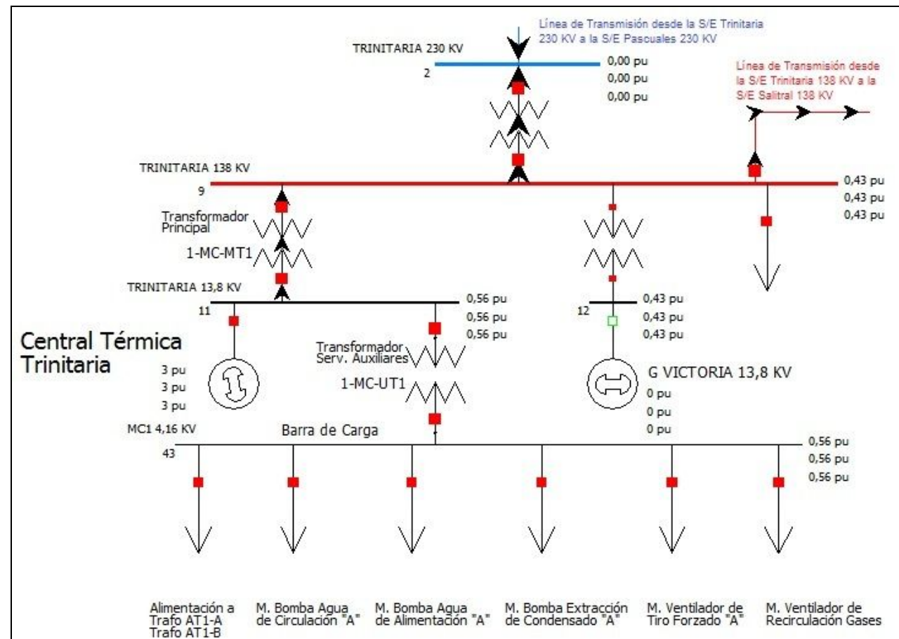
3.1 Falla trifásica en la Barra #2, Trinitaria 230 KV.
