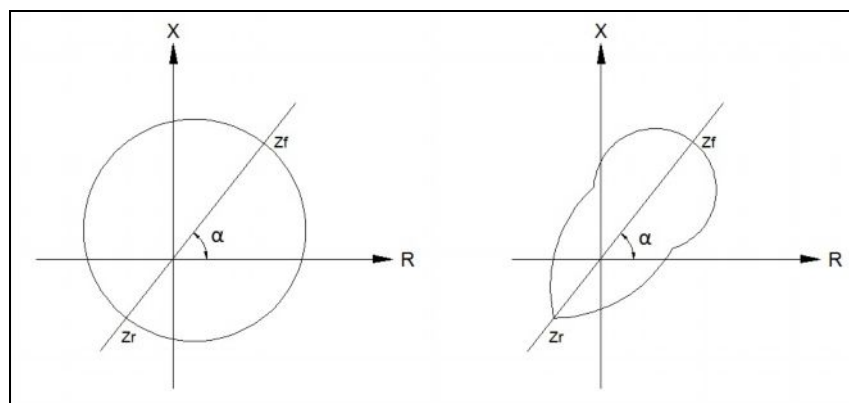
Figura 4.12 - Característica circular MHO desplazada o lenta modificada con 60^\circ ó 75^\circ .
