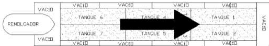
Ilustración 12. Esquema de llegada a puerto de barcaza articulada. (Fuente: Víctor Suárez Holguín).
