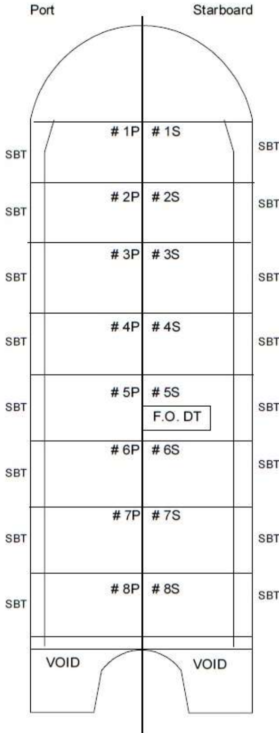
Ilustración 20. Esquema de distribución de tanques de barcazas articuladas. (Fuente: http://www.bouchardtransport.com/barges.php ).
